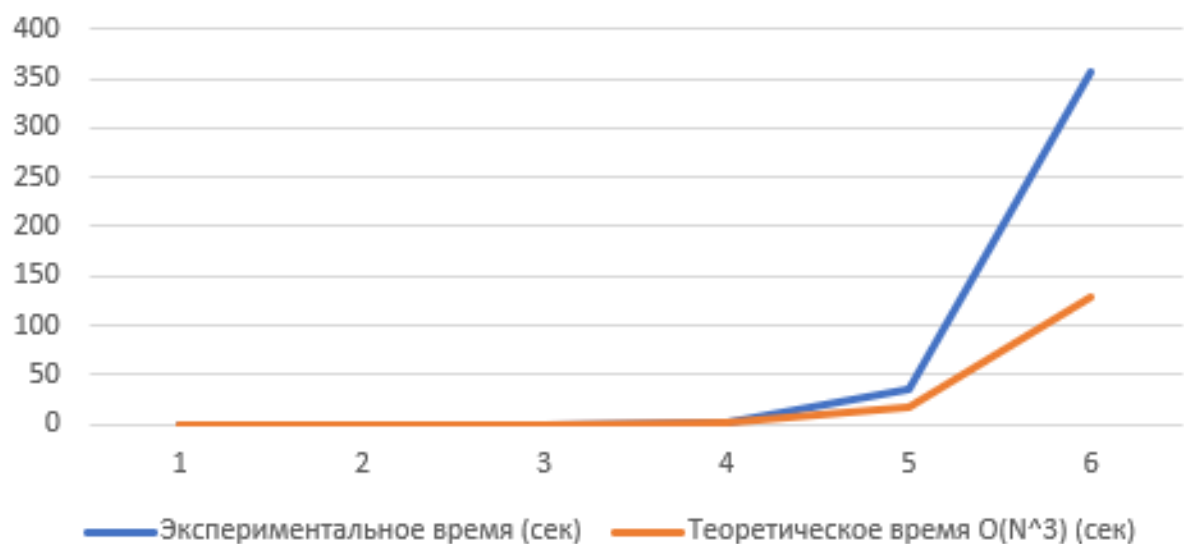
график зависимости времени выполнения программы
