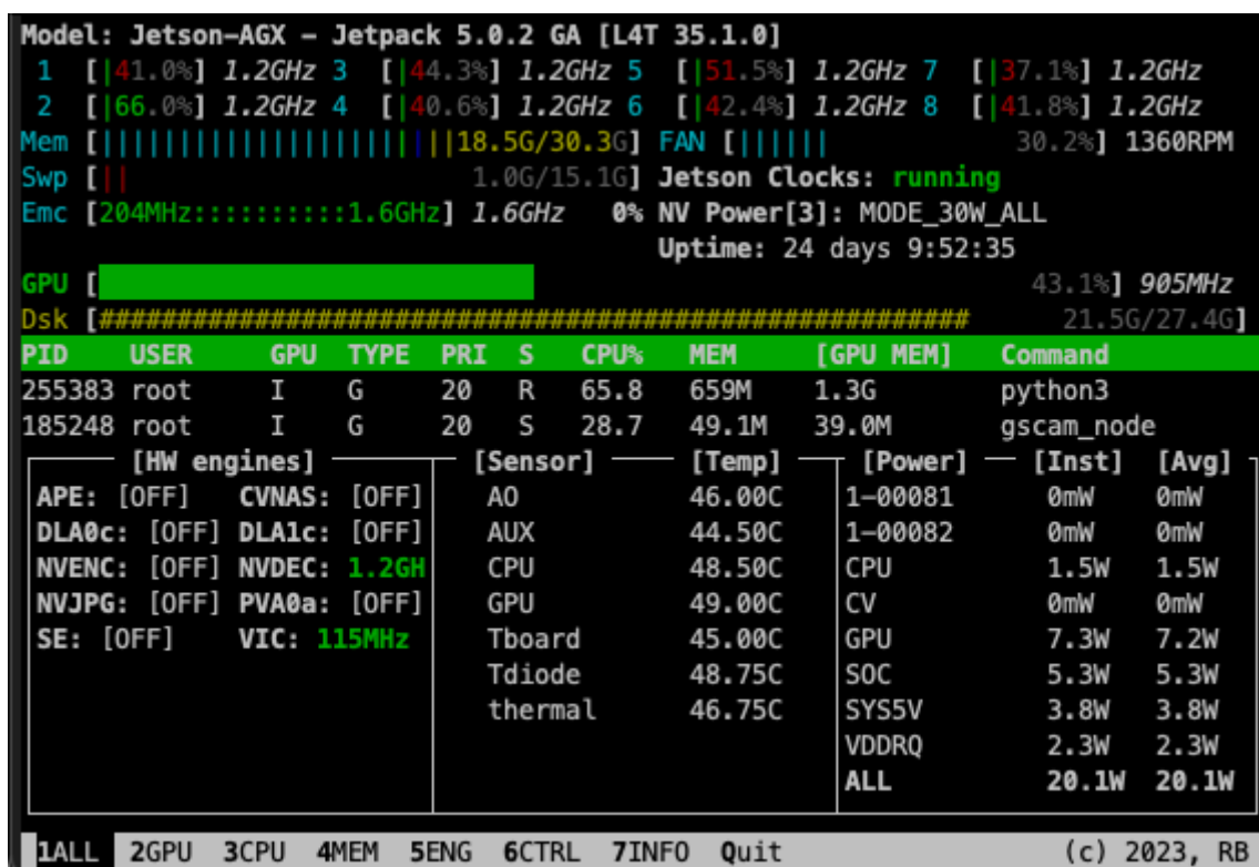
Joonis 5.3.1. YOLOv5l, ühe sisendiga, resolutsioonil 640x640 pikslit, optimeerimata mudeli jooksmine ei utiliseeri kogu graafikakaarti, monitooringurakenduses jtop [62]
