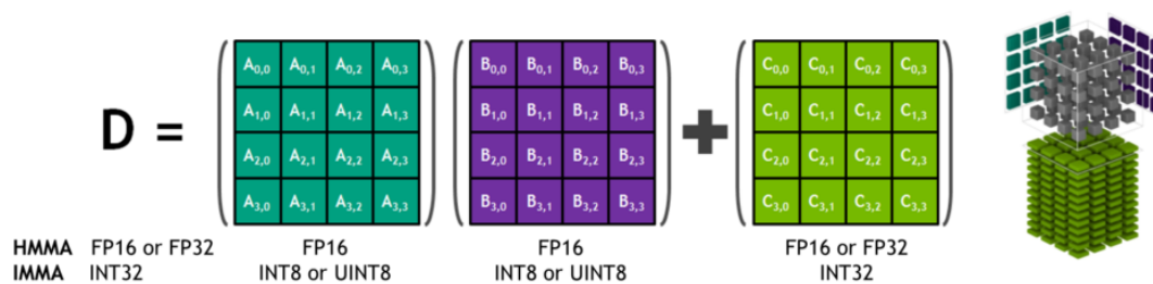
Joonis 3.2.1. Tensor Core, kolmedimensiooniliste 4x4x4 maatriksite korrutamine ning summeerimine [27]
