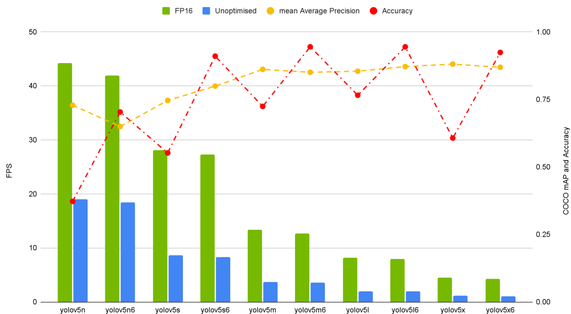
Joonis 6.2.2. Mudelite jõudlus 1 kaadri sisendiga, suurusel 1280x1280 pikslit
