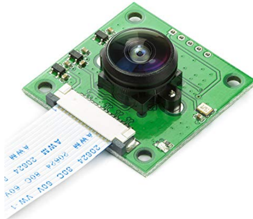
Joonis 3.3.1. Arducam Fisheye kaameraga moodul [34]
