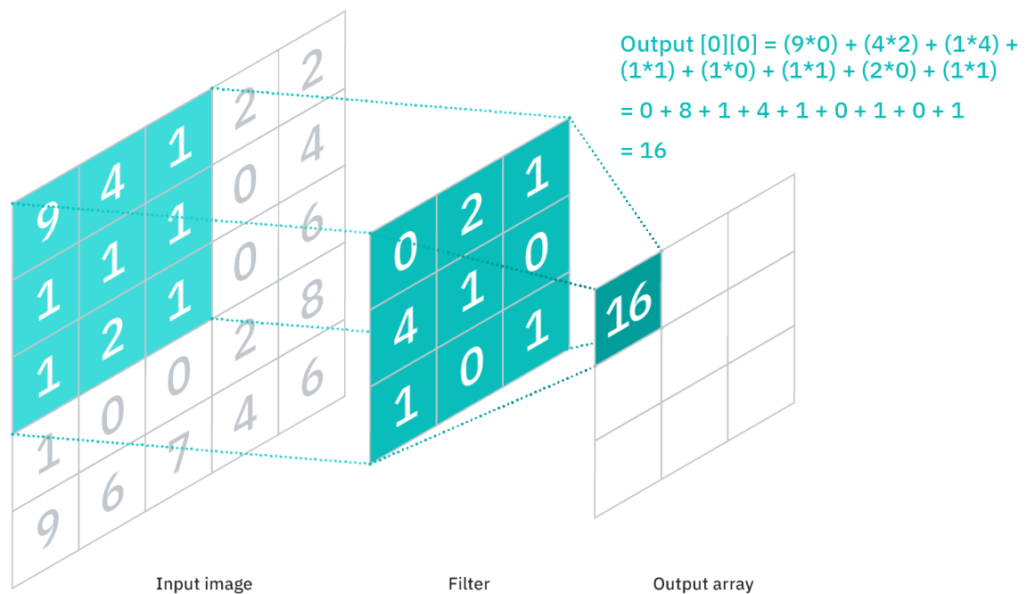
Joonis 3.1. Maatrikskujul pildil (vasakul) tehakse operatsioon filtriga (keskel), mis annab tulemuseks skalaarkorrutise tunnuste kaardina (paremal)
