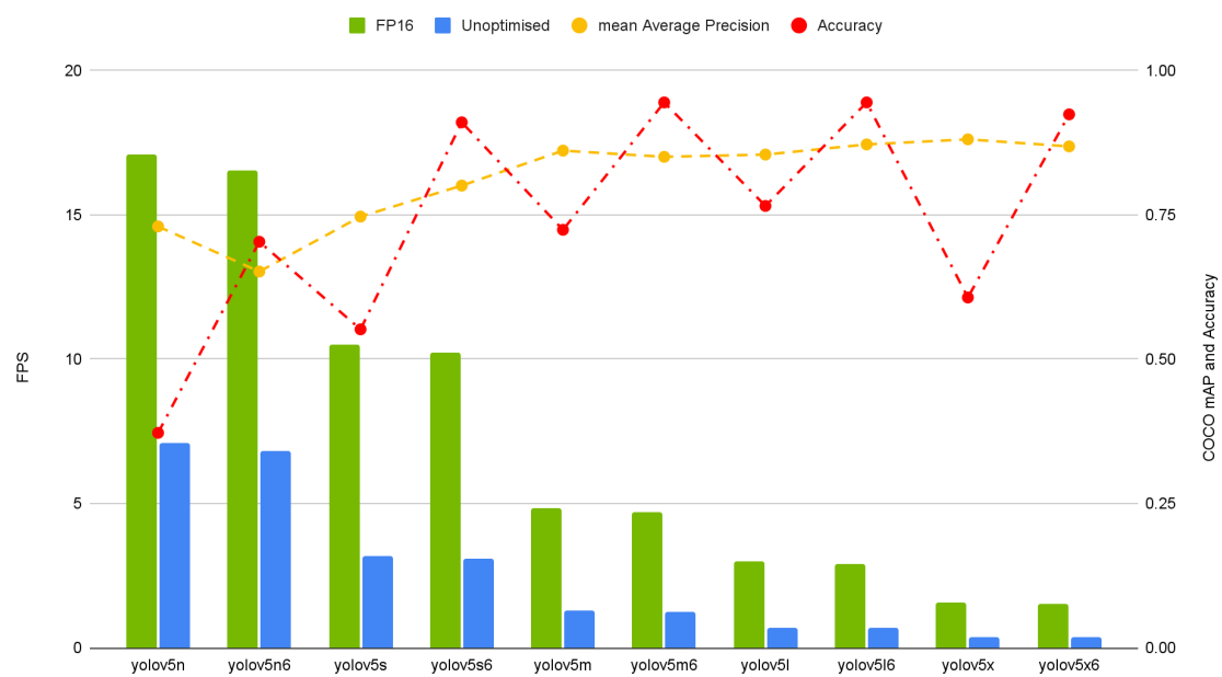
Joonis 7.4. Mudelite jõudlus 3 kaadri sisendiga paralleelselt, suurusel 1280x1280 pikslit
