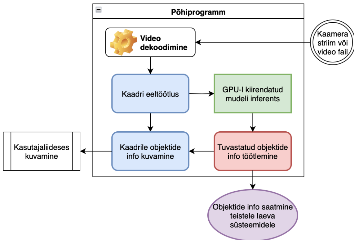
Joonis 6.4. Põhiprogrammi lihtsustatud plokkskeem
