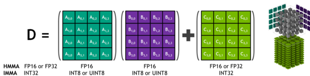
Joonis 4.2. Tensor Core, kolmedimensiooniliste 4x4x4 maatriksite korrutamine ning summeerimine [27]
