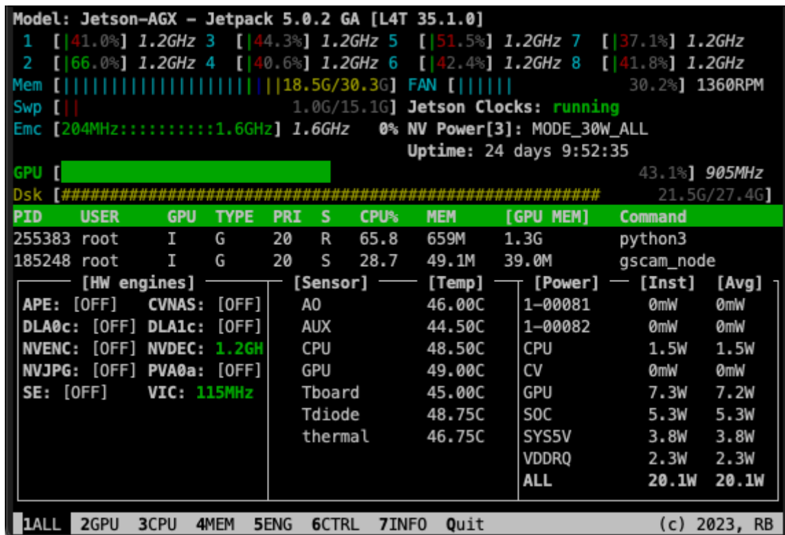
Joonis 6.9. YOLOv5l, ühe sisendiga, resolutsioonil 640x640 pikslit, optimeerimata mudeli jooksmine ei utiliseeri kogu graafikakaarti, monitooringurakenduses jtop [62]
