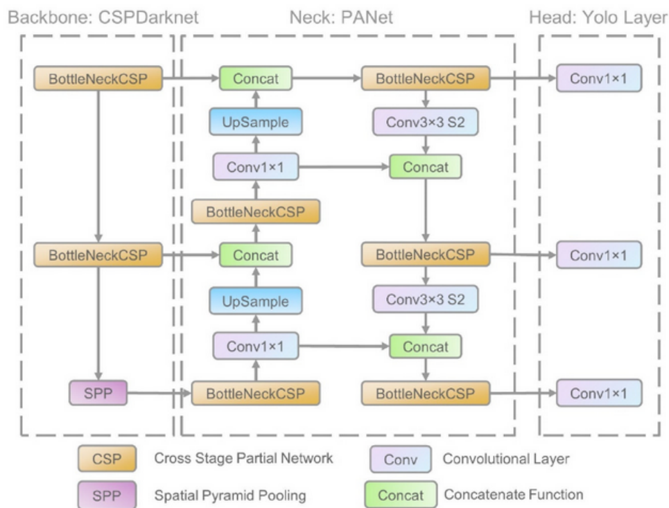
Joonis 5.1. YOLOv5 mudelite arhitektuur [54]
