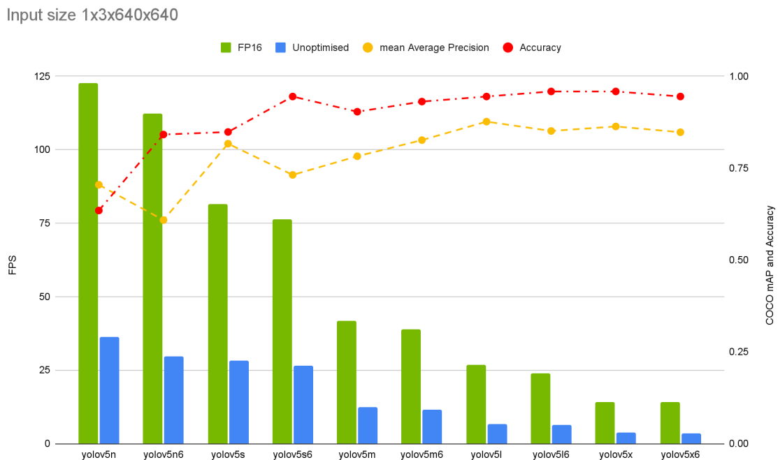
Joonis 7.1. Mudelite jõudlus 1 kaadri sisendiga, suurusel 640x640 pikslit
