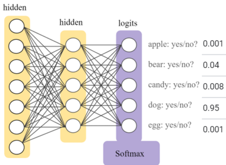
Joonis 3.2. SoftMaxi funktsiooniga rakendatud väljundite kiht närvivõrgus (lilla) ja tõenäosused iga klassi kohta (paremal) [17]
