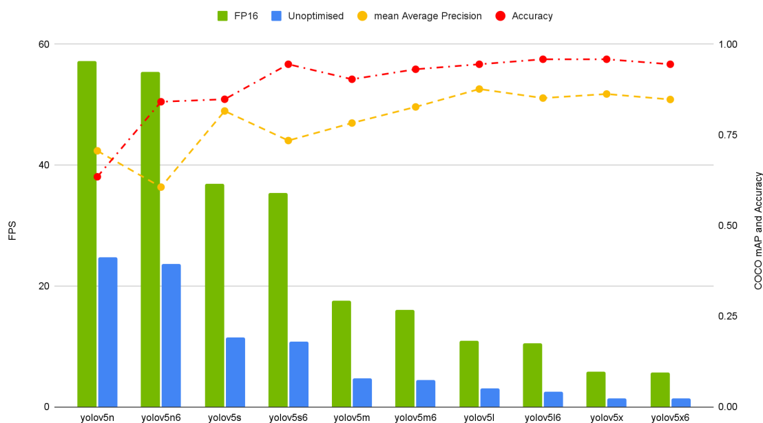
Joonis 7.3. Mudelite jõudlus 3 kaadri sisendiga paralleelselt, suurusel 640x640 pikslit
