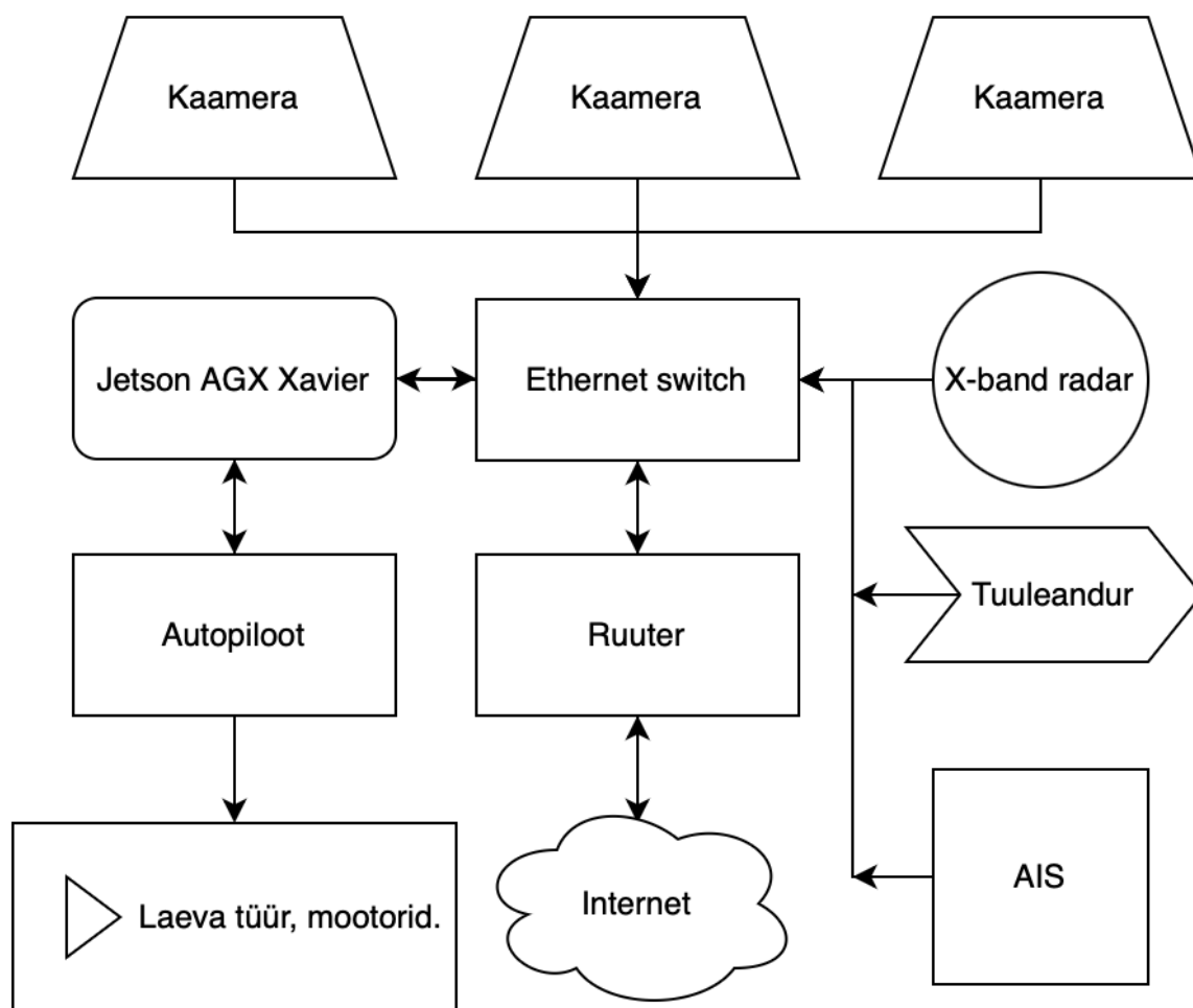
Joonis 4.4. Juhttorni lihtsustatud toimimisskeem
