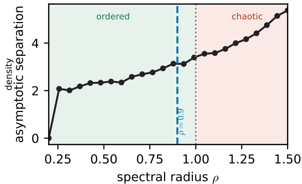
(d) edge of chaos
