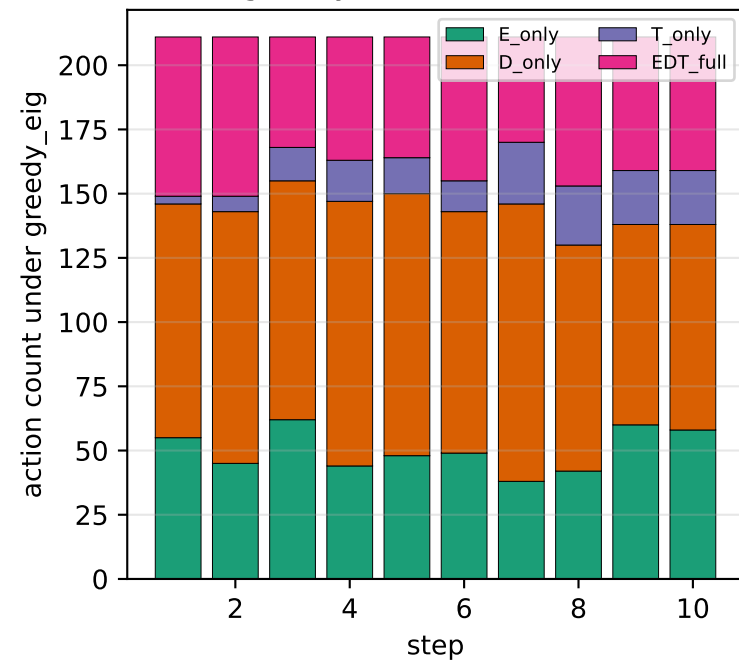
(d) greedy active-selection mix
