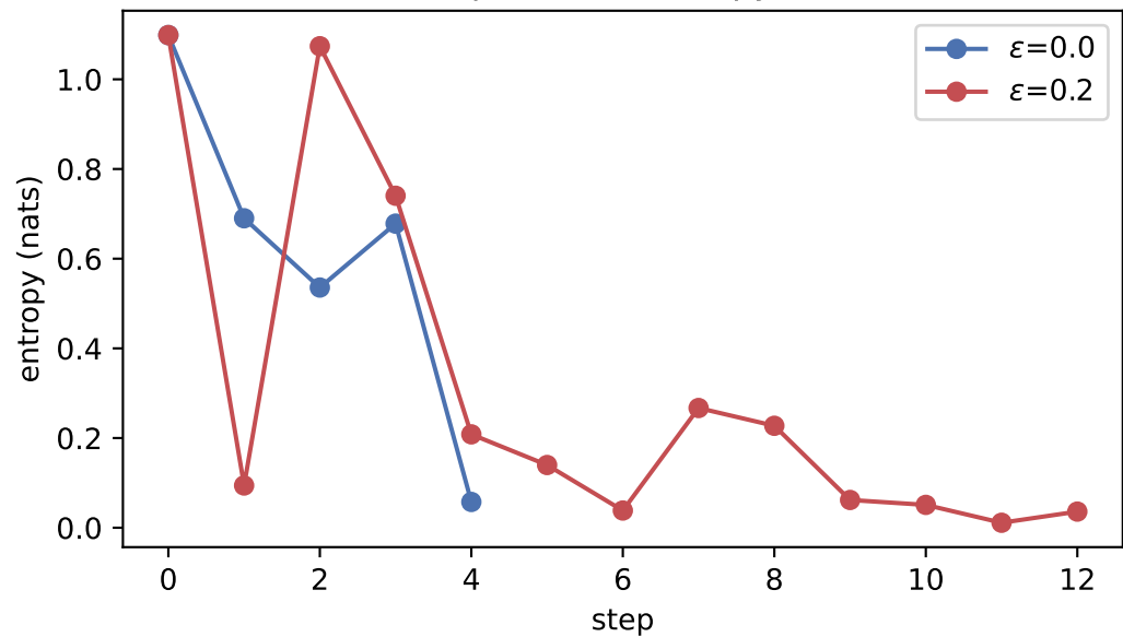
posterior entropy
