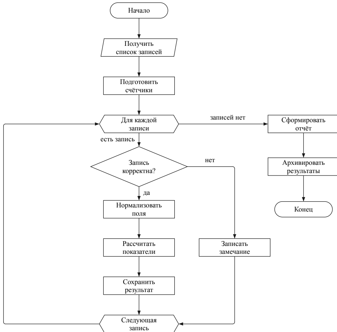
Рисунок 2 – Блок-схема обработки списка с границей цикла
