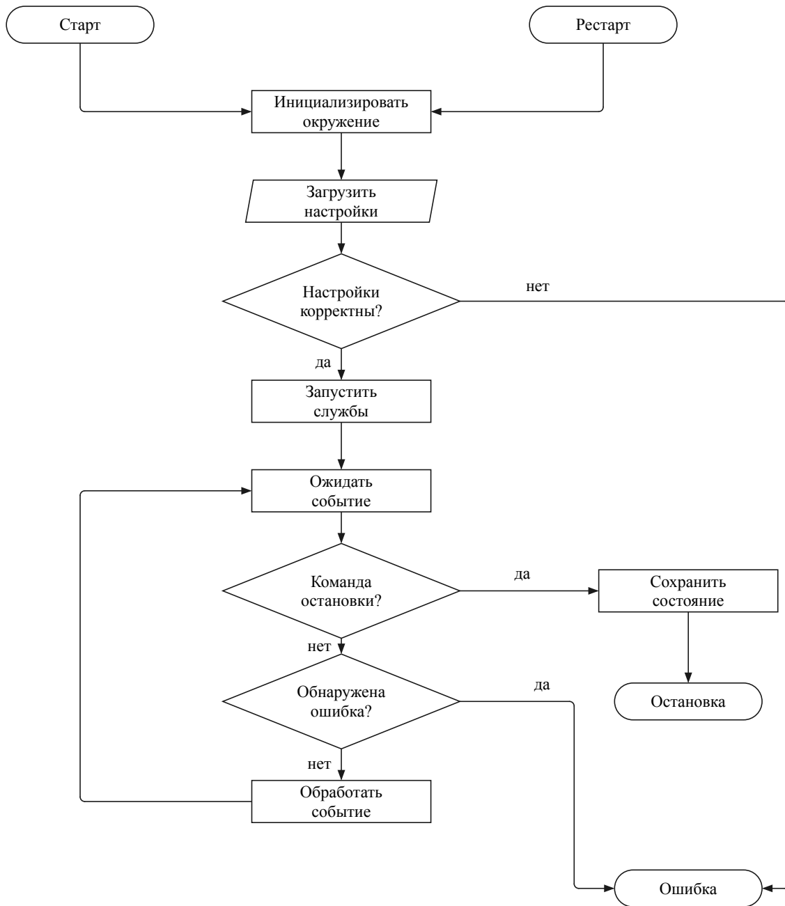
Рисунок 3 – Блок-схема цикла обработки событий программы
