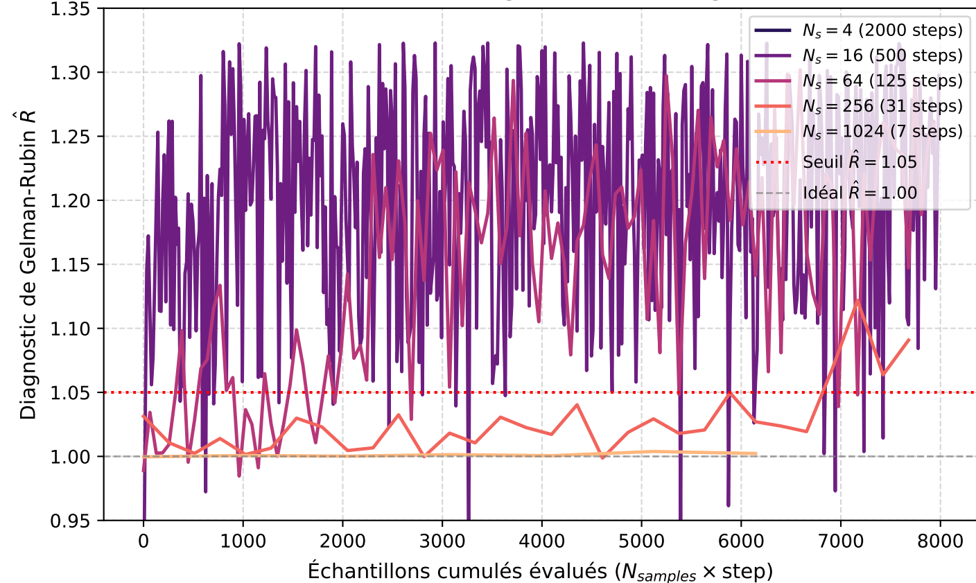
Qualité MCMC : Diagnostic \hat{R} vs Budget Total
