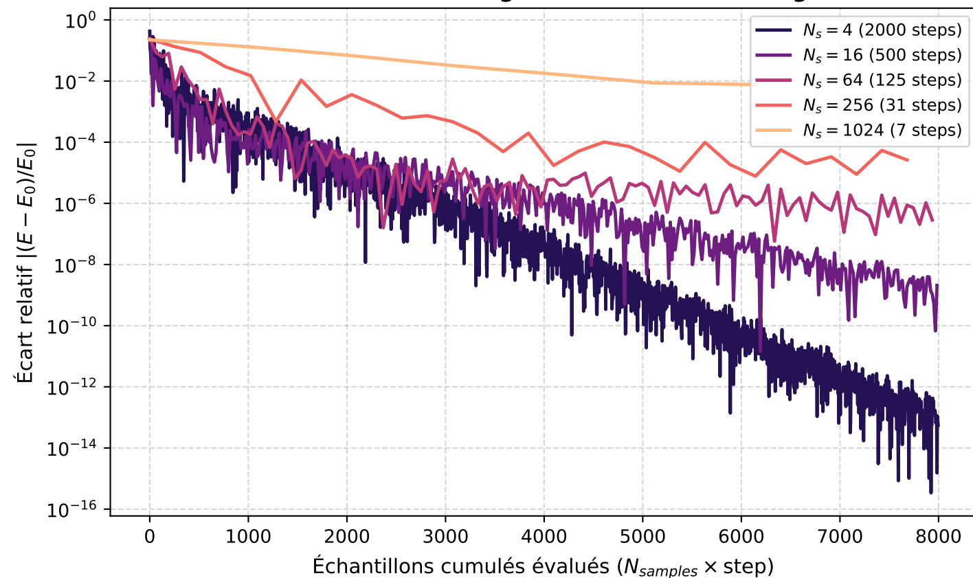
Efficacité d'Échantillonnage : Écart relatif vs Budget Total
