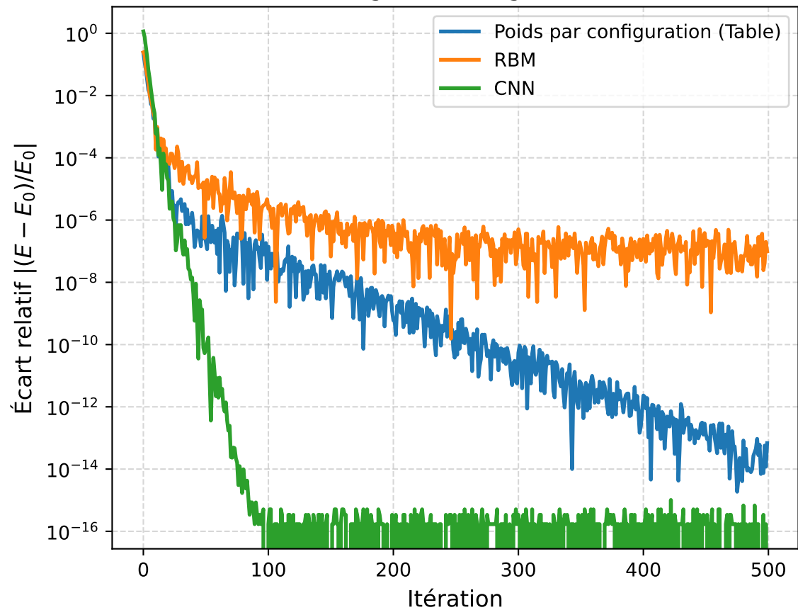
Convergence Énergie (TFIM)
