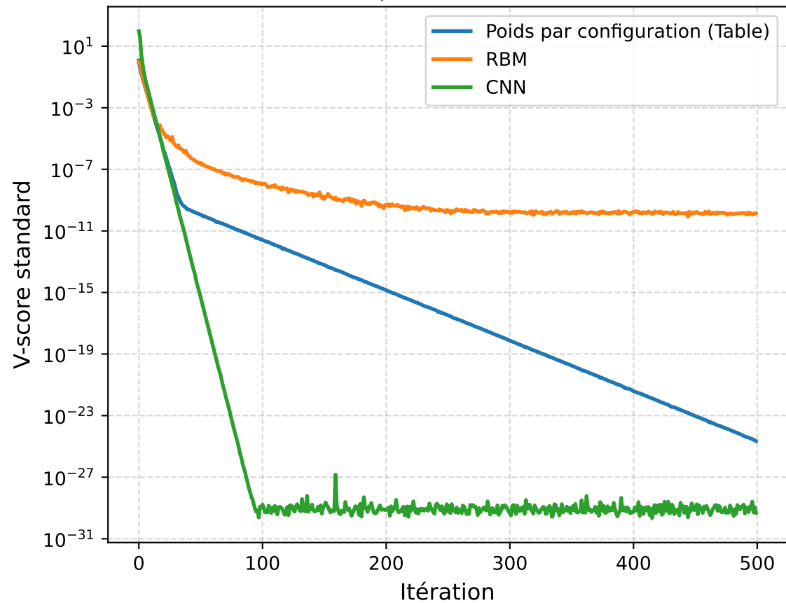
V-score par itération (TFIM)
