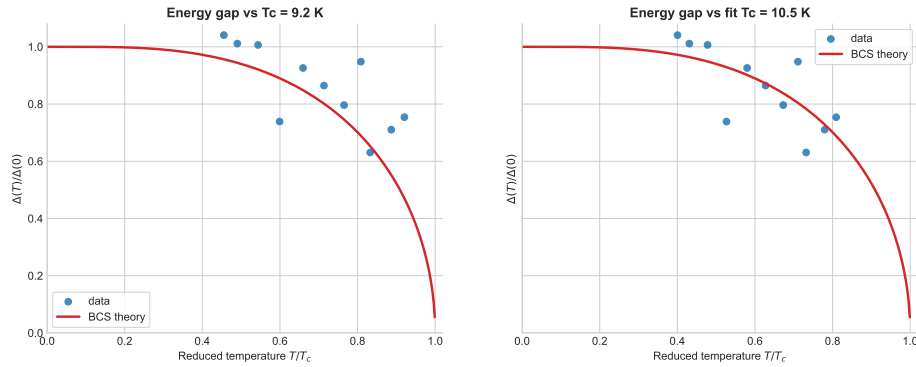
Abbildung 3: Energie-Lücke \Delta(T)/\Delta(0) gegen reduzierte Temperatur T/T_c . Links für Literaturwerte von T_c = 9.2 K und rechts für den Fit der kritischen Temperatur T_c = 10.5 K.
