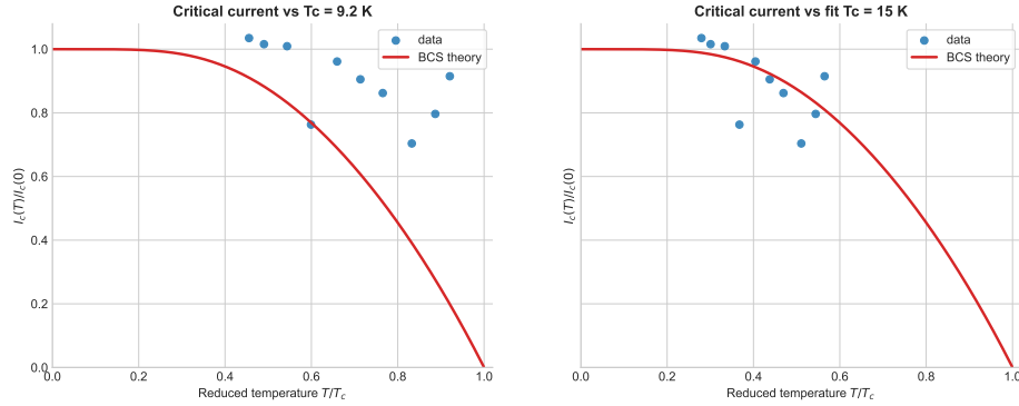
Abbildung 2: Kritischer Strom I_c(T)/I_c(0) gegen reduzierte Temperatur T/T_c . Links für Literaturwerte von T_c = 9.2 K und rechts für den Fit der kritischen Temperatur T_c = 15 K.
