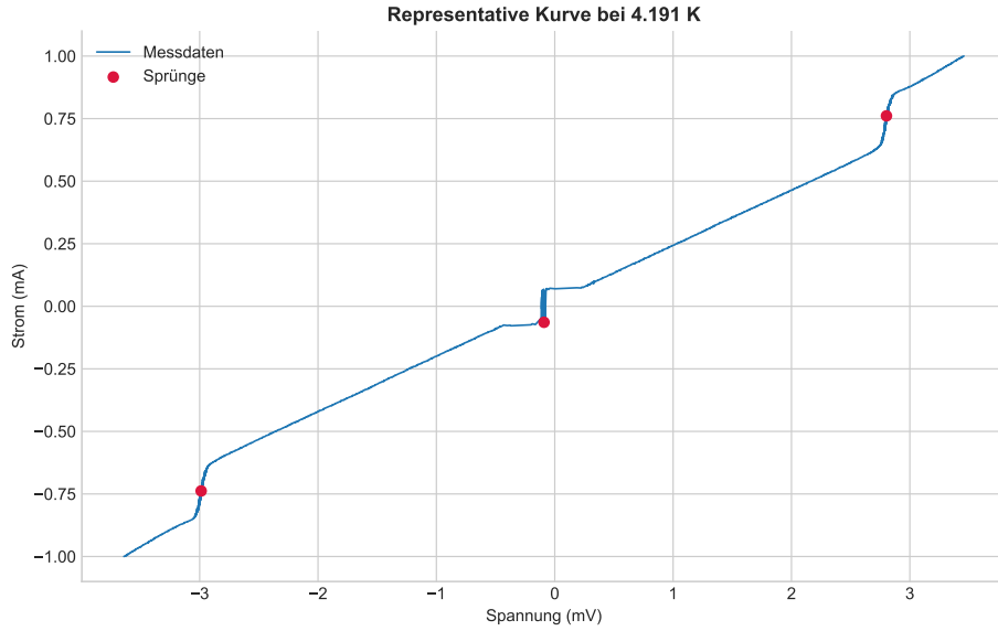
Abbildung 4: Es ist die gemessene Strom-Spannungs-Kennlinie bei einer Temperatur von T = 4.2 \text{ K} zu sehen. Die Sprünge drei Sprünge jeweils sind mit einem roten Punkten markiert.
