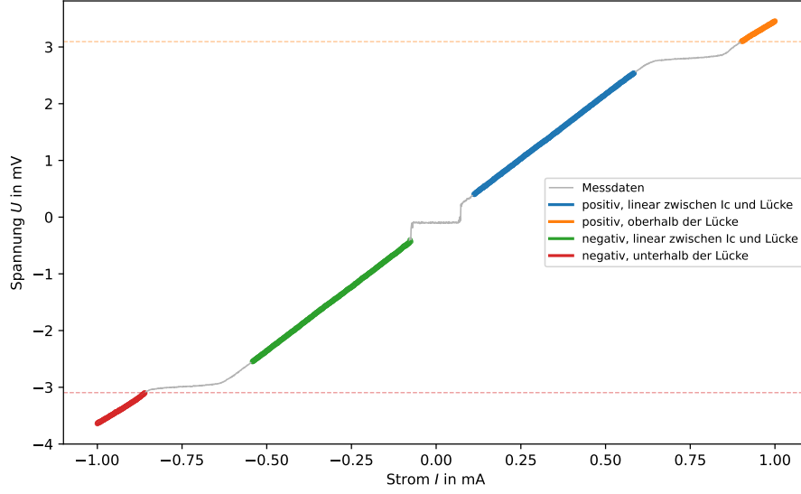
Abbildung 7: Strom-Spannungs-Kennlinie bei T = 4.2 \text{ K} und B = 0 \text{ T} . Die eingefärbten Bereiche zeigen jeweils die Bereiche an in denen gefittet wurde.
