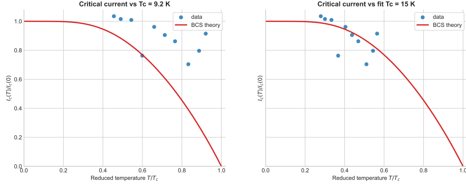
Abbildung 5: Kritischer Strom I_c(T)/I_c(0) gegen reduzierte Temperatur T/T_c . Links für Literaturwerte von T_c = 9.2 K und rechts für den Fit der kritischen Temperatur T_c = 15 K.
