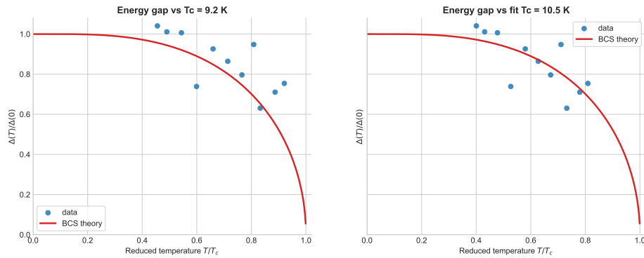
Abbildung 6: Energie-Lücke \Delta(T)/\Delta(0) gegen reduzierte Temperatur T/T_c . Links für Literaturwerte von T_c = 9.2 K und rechts für den Fit der kritischen Temperatur T_c = 10.5 K.
