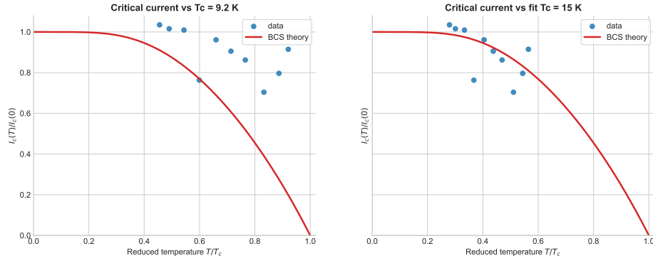
Abbildung 2: Kritischer Strom I_c(T)/I_c(0) gegen reduzierte Temperatur T/T_c . Links für Literaturwerte von T_c = 9.2\text{ K} und rechts für den Fit der kritischen Temperatur T_c = 15\text{ K} .
