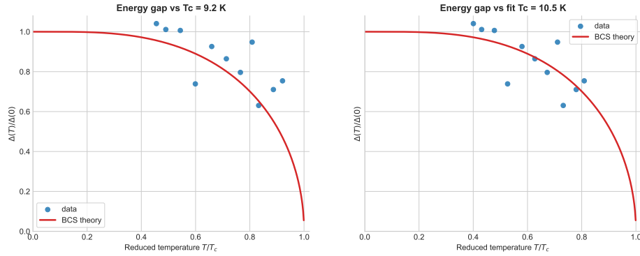
Abbildung 3: Energie-Lücke \Delta(T)/\Delta(0) gegen reduzierte Temperatur T/T_c . Links für Literaturwerte von T_c = 9.2\text{ K} und rechts für den Fit der kritischen Temperatur T_c = 10.5\text{ K} .
