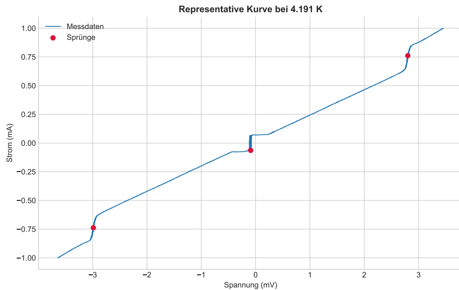
Abbildung 1: Es ist die gemessene Strom-Spannungs-Kennlinie bei einer Temperatur von T = 4.2 K zu sehen. Die Sprünge drei Sprünge jeweils sind mit einem roten Punkten markiert.
