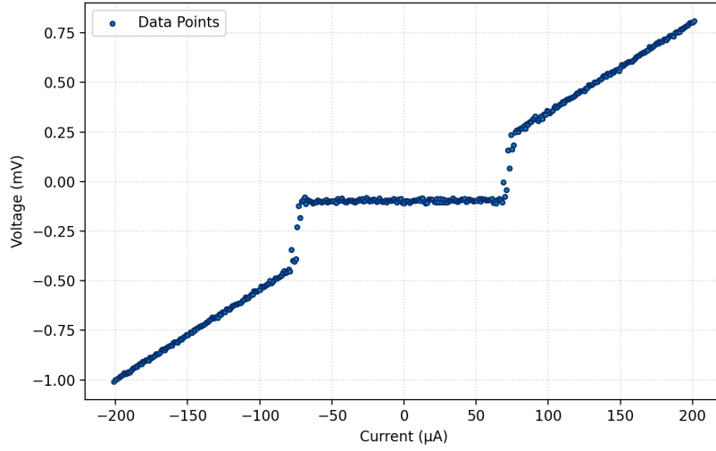
Abbildung 1: Aufgenommene Spannung-Strom-Kennlinie für eine angelegte Spulenspannung von -0.5 Volt bei 4.2 K. Die Sprünge bei V = \pm 2\Delta/e sind deutlich zu erkennen.
