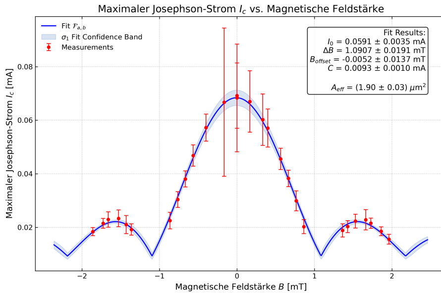
Abbildung 2: Maximaler Josephson-Strom I_C in Abhängigkeit der angelegten Magnetfeldstärke der Helmholtz-Spulen. Die Ergebnisse wurden an die Theorie der Fraunhofer-Interferenz gefittet. Zusätzlich sind noch die Konfidenzintervalle für \sigma_1 basierend auf den Fehlern der Fits für die maximalen Josephson-Ströme dargestellt.
