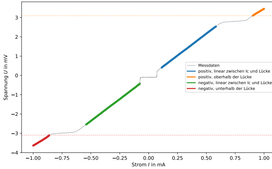
Abbildung 6: Strom-Spannungs-Kennlinie bei T = 4.2 \text{ K} und B = 0 \text{ T} . Die eingefärbten Bereiche zeigen jeweils die Bereiche an in denen gefittet wurde.
