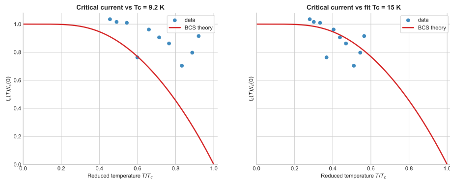
Abbildung 4: Kritischer Strom I_c(T)/I_c(0) gegen reduzierte Temperatur T/T_c . Links für Literaturwerte von T_c = 9.2 \text{ K} und rechts für den Fit der kritischen Temperatur T_c = 15 \text{ K} .
