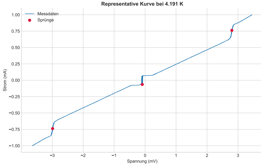
Abbildung 3: Es ist die gemessene Strom-Spannungs-Kennlinie bei einer Temperatur von T = 4.2 \text{ K} zu sehen. Die Sprünge drei Sprünge jeweils sind mit einem roten Punkten markiert.
