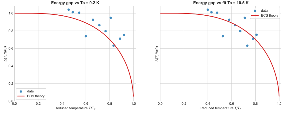
Abbildung 5: Energie-Lücke \Delta(T)/\Delta(0) gegen reduzierte Temperatur T/T_c . Links für Literaturwerte von T_c = 9.2\text{ K} und rechts für den Fit der kritischen Temperatur T_c = 10.5\text{ K} .
