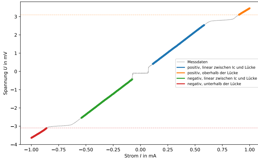
Abbildung 6: Strom-Spannungs-Kennlinie bei T = 4.2 \text{ K} und B = 0 \text{ T} . Die eingefärbten Bereiche zeigen jeweils die Bereiche an in denen gefittet wurde.
