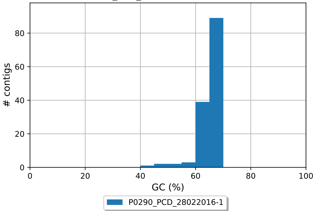
P0290_PCD_28022016-1 GC content
