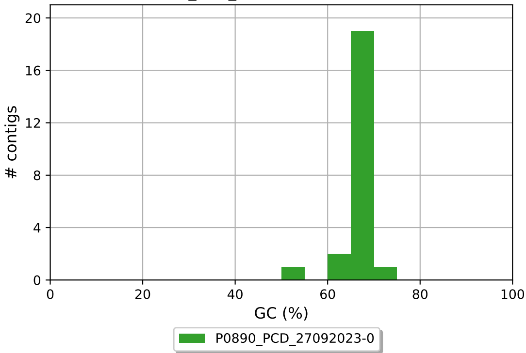
P0890_PCD_27092023-0 GC content
