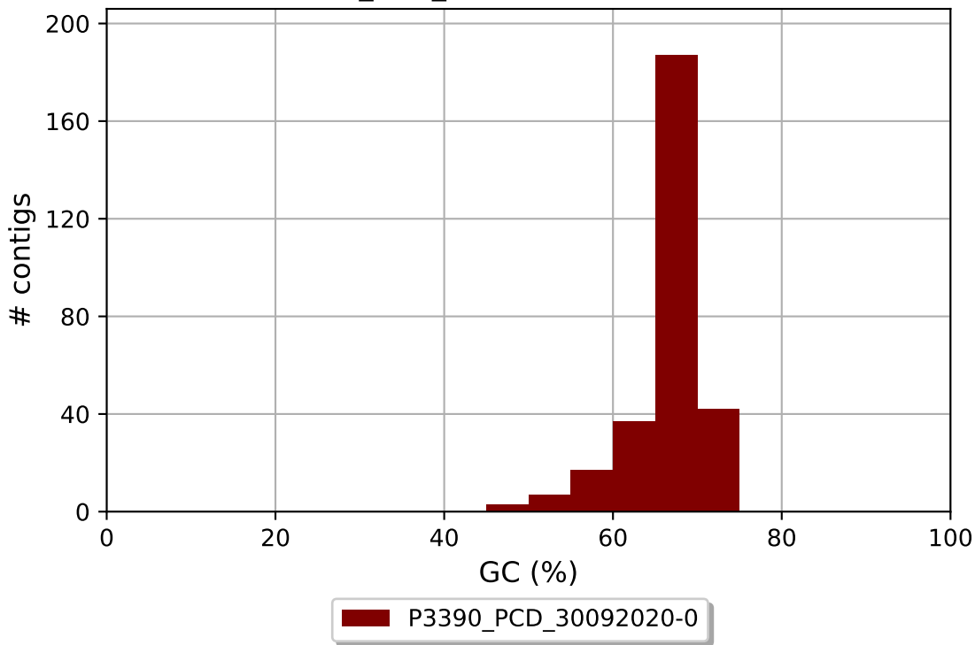
P3390_PCD_30092020-0 GC content
