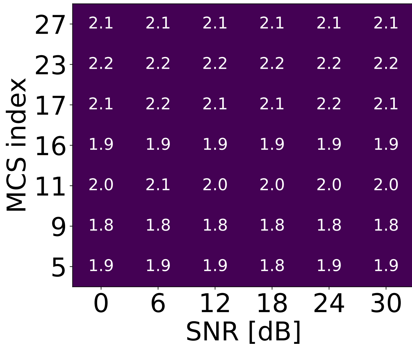
GPU 1024 CBs
