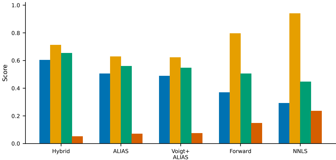
Precision Recall F1 FPR Best configuration per identification pathway
