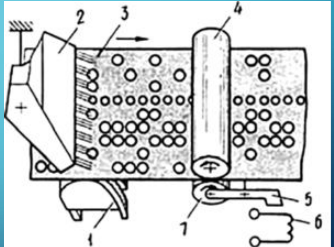
1 - контактная колодка, 2 - головка, 3 - перфолента, 4 - ведущий вал, 5 - рычаг, 6 - электромагнит протяжки, 7 - прижимной ролик
