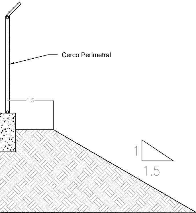
DETALLE DE TALUD DE RELLENO Sin Escala
