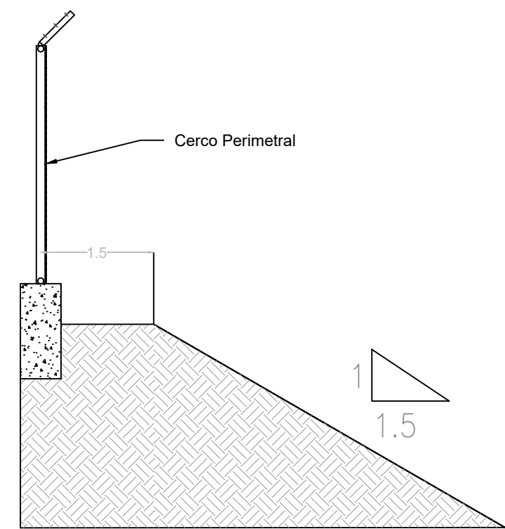
DETALLE DE TALUD DE RELLENO Sin Escala
