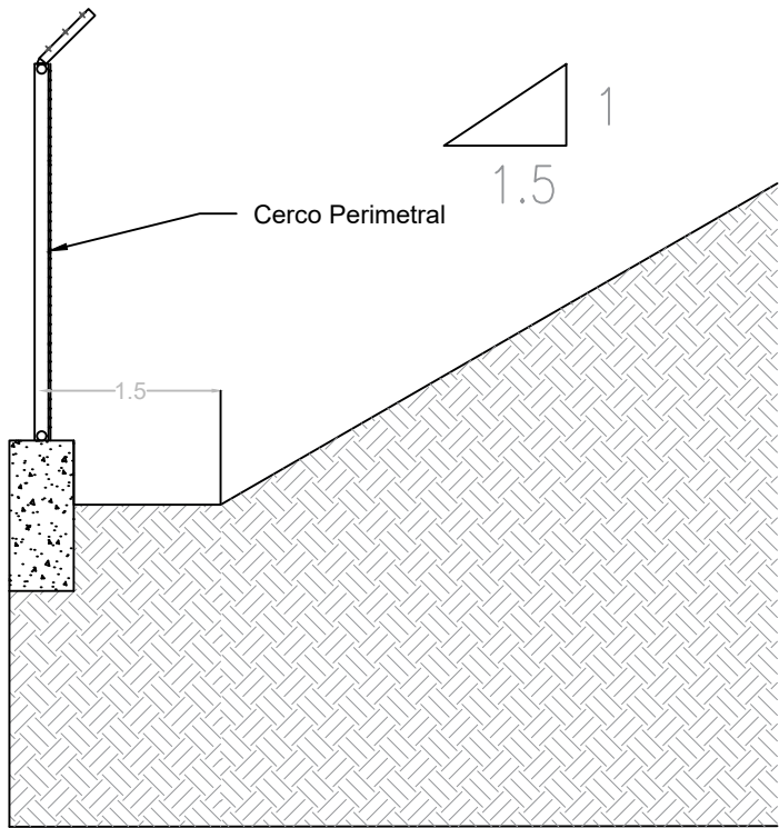
DETALLE DE TALUD DE CORTE Sin Escala
