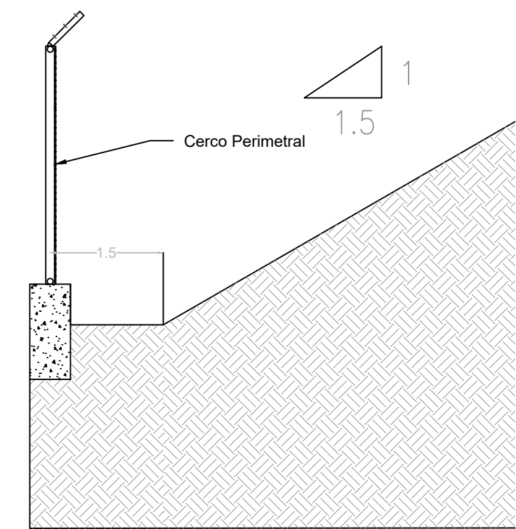
DETALLE DE TALUD DE CORTE Sin Escala
