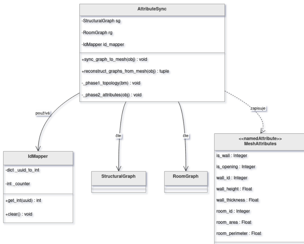
■ Obrázek 4 Diagram tříd na vrstvě 3
