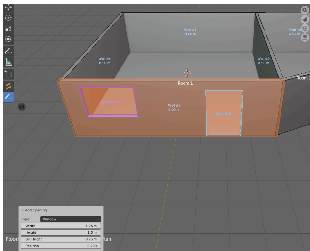
Obrázek 19 Vložení další parametrického otvoru, tentokrát okna a úprava jeho hodnot
