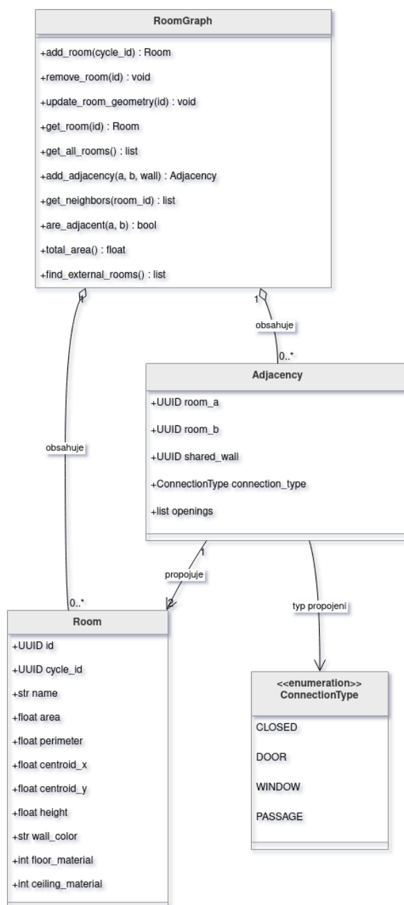
■ Obrázek 7 Diagram tříd na vrstvě 2
