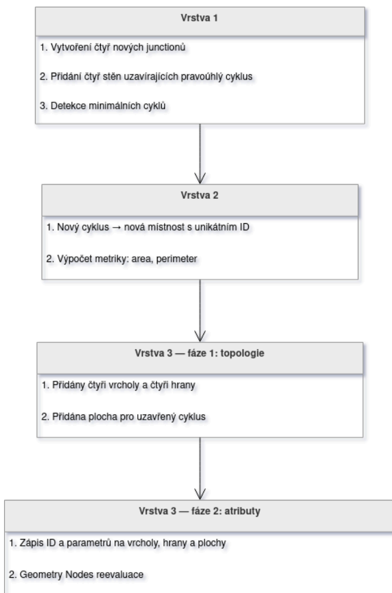
■ Obrázek 2 Tok dat: Přidání místnosti / uzavření cyklu
