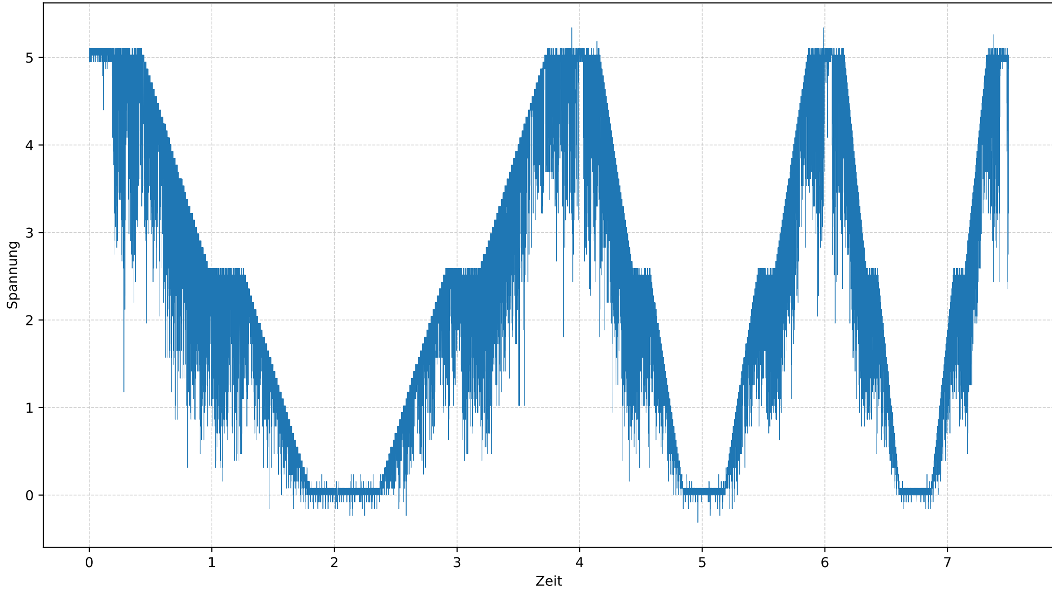
Rauschkurve Poti01_T01
