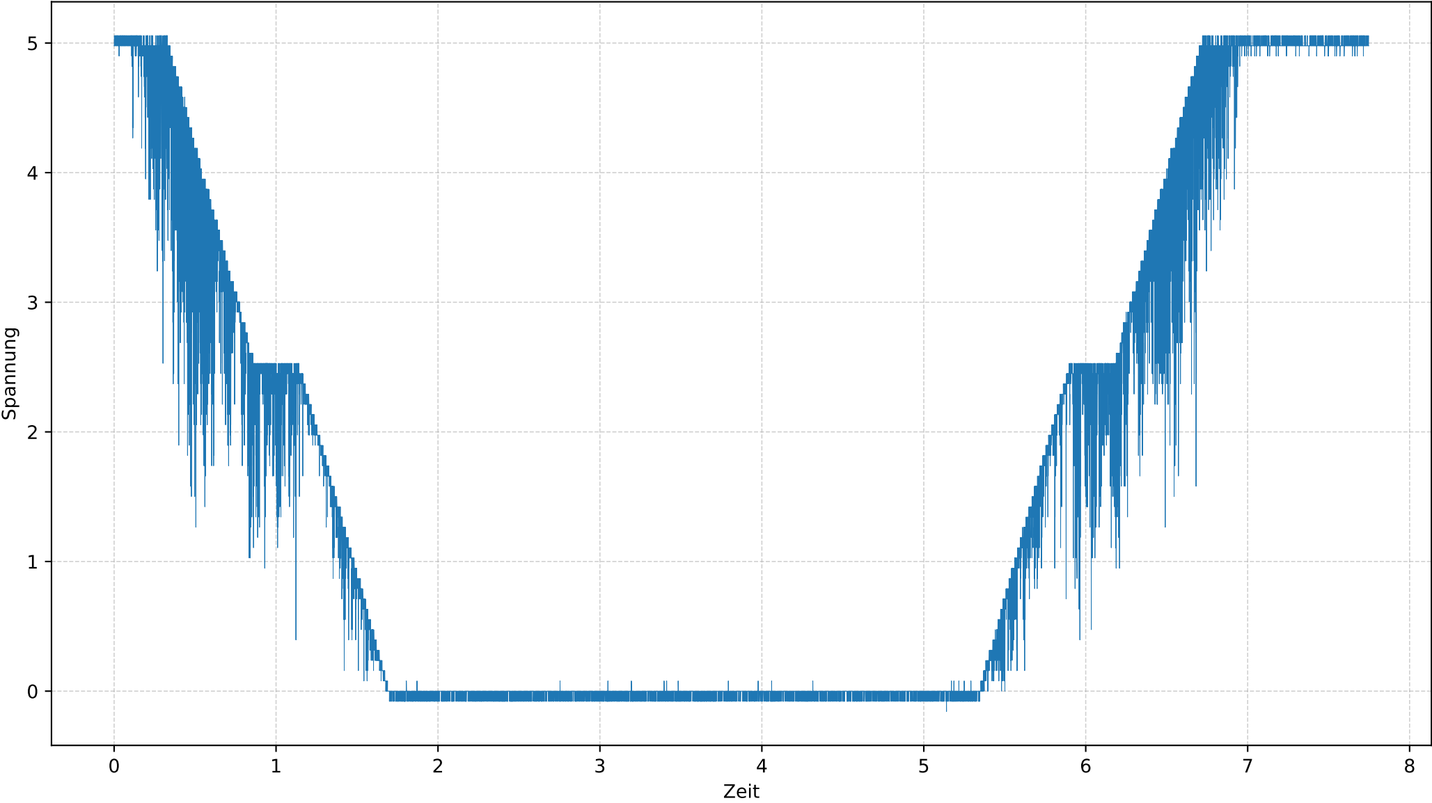
Rauschkurve 2222222222222222222222
