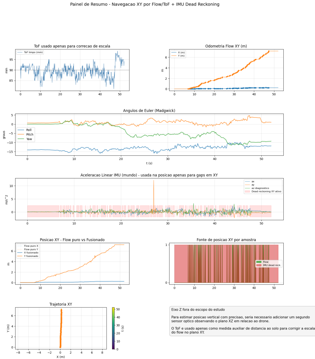
Imagem 4.4: Resumo visual do processamento de navegação, incluindo ToF, odometria óptica, atitude, aceleração linear e trajetória final no plano XY.
