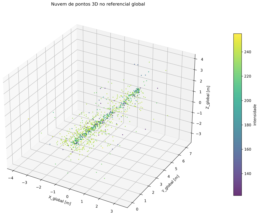
Imagem 4.2: Representação tridimensional da nuvem de pontos global obtida a partir da transformação dos dados do LiDAR para o referencial global.
