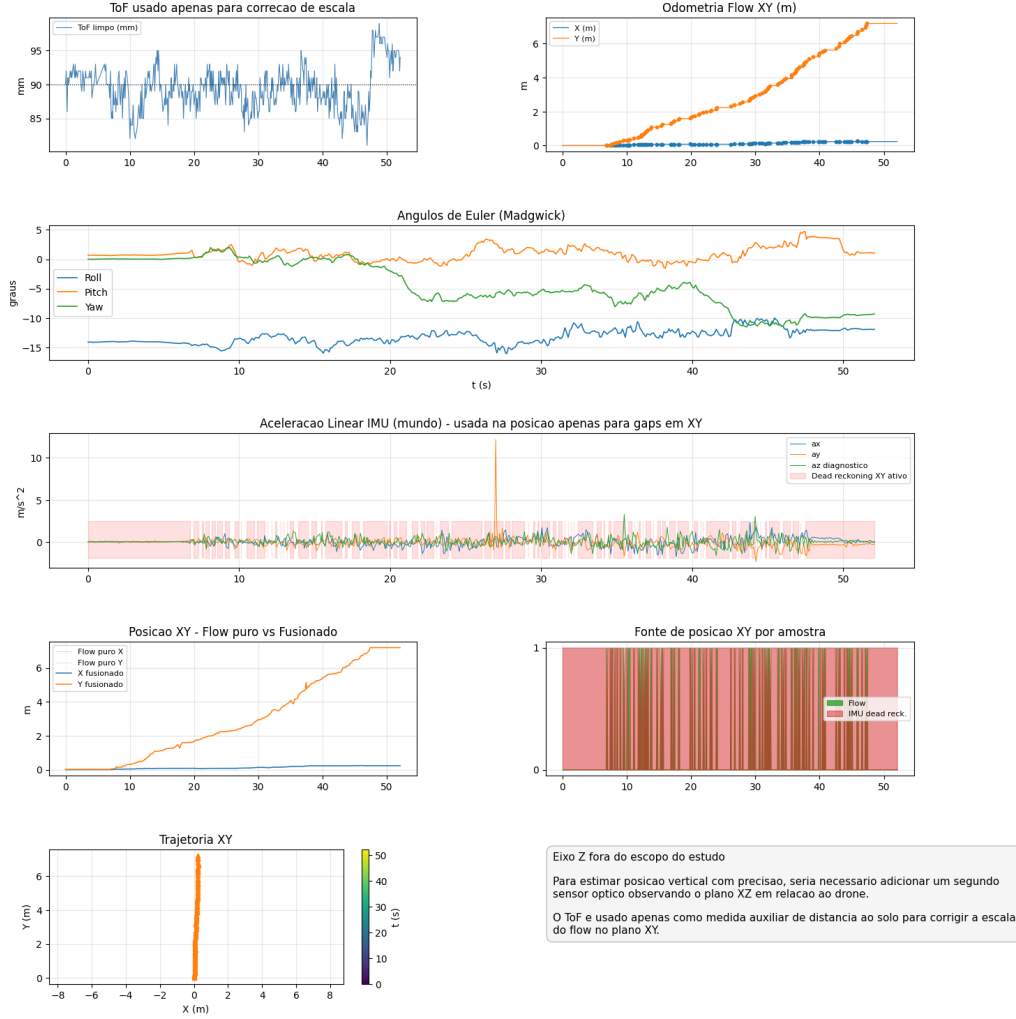
Imagem 4.2: Resumo visual do processamento de navegação, incluindo ToF, odometria óptica, atitude, aceleração linear e trajetória final no plano XY.
