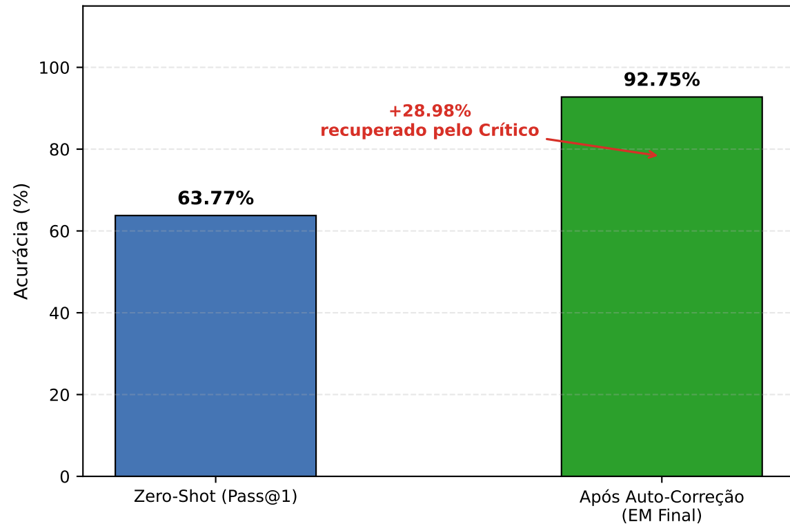
(a) Ganho Epistêmico do Ciclo Agente-Crítico
