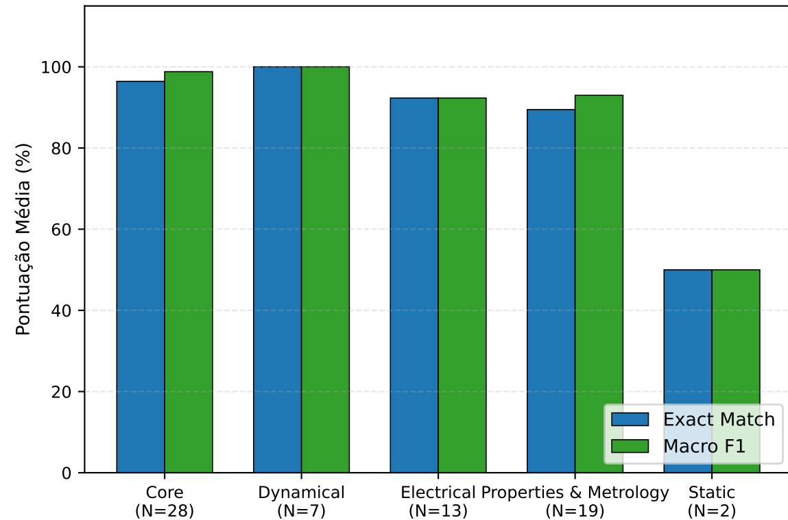
(b) Desempenho por Subdomínio Ontológico
