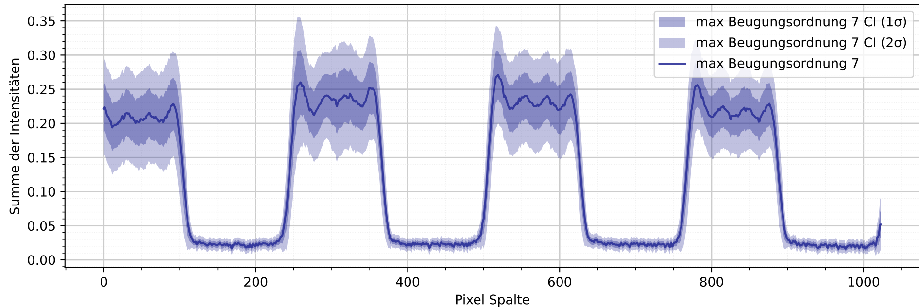
Intensitätsprofil mit Gitter 1 und max. Beugungsordnung 7
