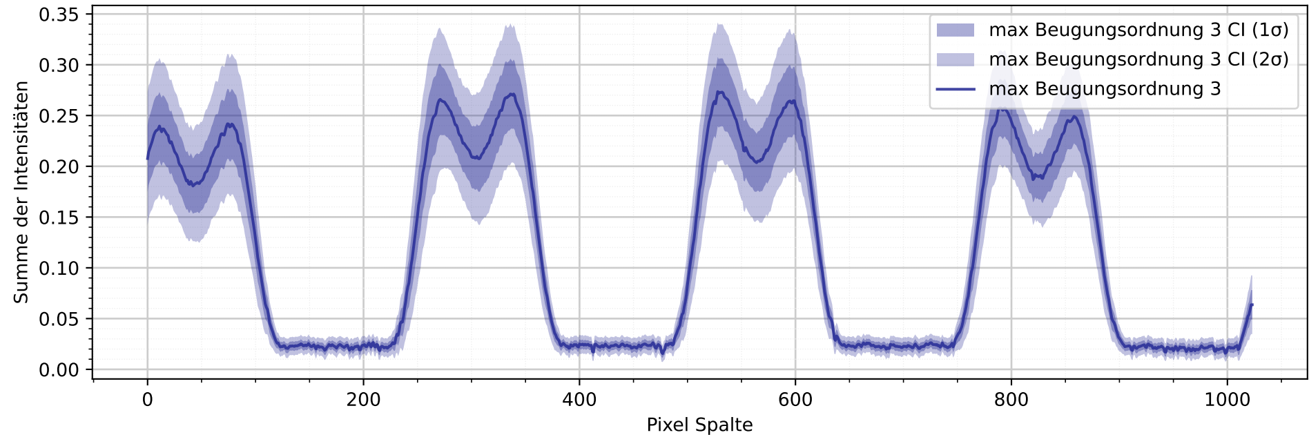
Intensitätsprofil mit Gitter 1 und max. Beugungsordnung 3
