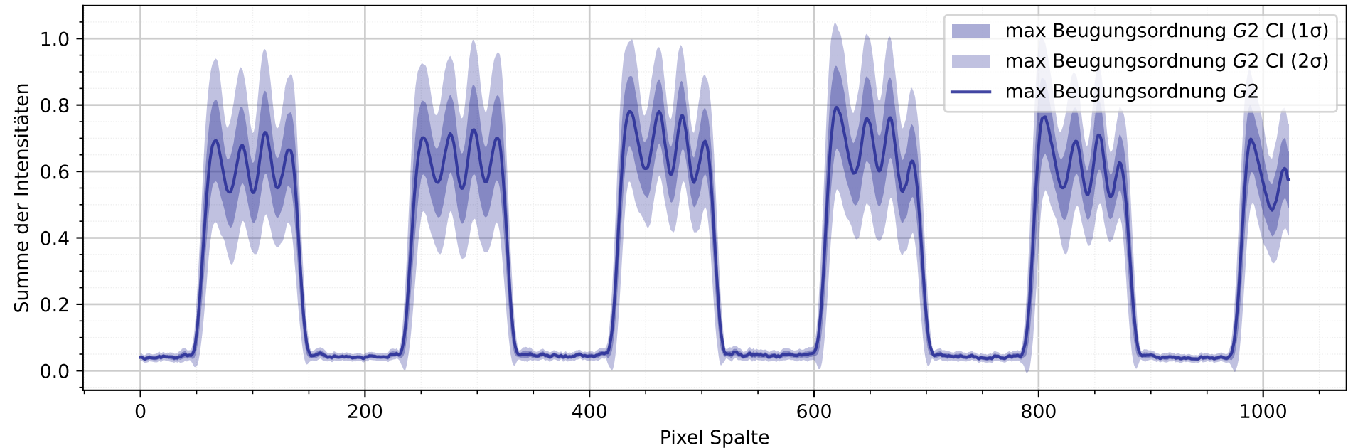
Intensitätsprofil mit Gitter 1 und max. Beugungsordnung G2
