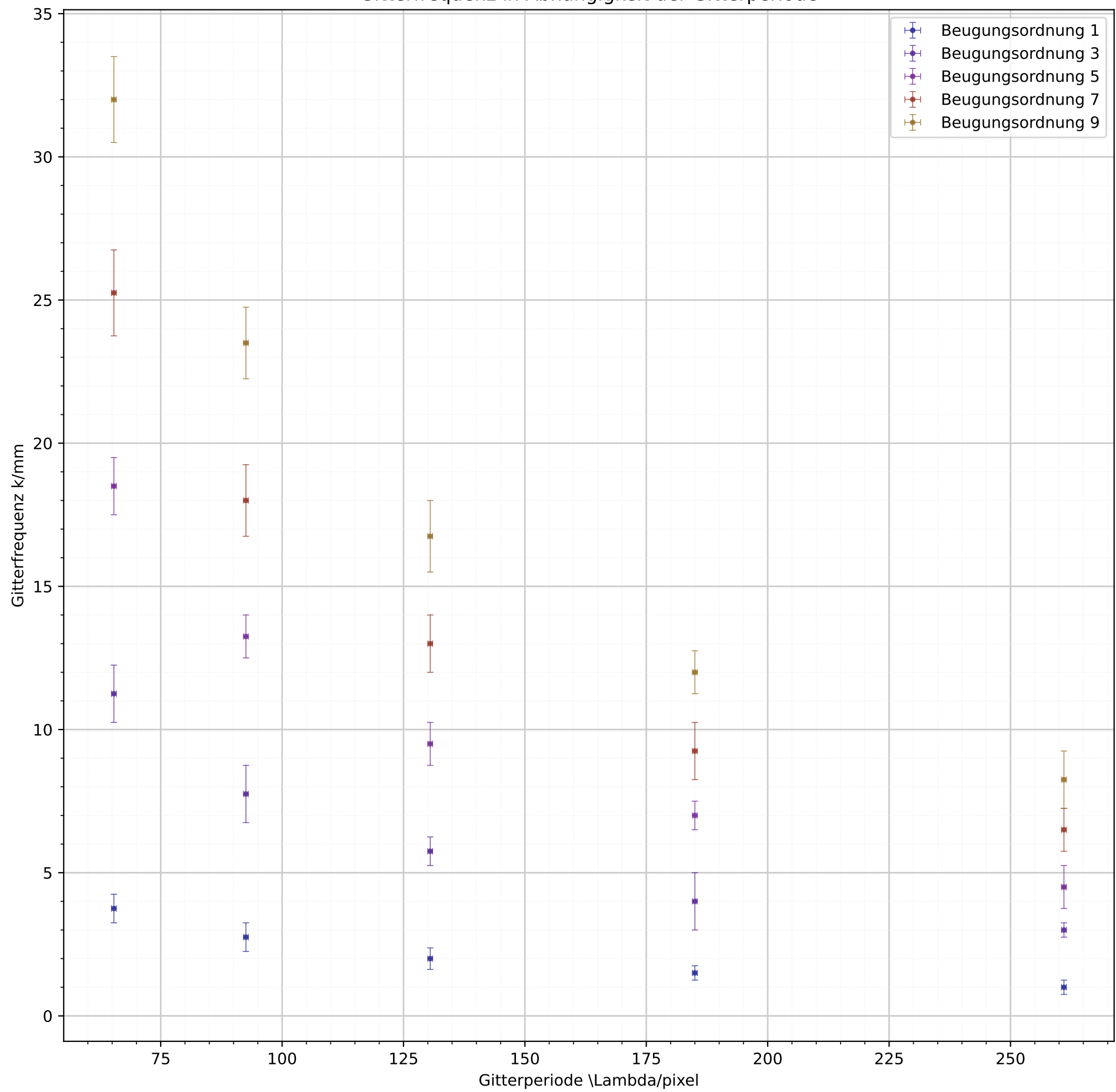
Gitterfrequenz in Abhängigkeit der Gitterperiode
