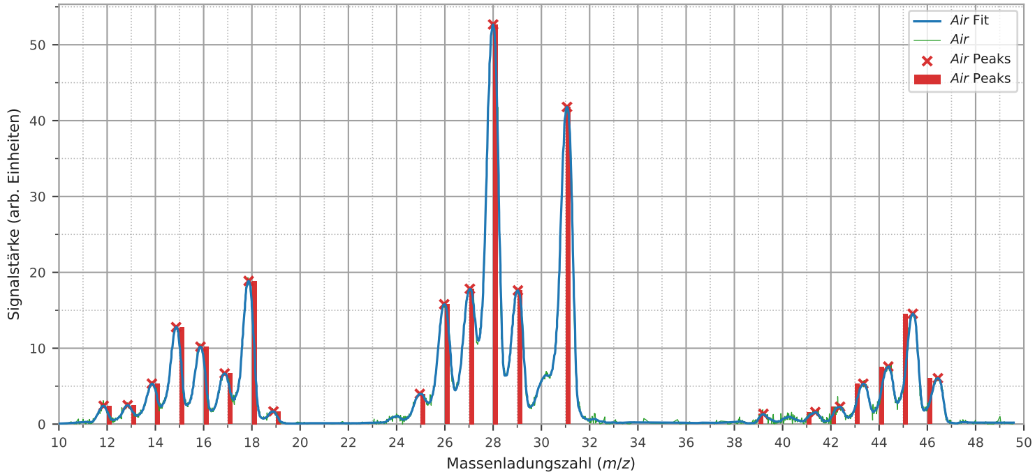
Signalstärke von Air 1 und gefundene Peaks
