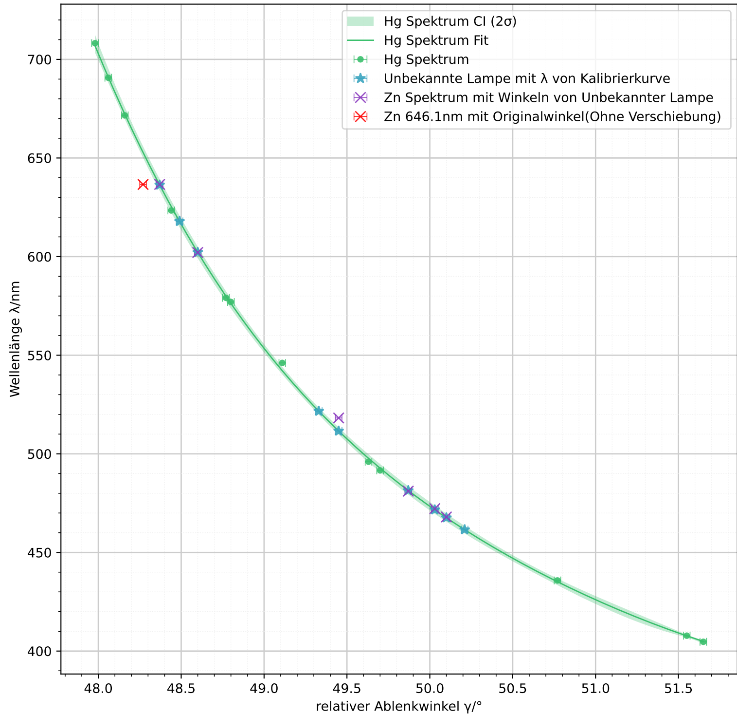
Kalibrierkurve (Spline) des Hg-Spektrums mit Zink-Spektrum
