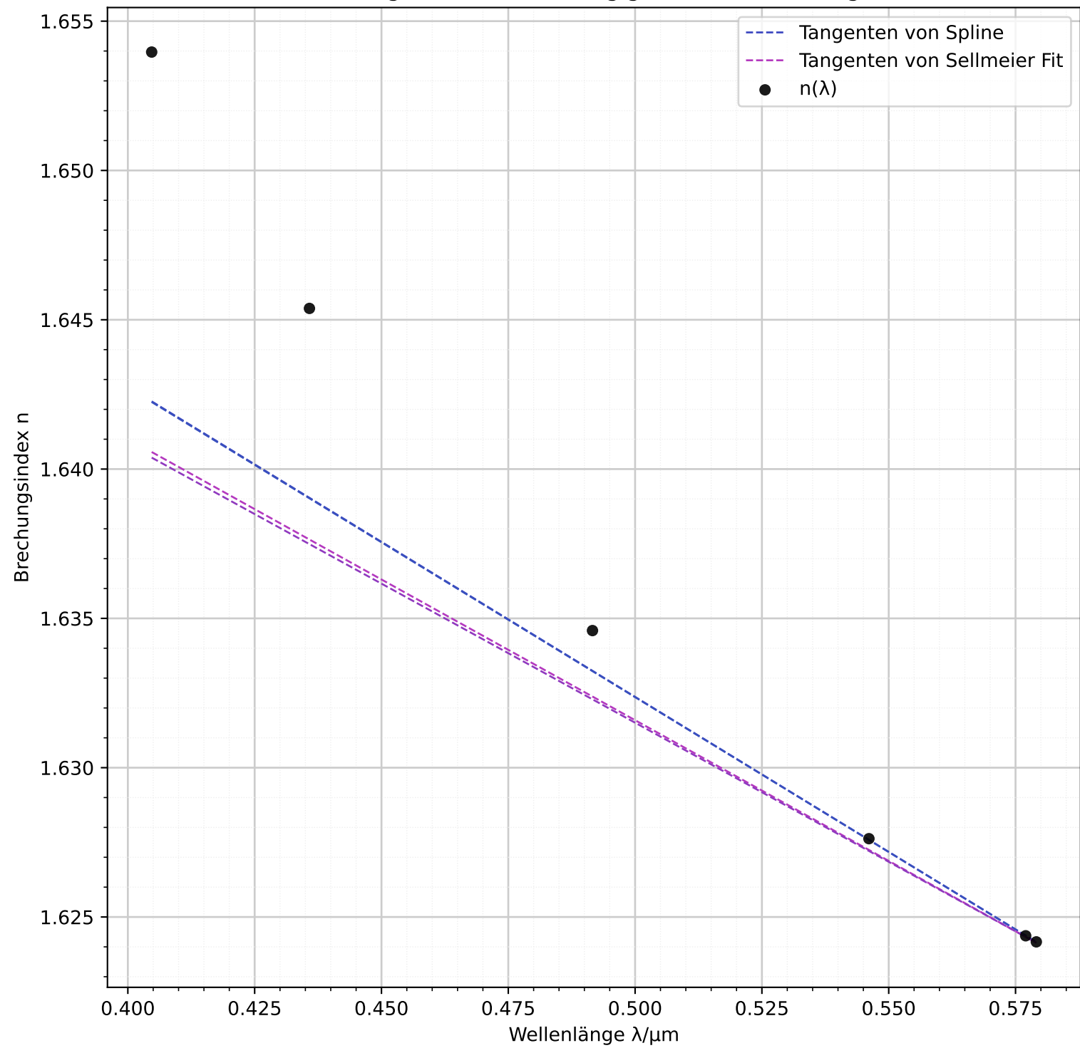
Brechungsindex n in Abhängigkeit der Wellenlänge \lambda
