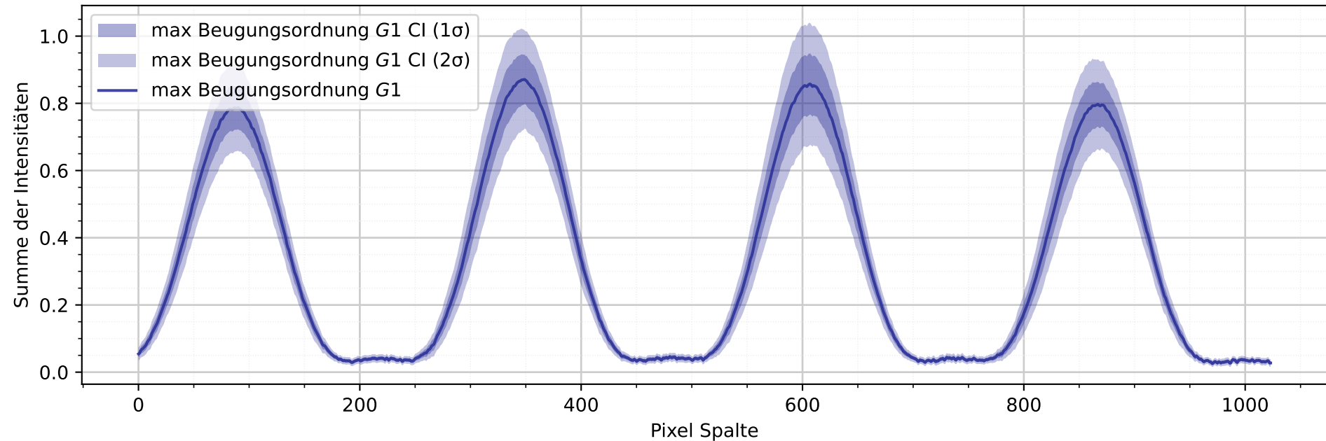
Intensitätsprofil mit Gitter 1 und max. Beugungsordnung G1
