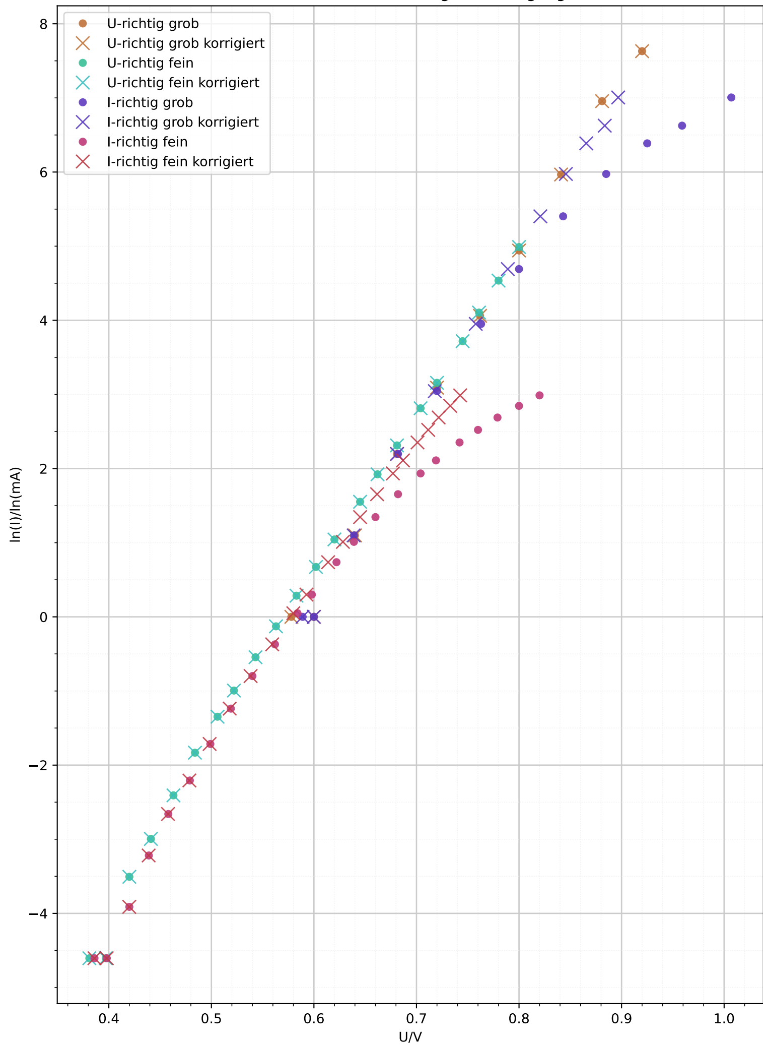
Kennlinie Diode mit U und I richtige Messung logarithmiert
