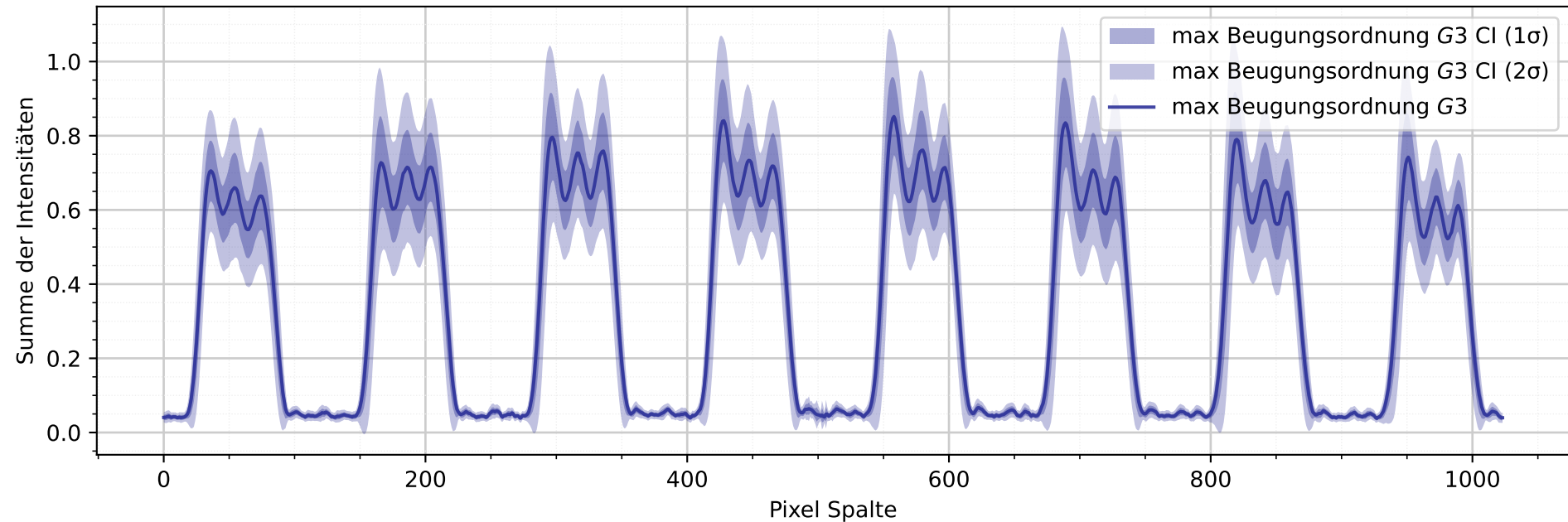
Intensitätsprofil mit Gitter 1 und max. Beugungsordnung G3
