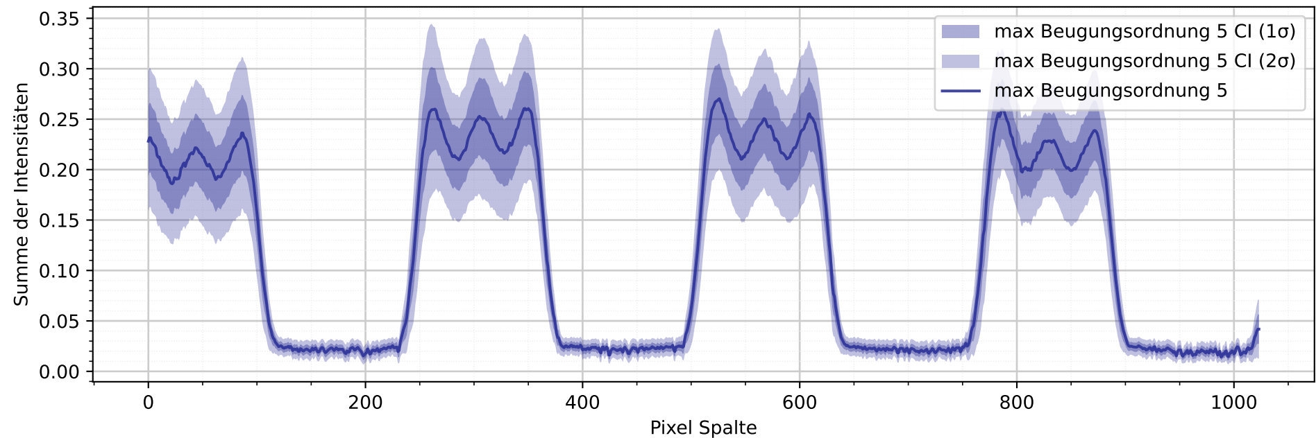
Intensitätsprofil mit Gitter 1 und max. Beugungsordnung 5
