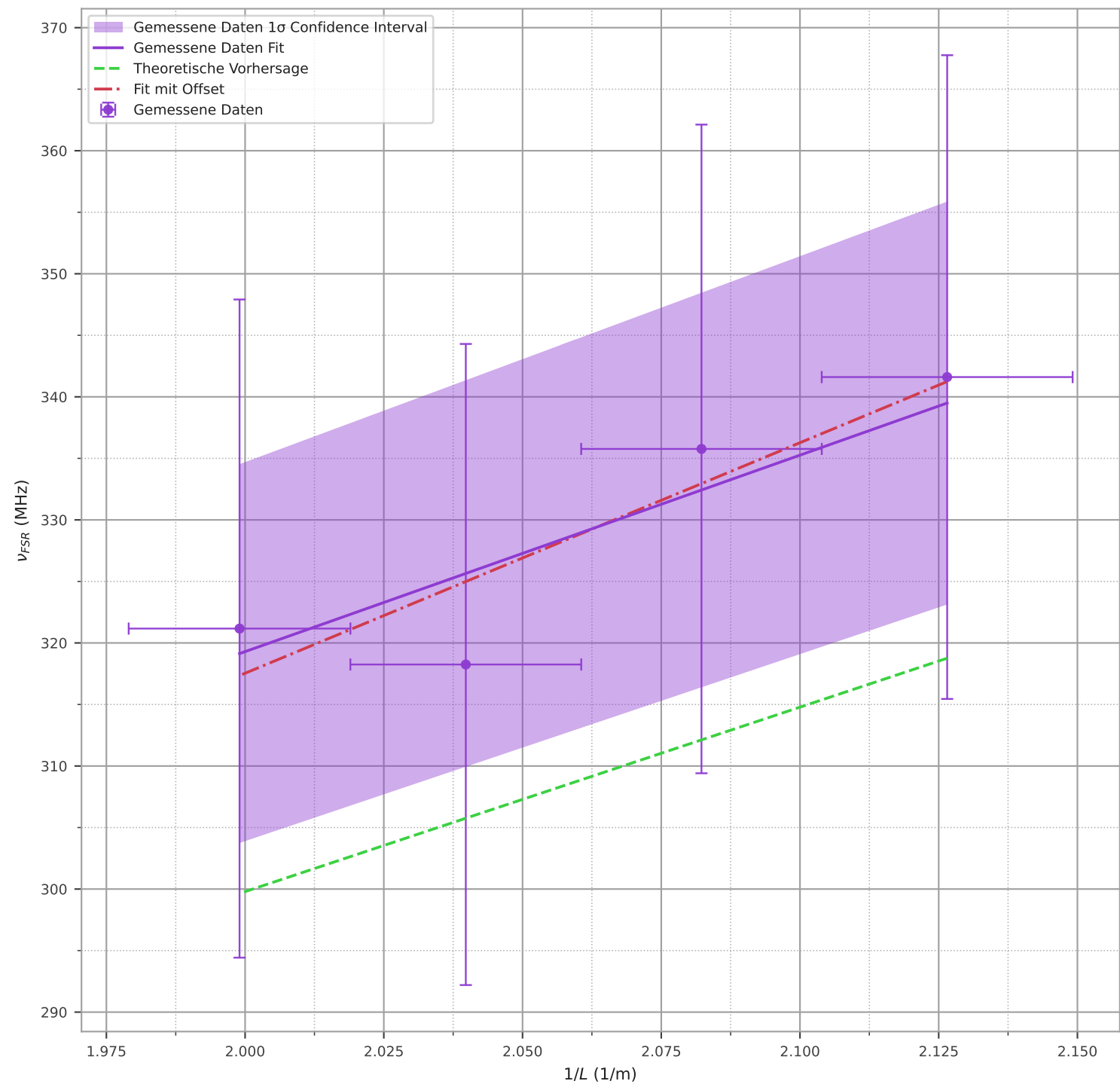
Longitudinaler Modenabstand in Abhängigkeit von 1/L
