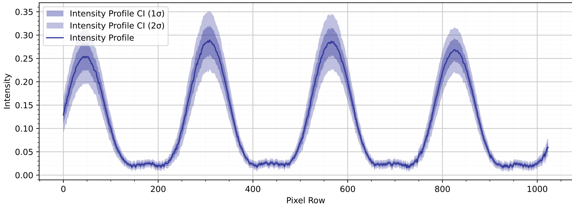
Intensitätsprofil mit Beugungsordnung 1
