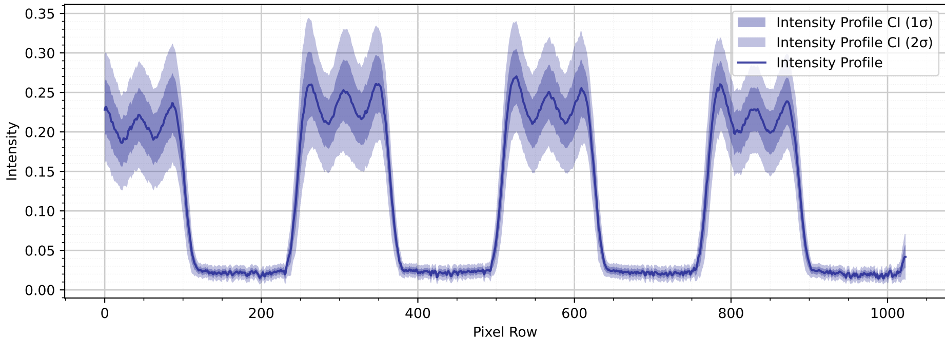
Intensitätsprofil mit Beugungsordnung 5
