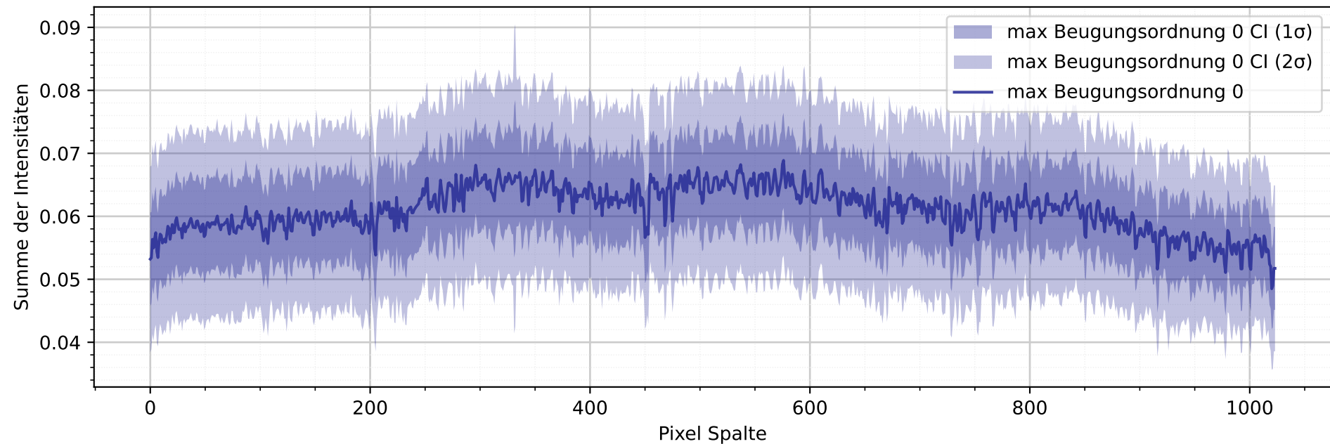
Intensitätsprofil mit Gitter 1 und max. Beugungsordnung 0
