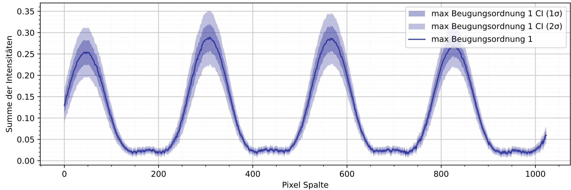
Intensitätsprofil mit Gitter 1 und max. Beugungsordnung 1
