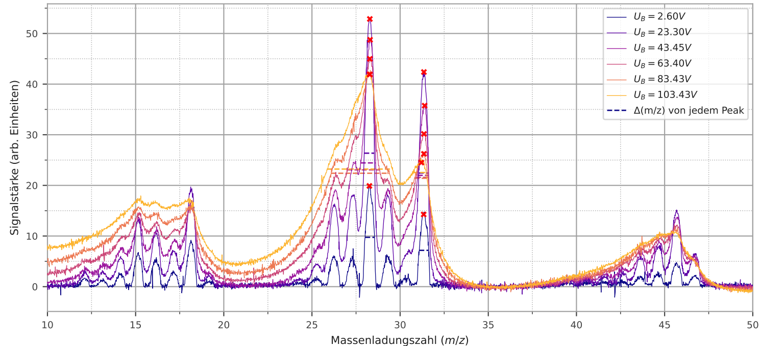
Signalstärke bei verschiedenen Spannungen
