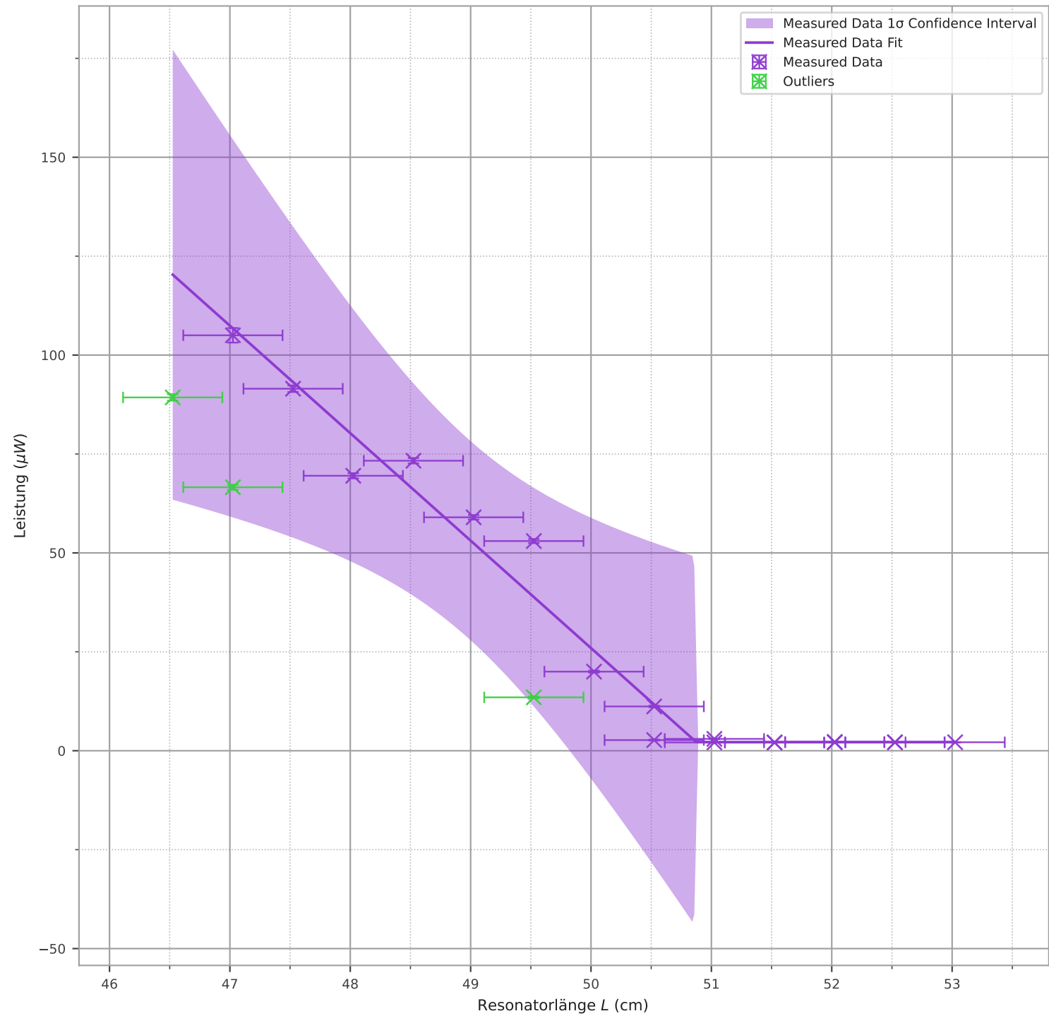
Messlaserintensität in Abhängigkeit der Resonatorlänge
