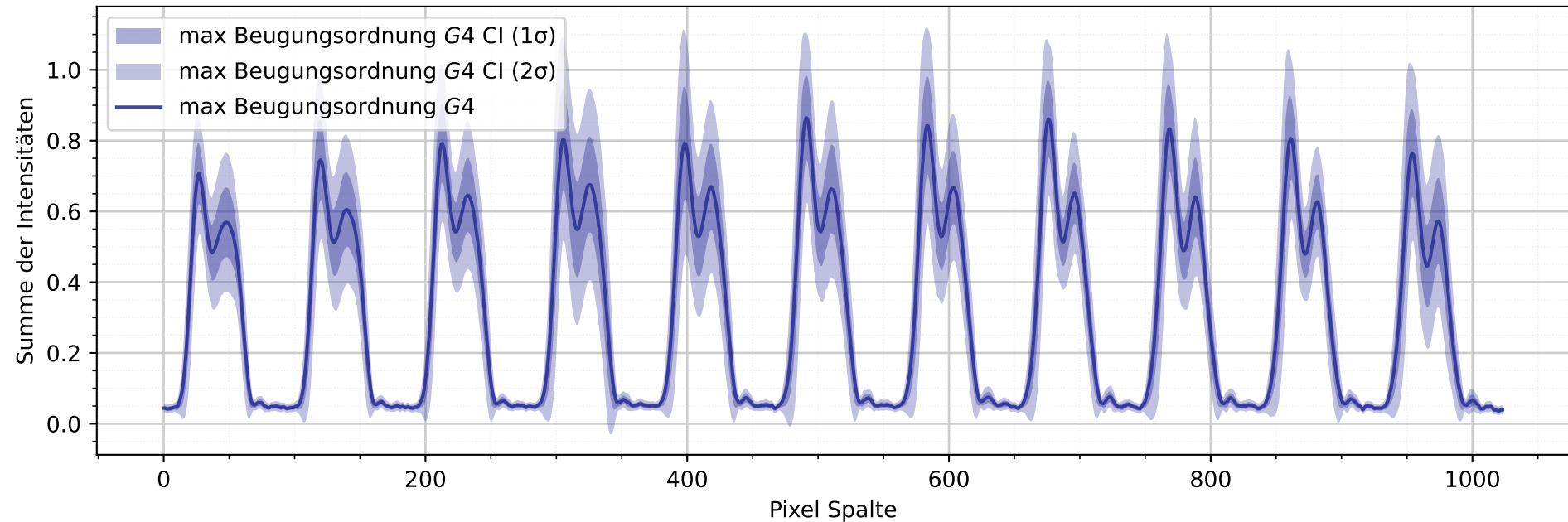
Intensitätsprofil mit Gitter 1 und max. Beugungsordnung G4
