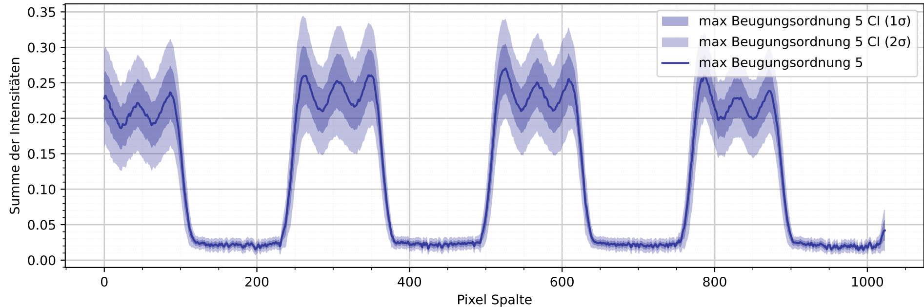
Intensitätsprofil mit Gitter 1 und max. Beugungsordnung 5
