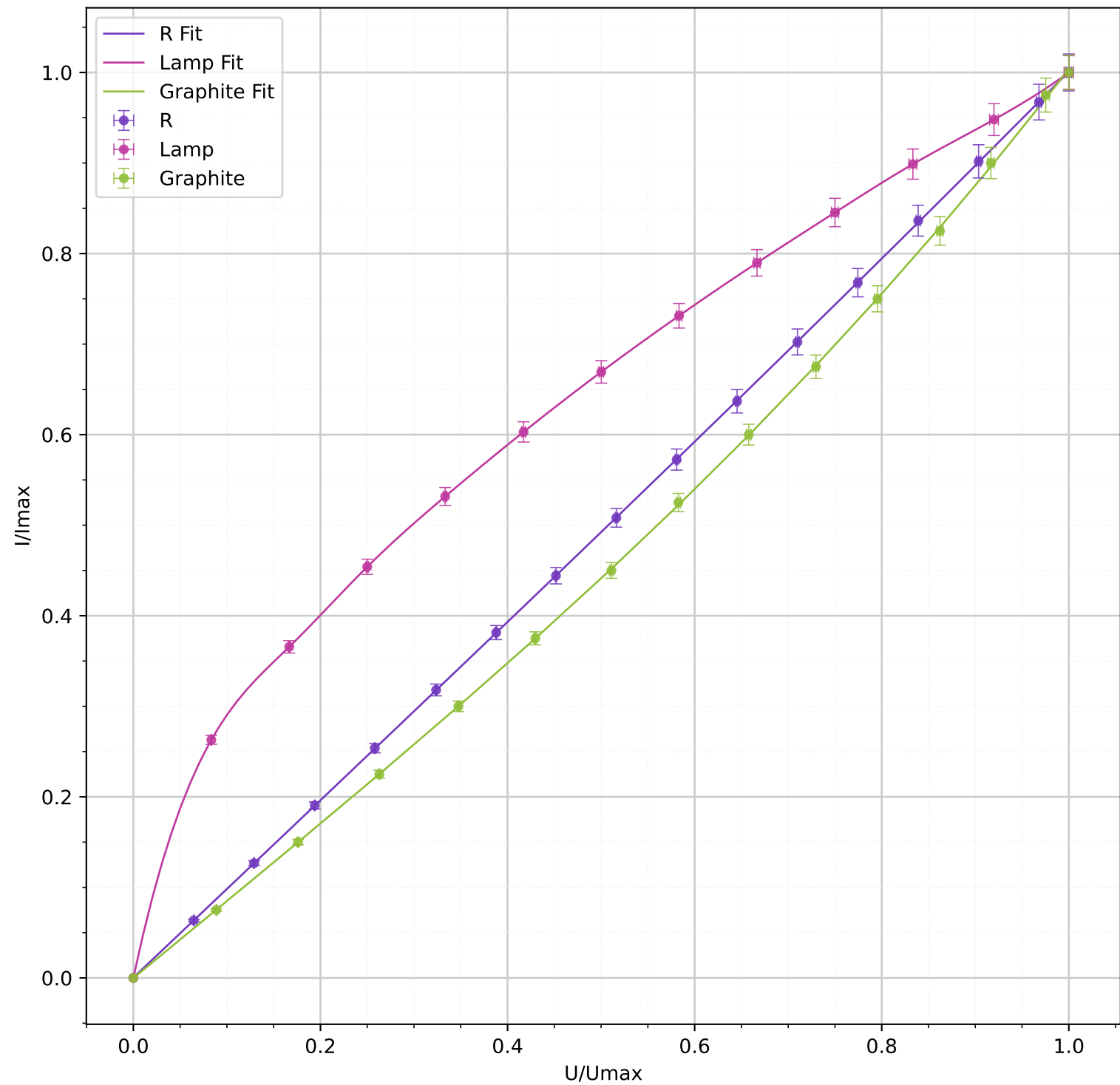
Kennlinien verschiedener Materialien
