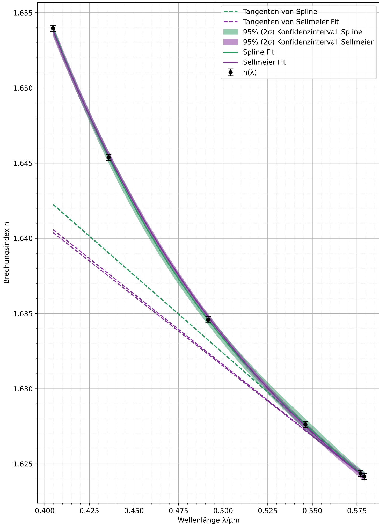
Brechungsindex n in Abhängigkeit der Wellenlänge \lambda
