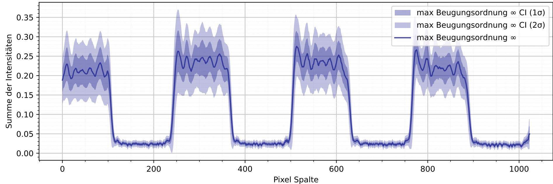
Intensitätsprofil mit Gitter 1 und max. Beugungsordnung \infty
