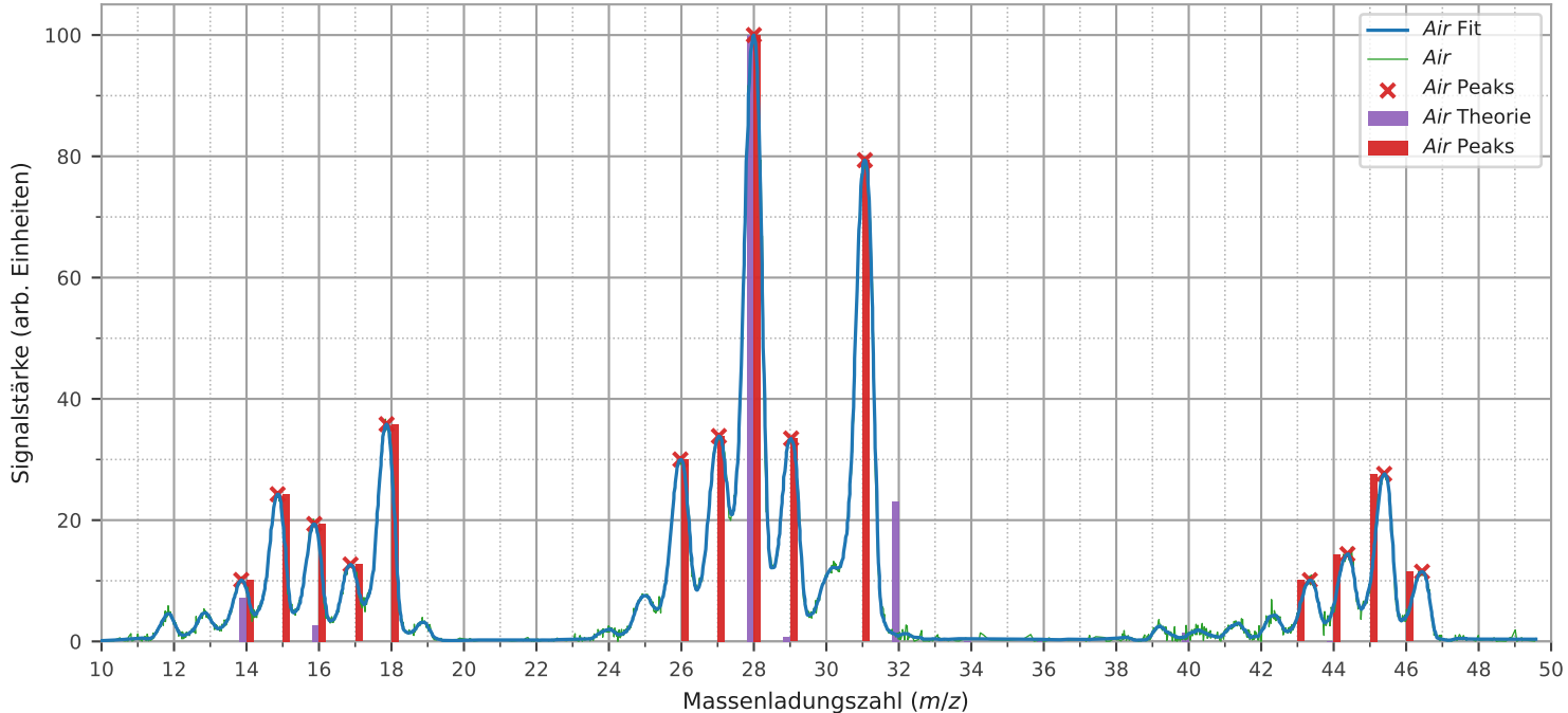
Signalstärke von Air 1 im Vergleich zur Theorie
