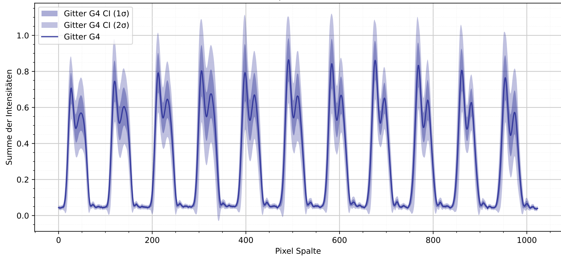
Intensitätsprofil mit Gitter G4
