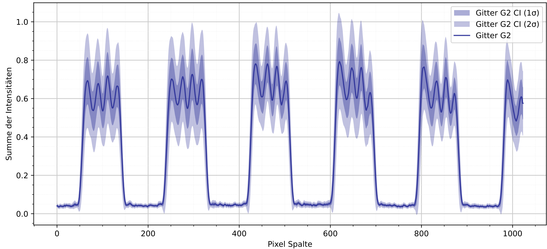
Intensitätsprofil mit Gitter G2
