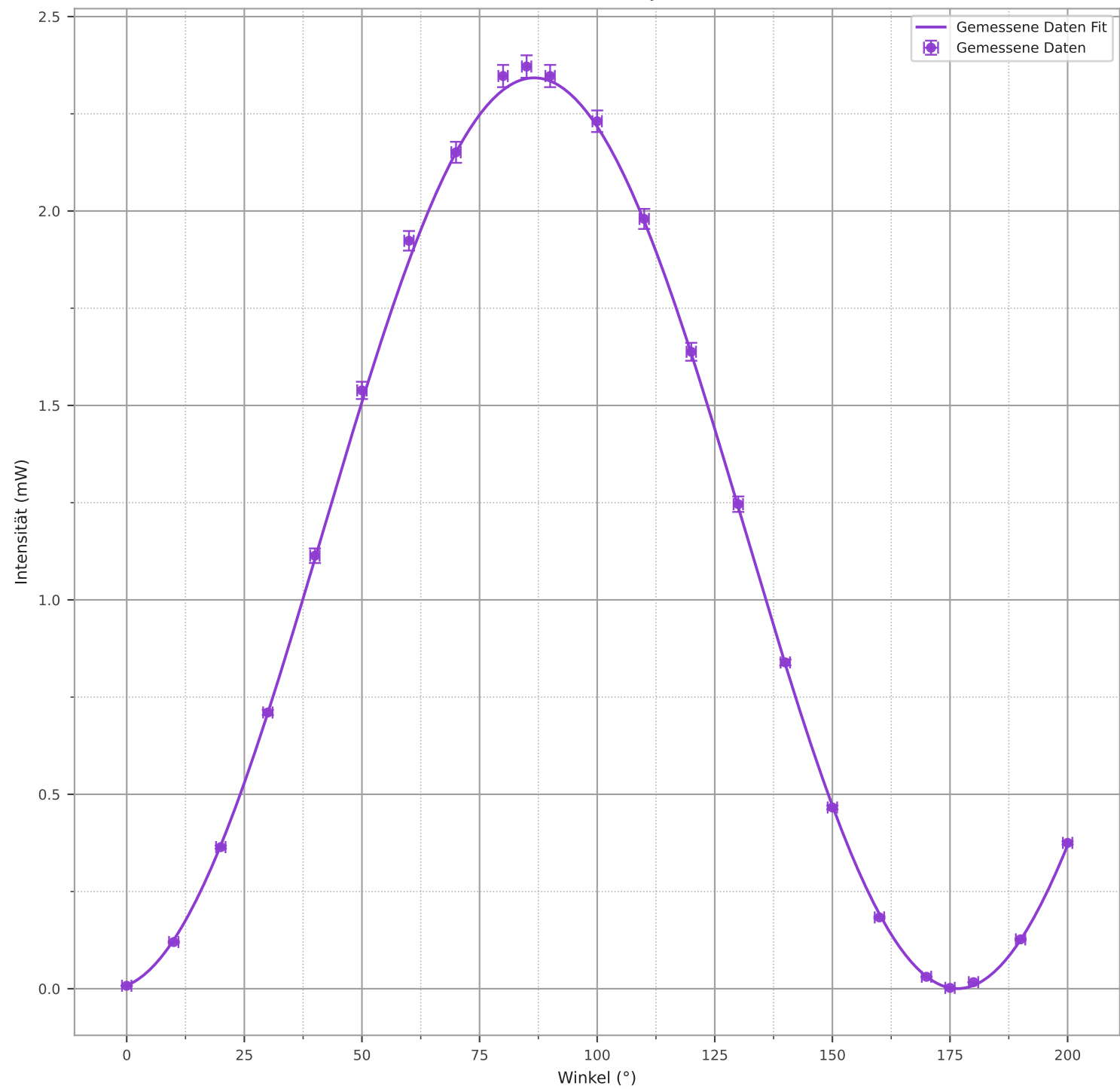
Polarisationskurve des Justierlasers
