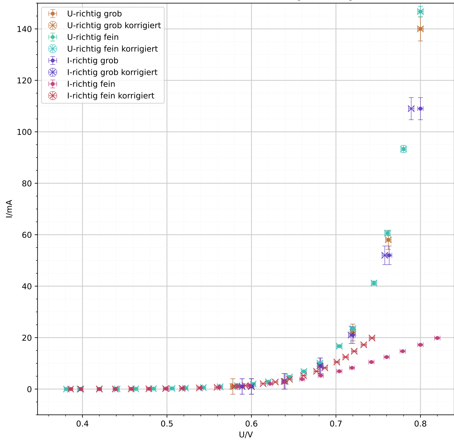
Kennlinie Diode mit U und I richtige Messung
