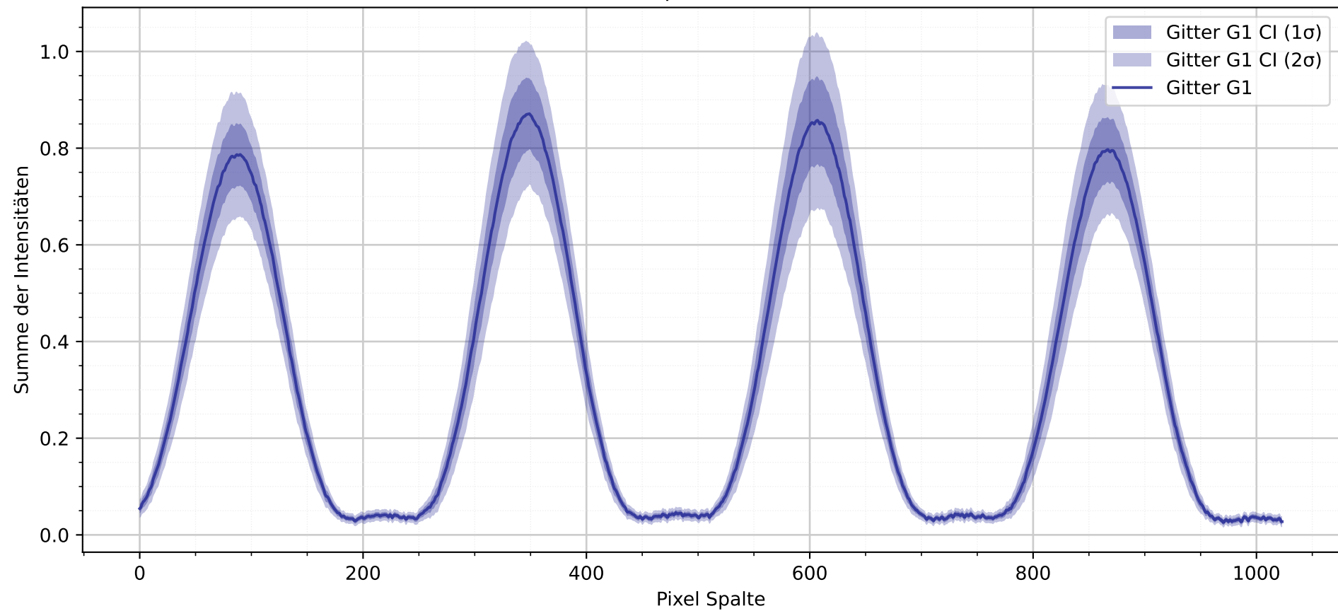
Intensitätsprofil mit Gitter G1
