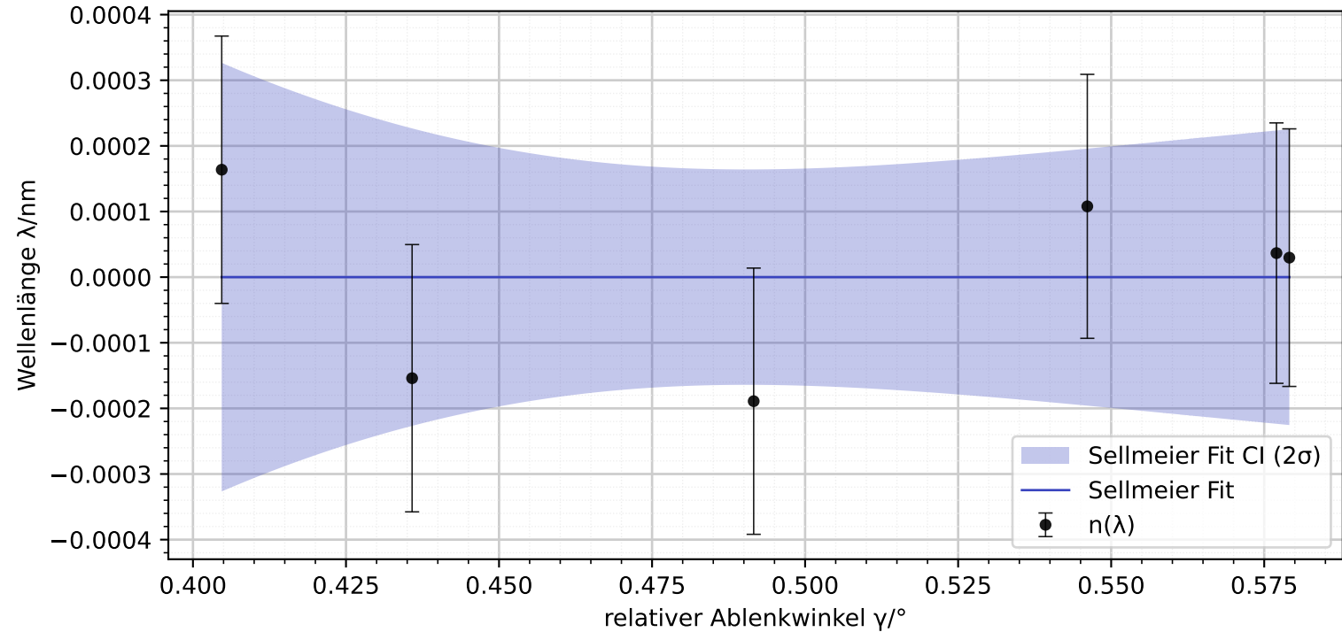
Residuen des Sellmeier Fits
