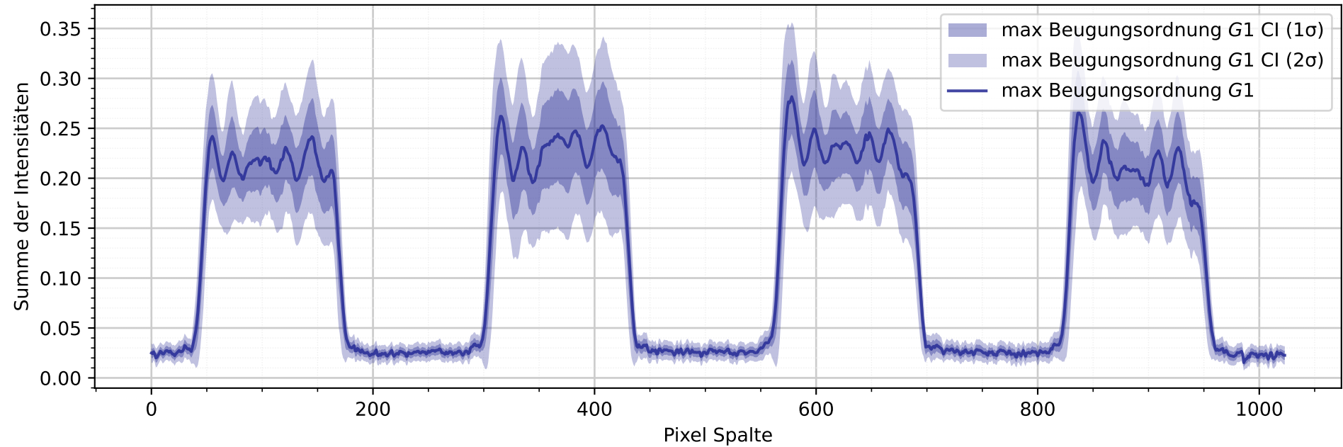
Intensitätsprofil mit Gitter 1 und max. Beugungsordnung G1
