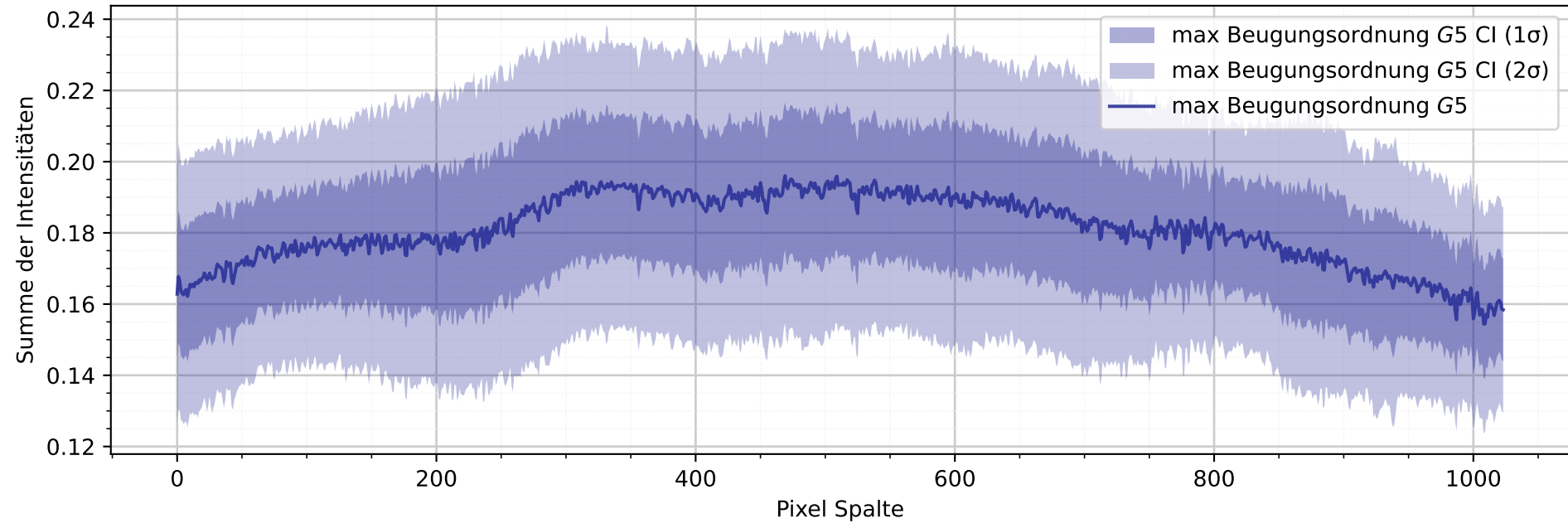
Intensitätsprofil mit Gitter 1 und max. Beugungsordnung G5
