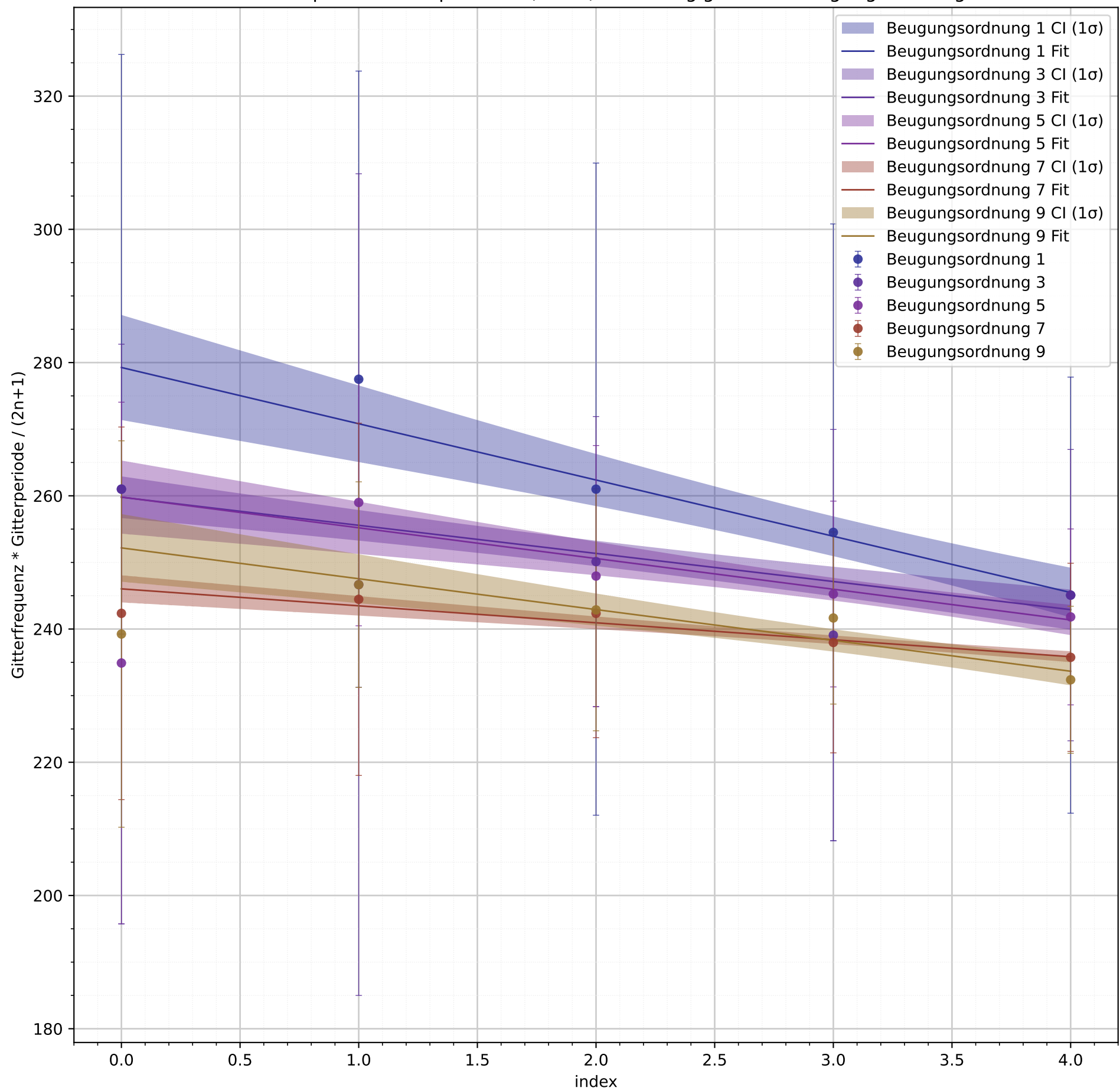
Gitterfrequenz * Gitterperiode / (2n+1) in Abhängigkeit der Beugungsordnung
