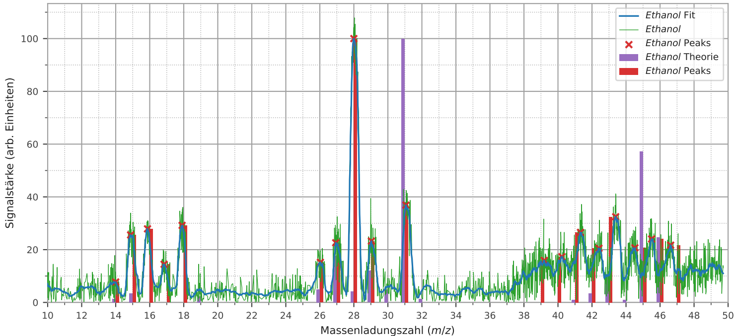
Signalstärke von Ethanol 1 im Vergleich zur Theorie
