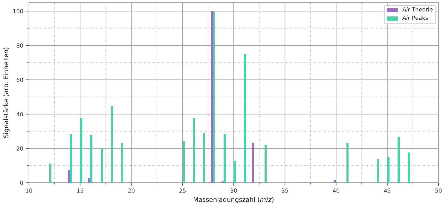
Massenspektrum von Air 1 im Vergleich zur Theorie
