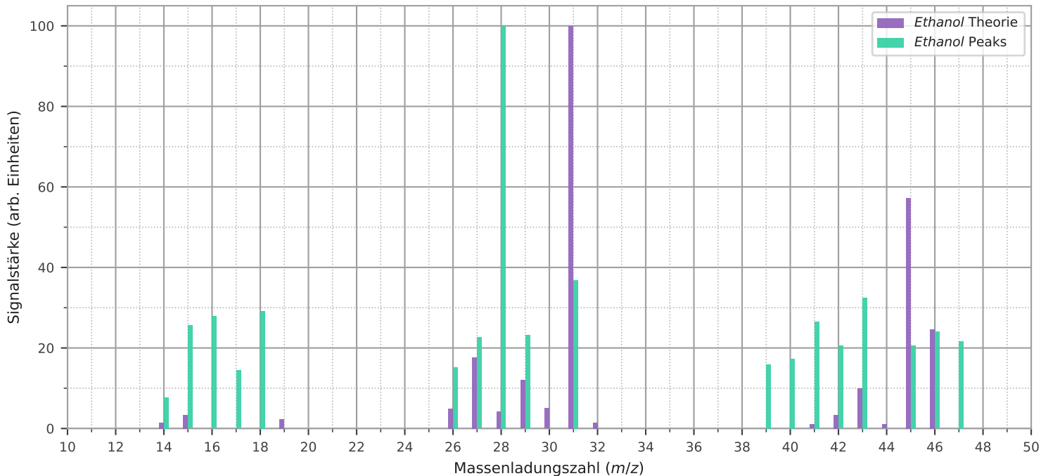
Massenspektrum von Ethanol 1 im Vergleich zur Theorie
