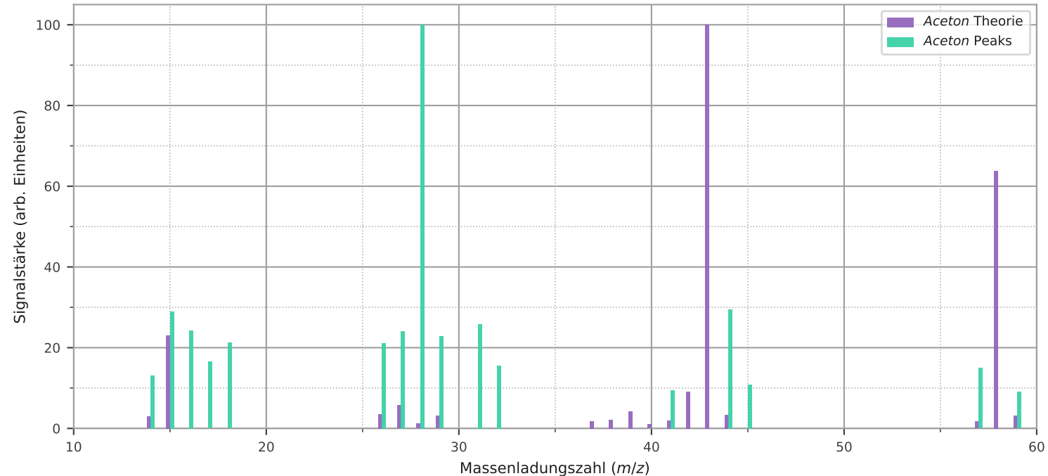
Massenspektrum von Aceton 2 im Vergleich zur Theorie
