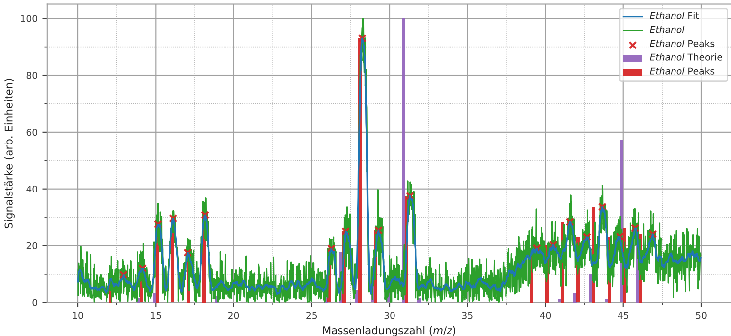
Signalstärke von Ethanol 1 im Vergleich zur Theorie
