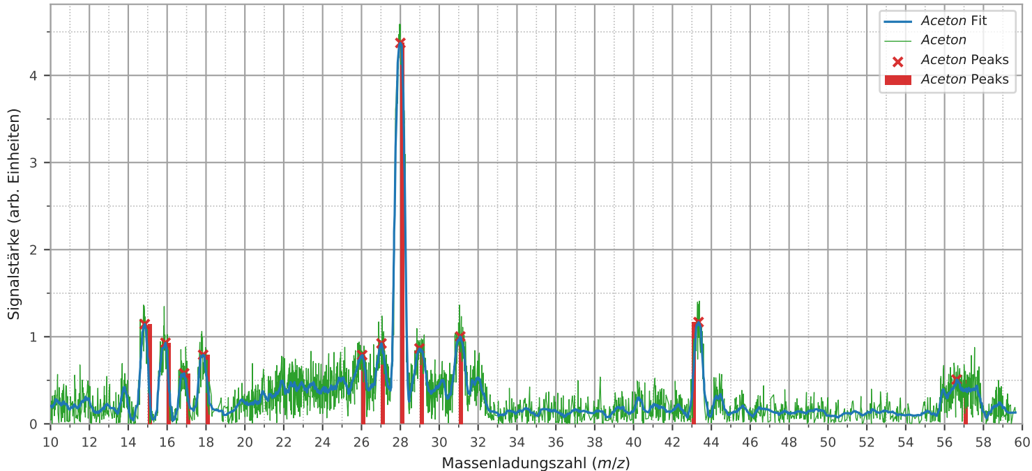
Signalstärke von Aceton 2 und gefundene Peaks
