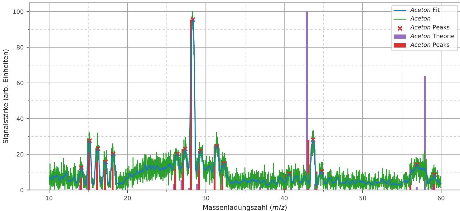
Signalstärke von Aceton 2 im Vergleich zur Theorie
