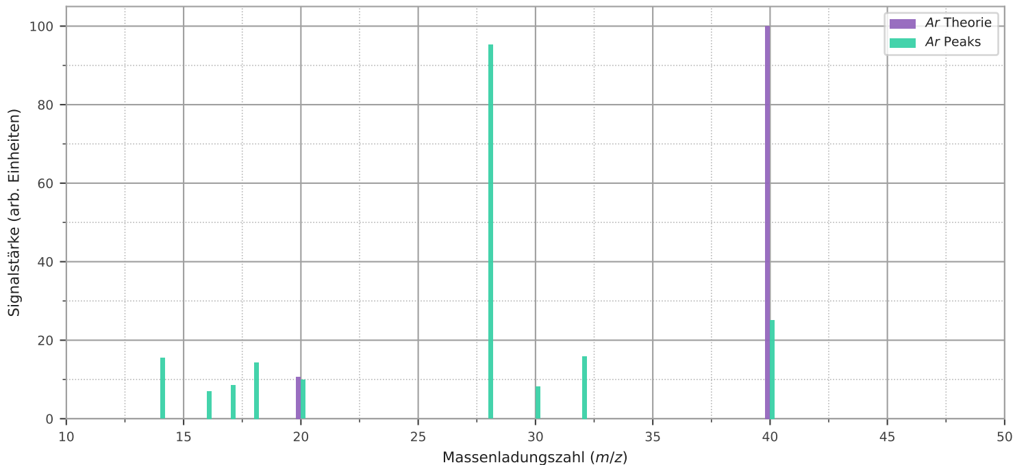
Massenspektrum von Ar 2 im Vergleich zur Theorie
