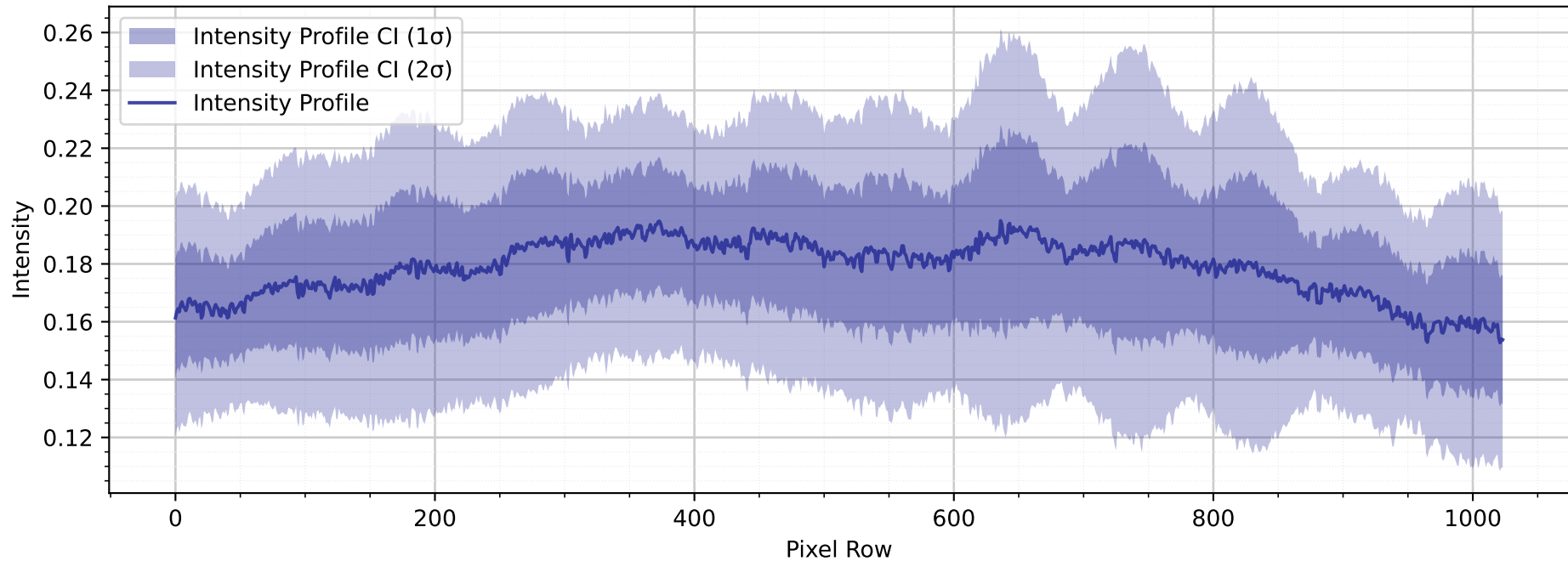
Intensitätsprofil mit Beugungsordnung a3_G4
