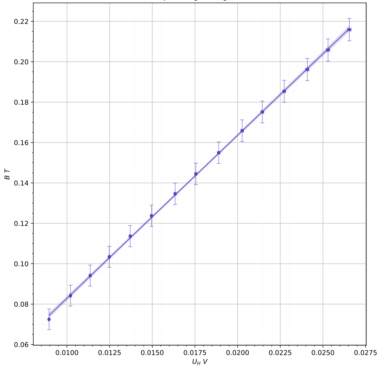
Hallspannung in Magnetfeld
