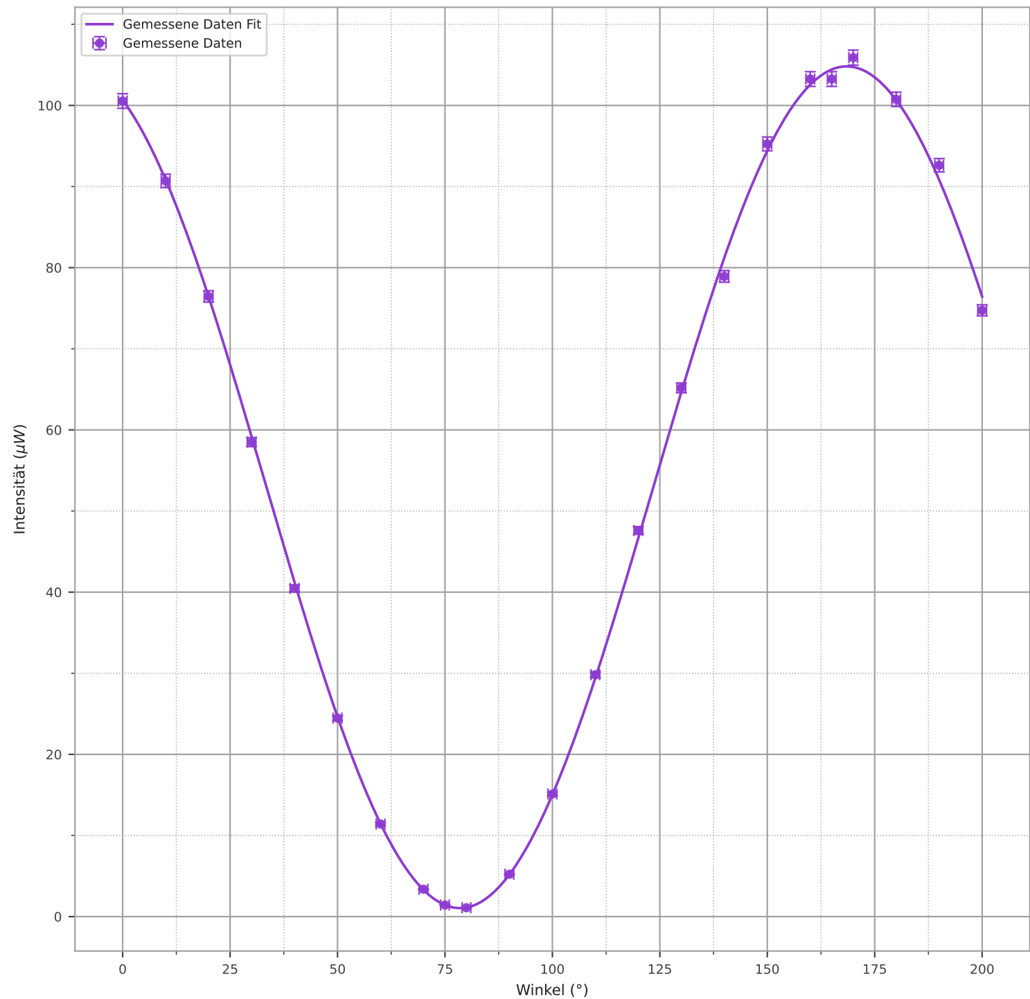
Polarisationskurve des Messlasers
