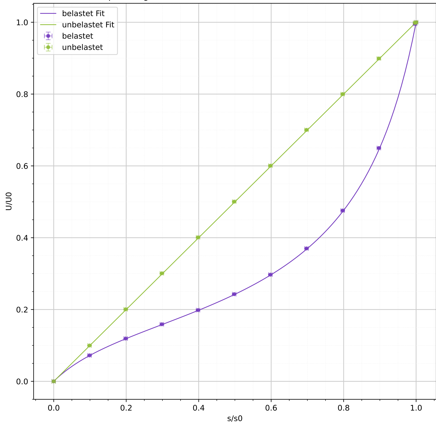
Spannungsverlauf Potentiometer belastet und unbelastet
