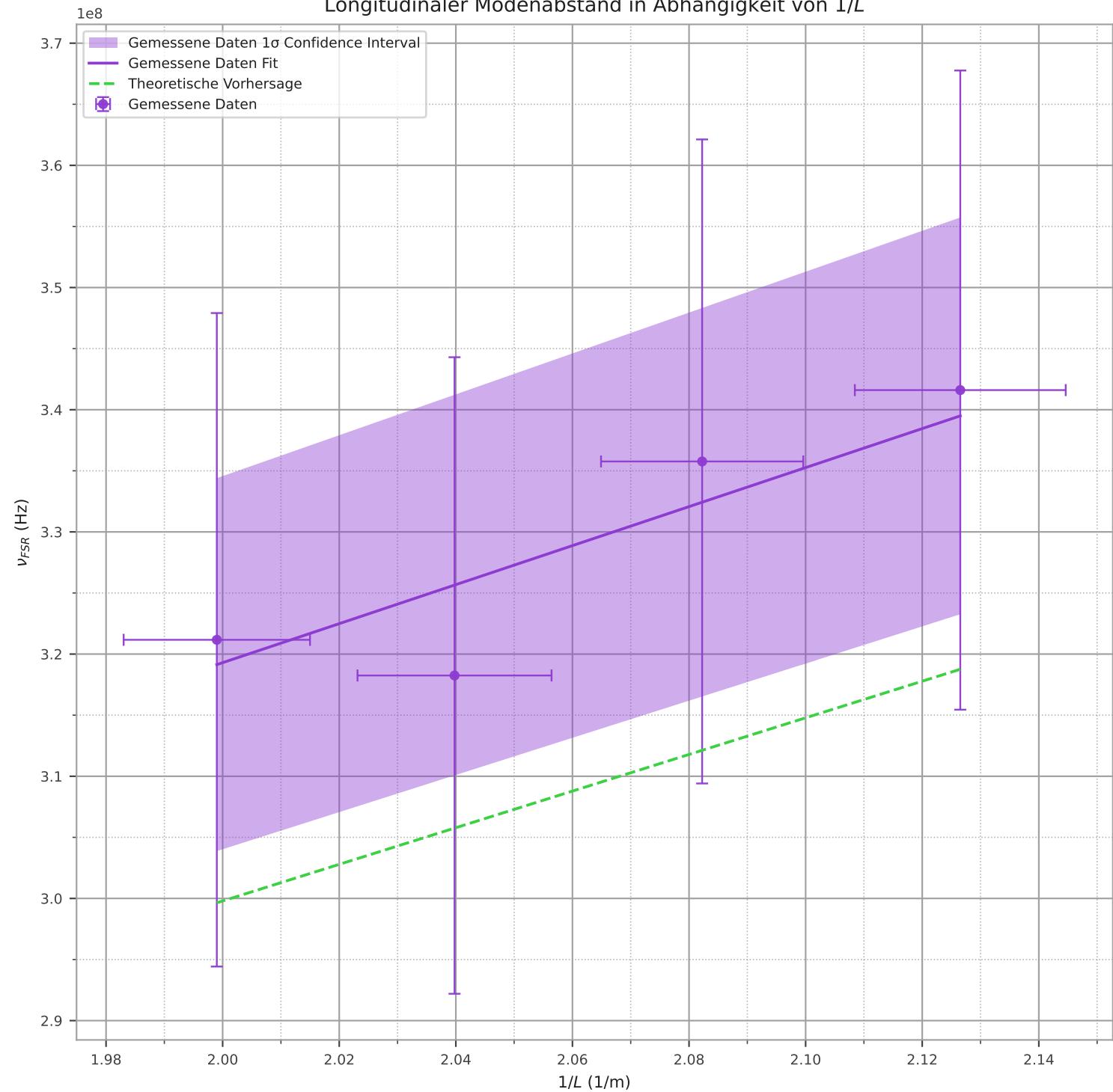
Longitudinaler Modenabstand in Abhängigkeit von 1/L
