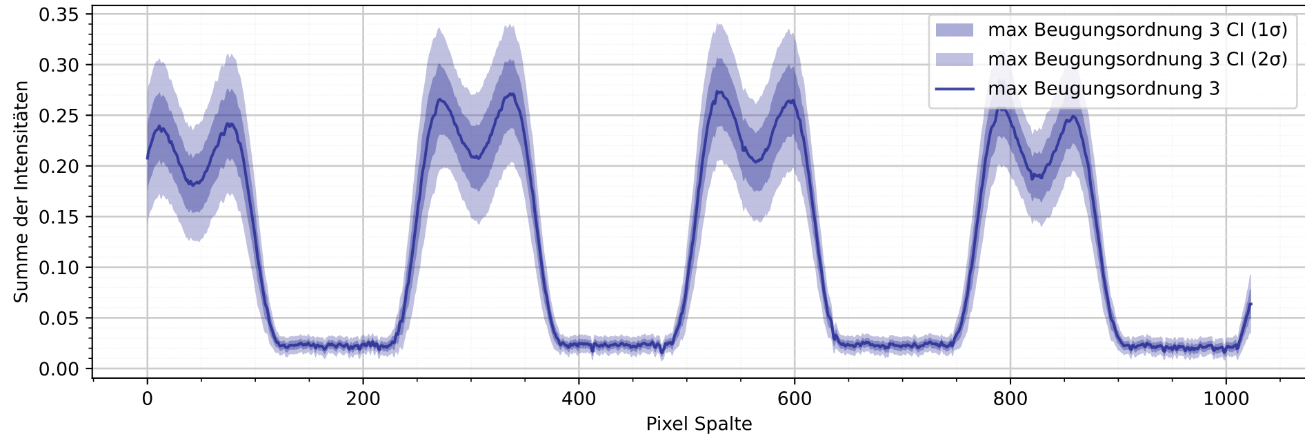
Intensitätsprofil mit Gitter 1 und max. Beugungsordnung 3
