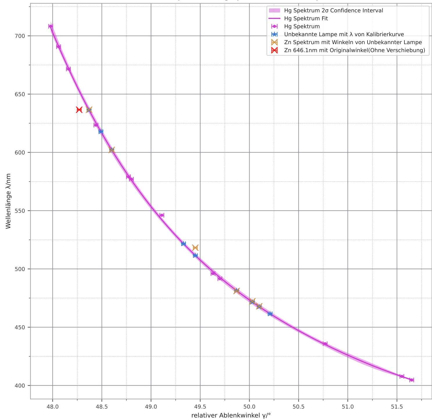
Kalibrierkurve (Spline) des Hg-Spektrums mit Zink-Spektrum
