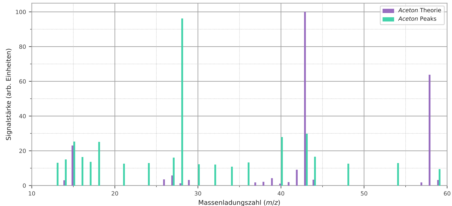
Massenspektrum von Aceton 1 im Vergleich zur Theorie
