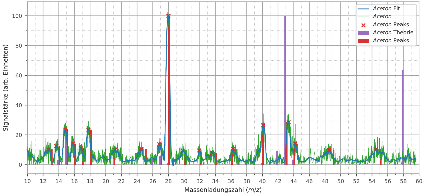
Signalstärke von Aceton 1 im Vergleich zur Theorie
