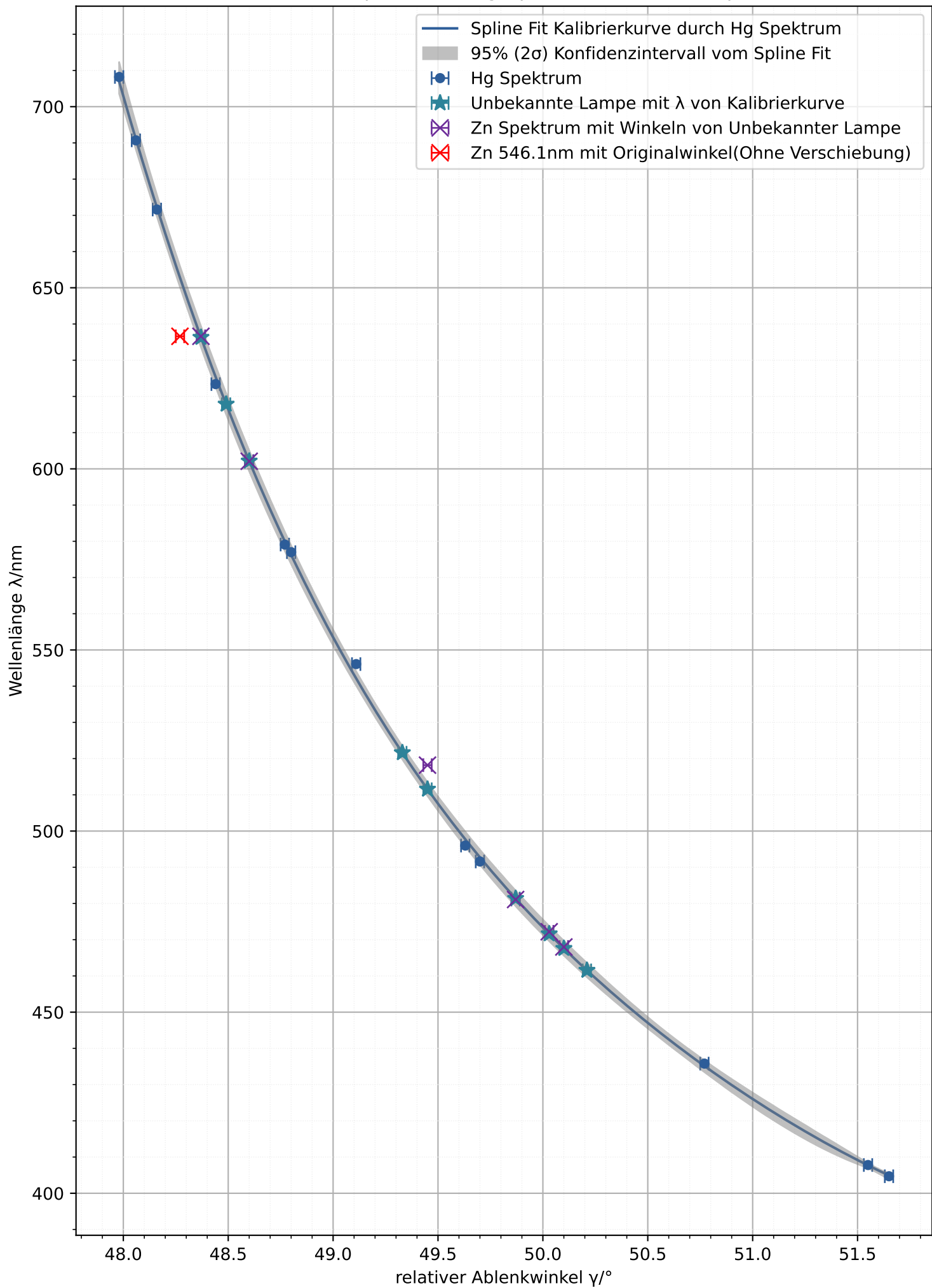
Kalibrierkurve (Spline) des Hg-Spektrums mit Zink-Spektrum
