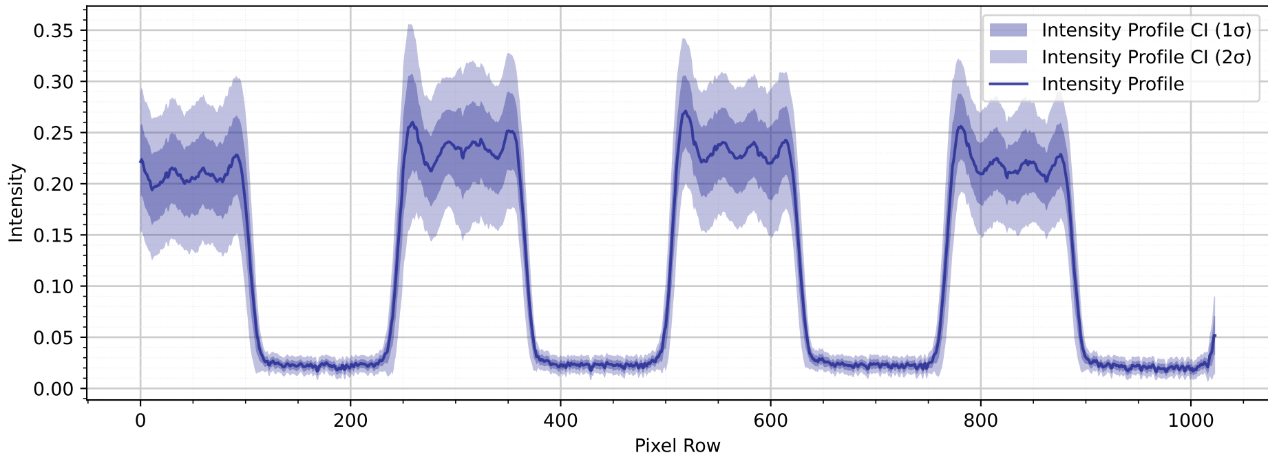
Intensitätsprofil mit Beugungsordnung 7
