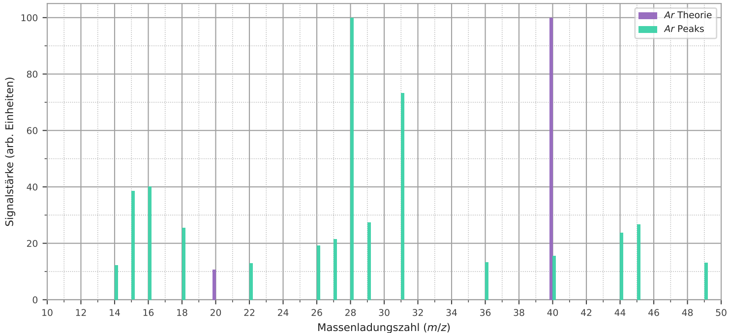
Massenspektrum von Ar 3 im Vergleich zur Theorie
