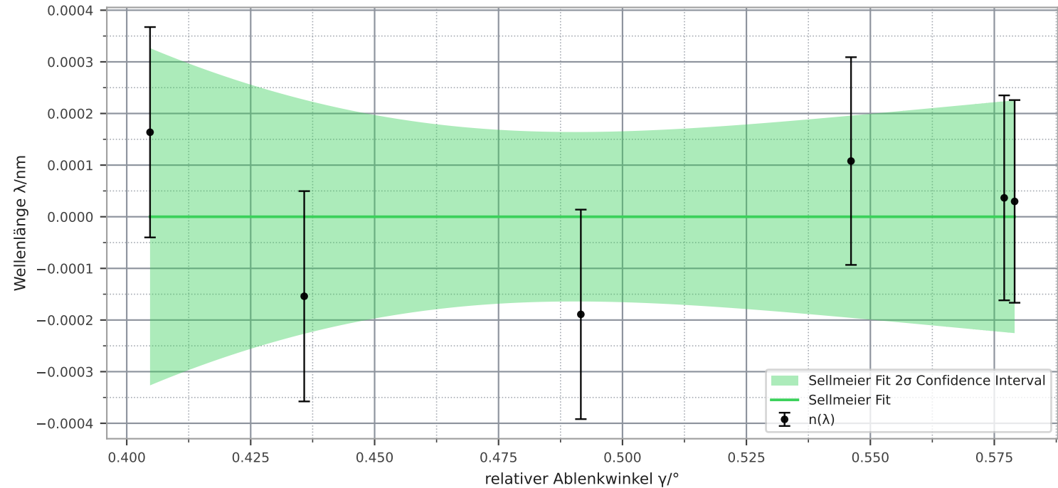
Residuen des Sellmeier Fits
