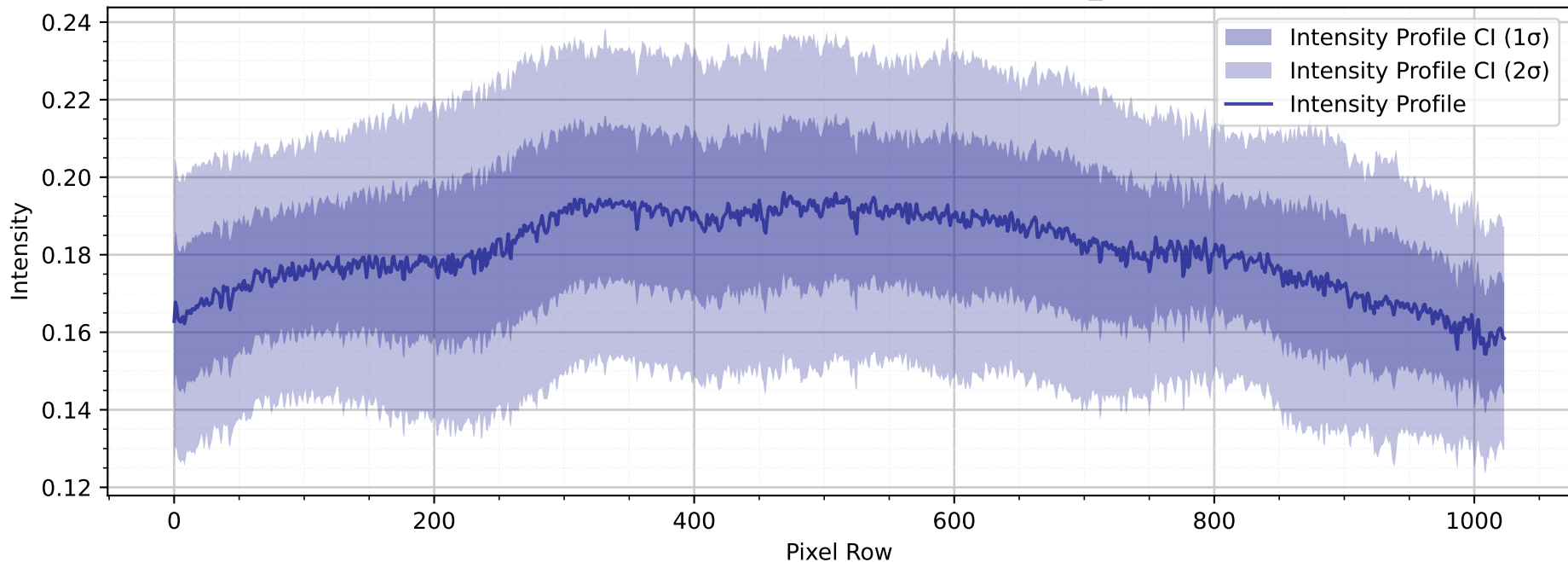
Intensitätsprofil mit Beugungsordnung a3_G5
