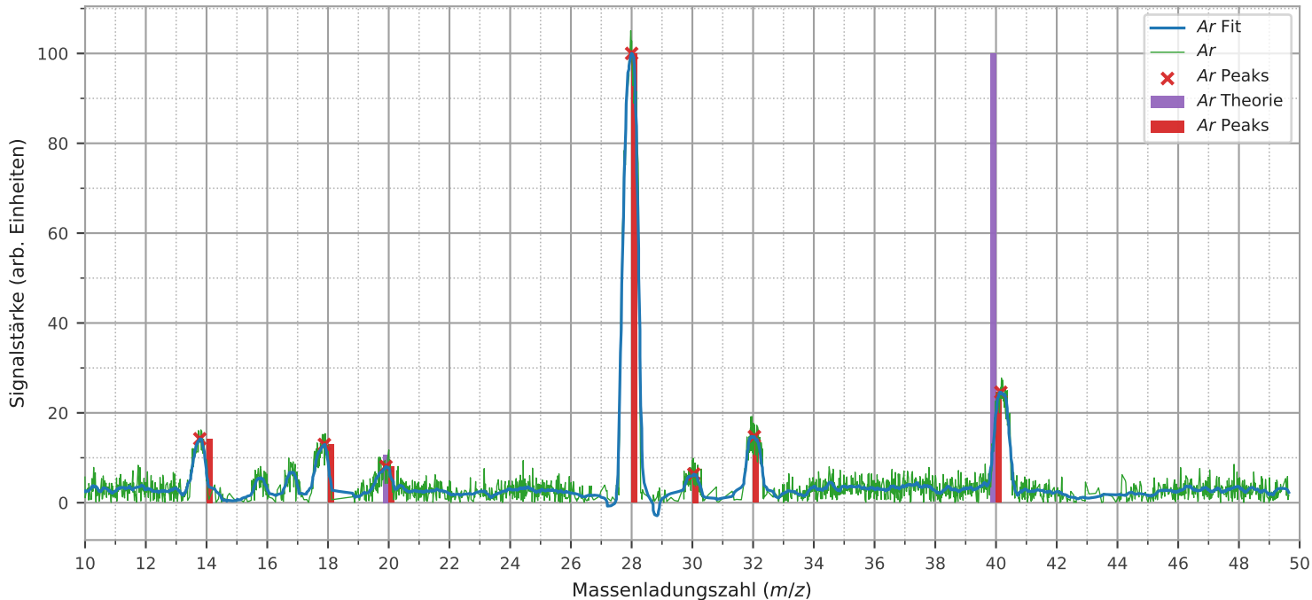
Signalstärke von Ar 2 im Vergleich zur Theorie
