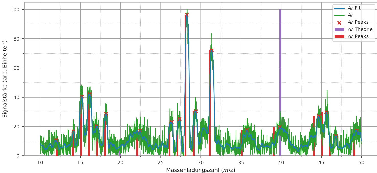
Signalstärke von Ar 3 im Vergleich zur Theorie
