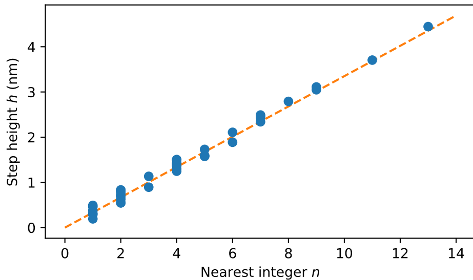
h vs. n \cdot h_0
