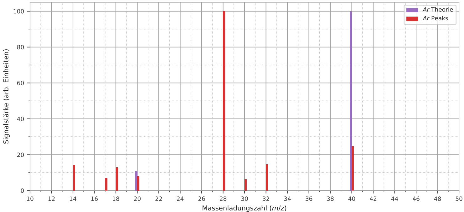
Massenspektrum von Ar 2 im Vergleich zur Theorie
