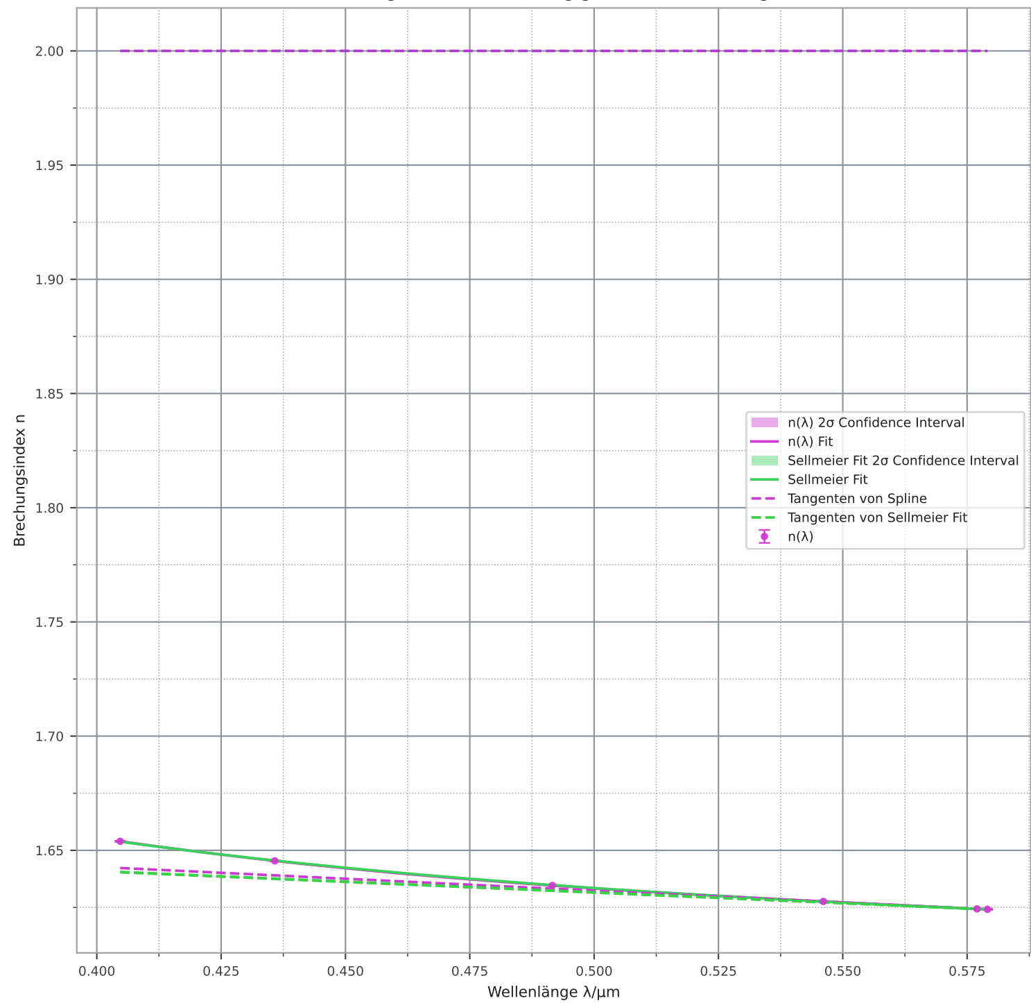
Brechungsindex n in Abhängigkeit der Wellenlänge \lambda
