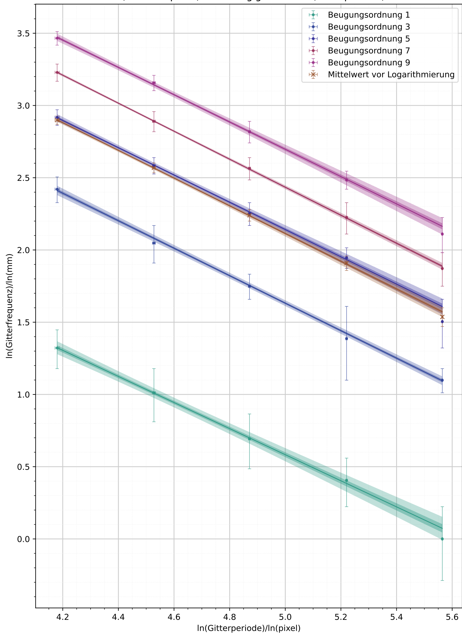
\ln(\text{Gitterfrequenz}) in Abhängigkeit von \ln(\text{Gitterperiode})
