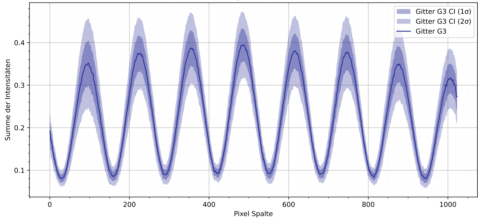
Intensitätsprofil mit Gitter G3
