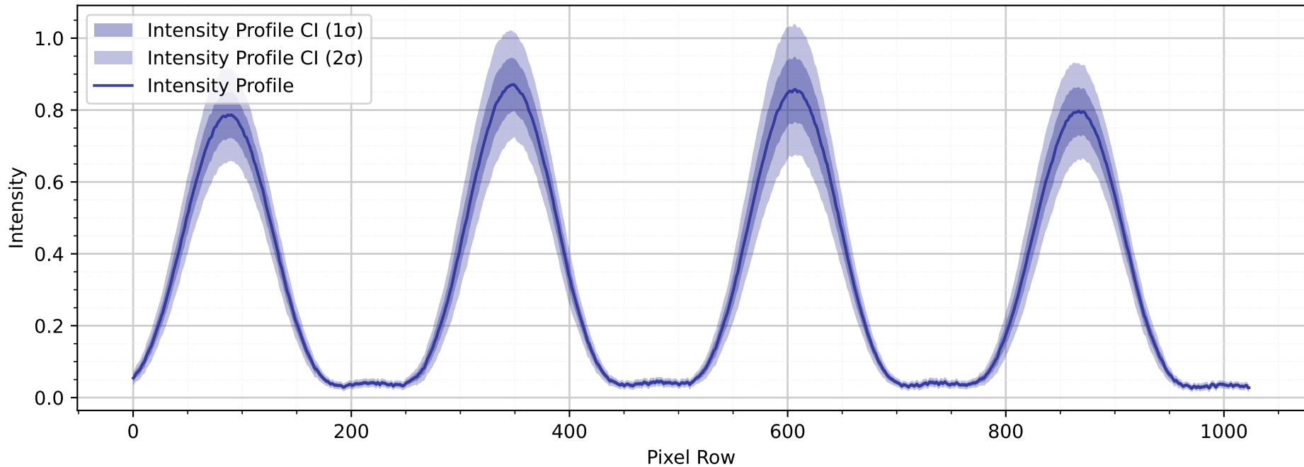
Intensitätsprofil mit Beugungsordnung a3_G1
