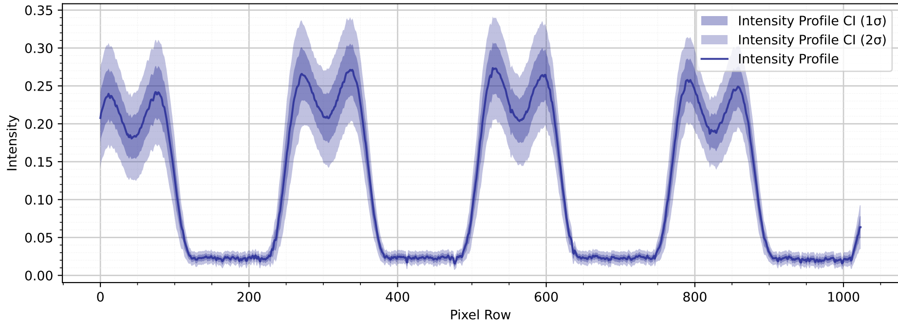
Intensitätsprofil mit Beugungsordnung 3
