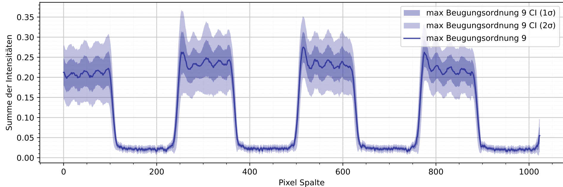
Intensitätsprofil mit Gitter 1 und max. Beugungsordnung 9
