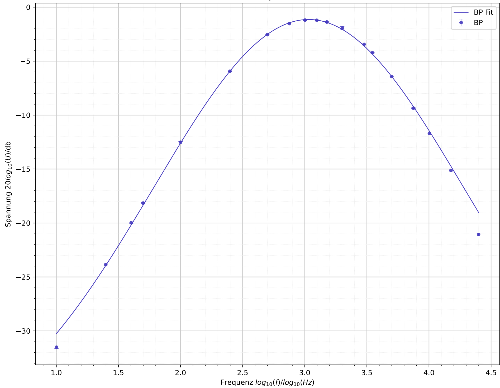
Bandpass
