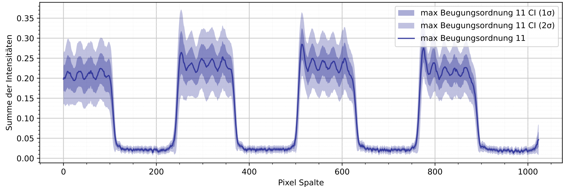
Intensitätsprofil mit Gitter 1 und max. Beugungsordnung 11
