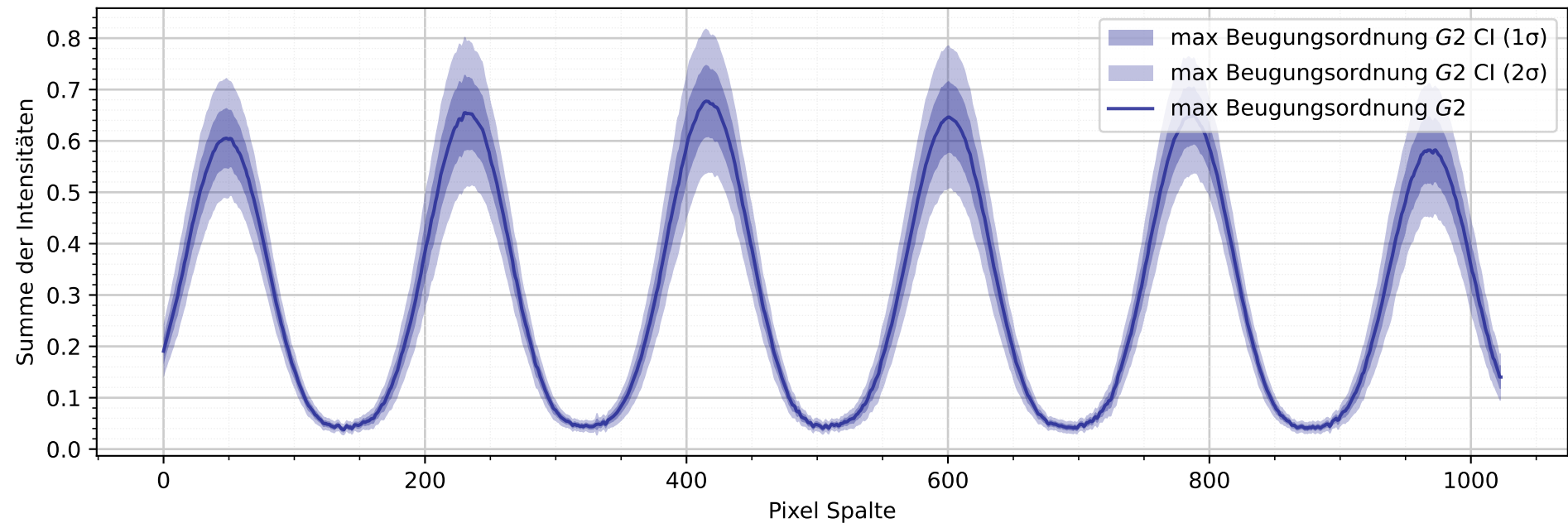
Intensitätsprofil mit Gitter 1 und max. Beugungsordnung G2
