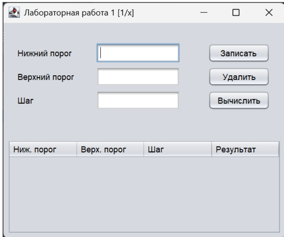
Рисунок 1. – Интерфейс
