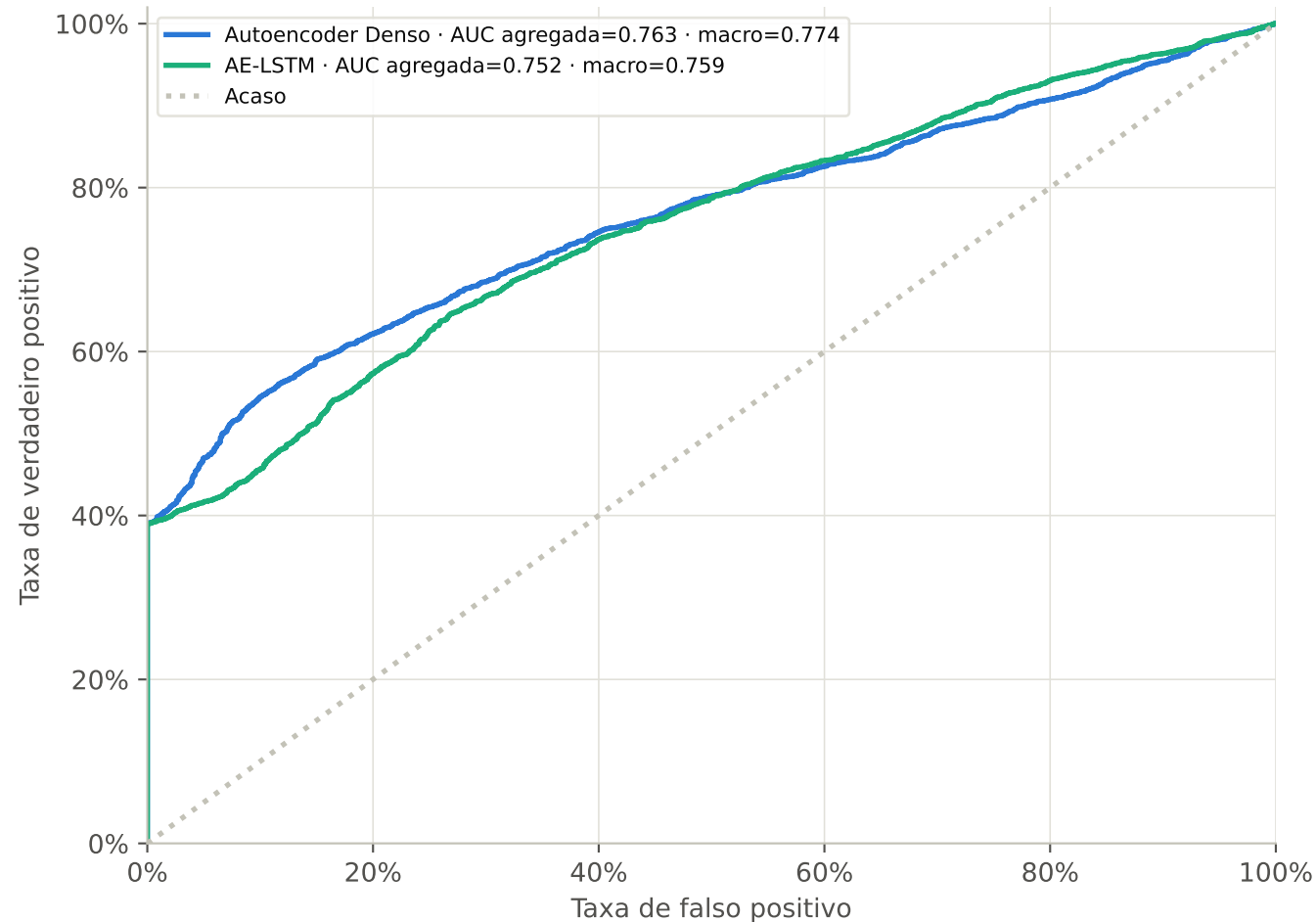
Curva ROC
