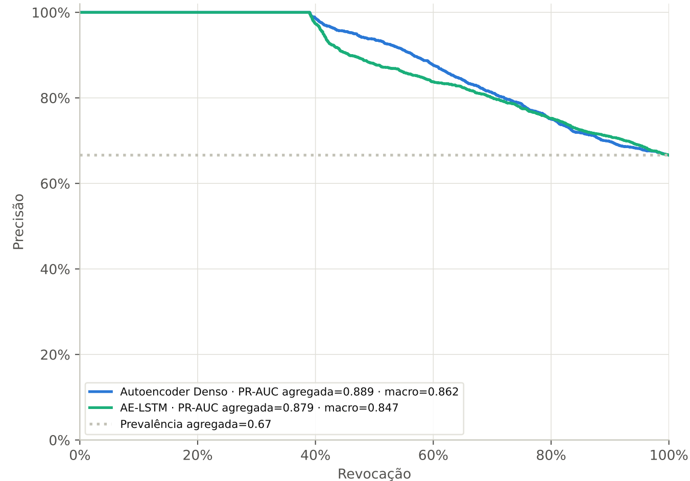
Curva precisão-revocação
