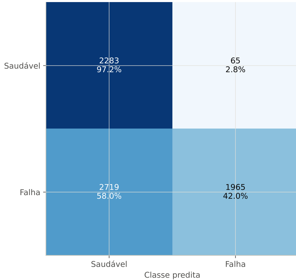
Autoencoder Denso
