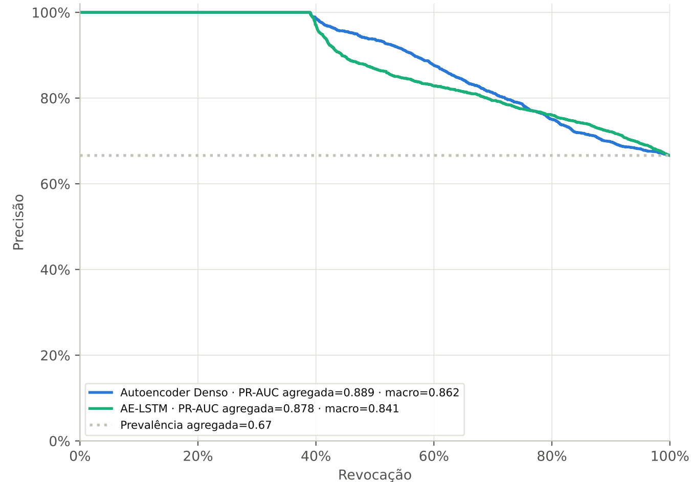
Curva precisão-revoação
