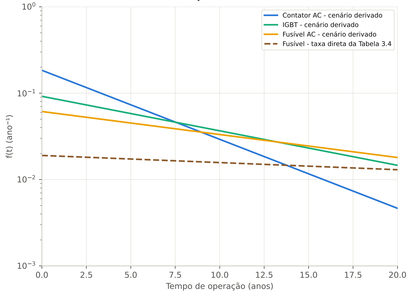
Densidade de probabilidade de falha
