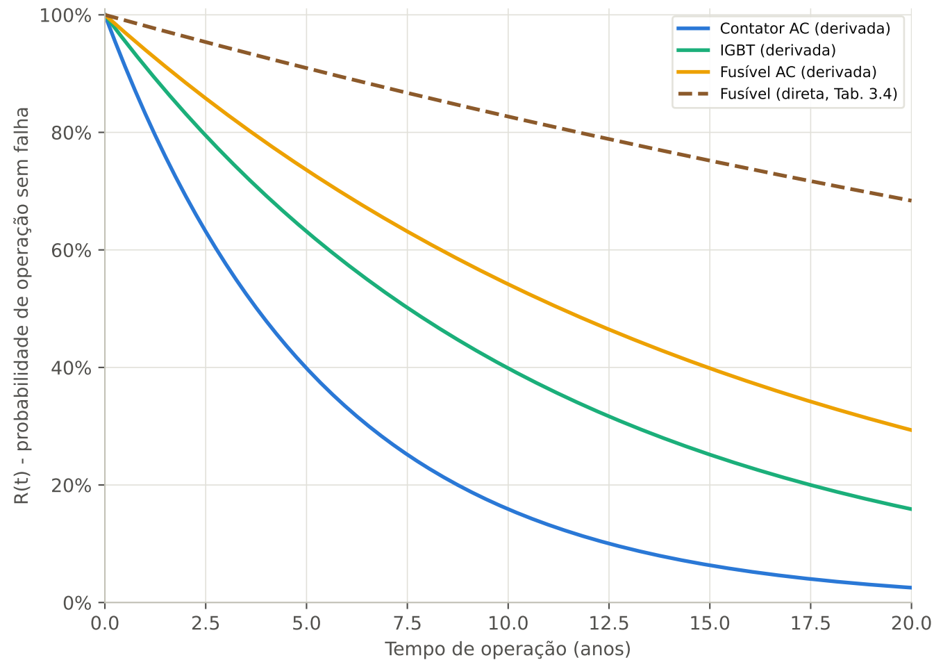
Curva de confiabilidade R(t)
