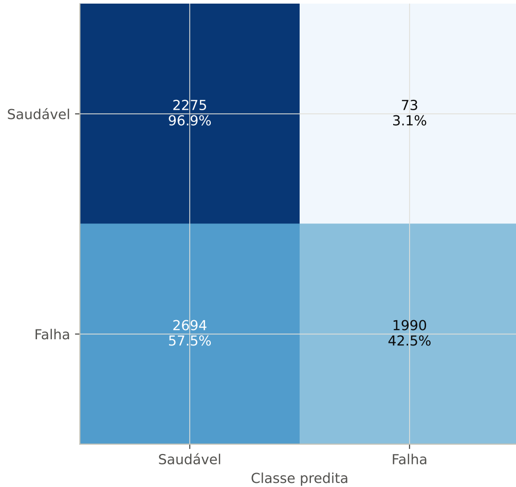
Autoencoder Denso
