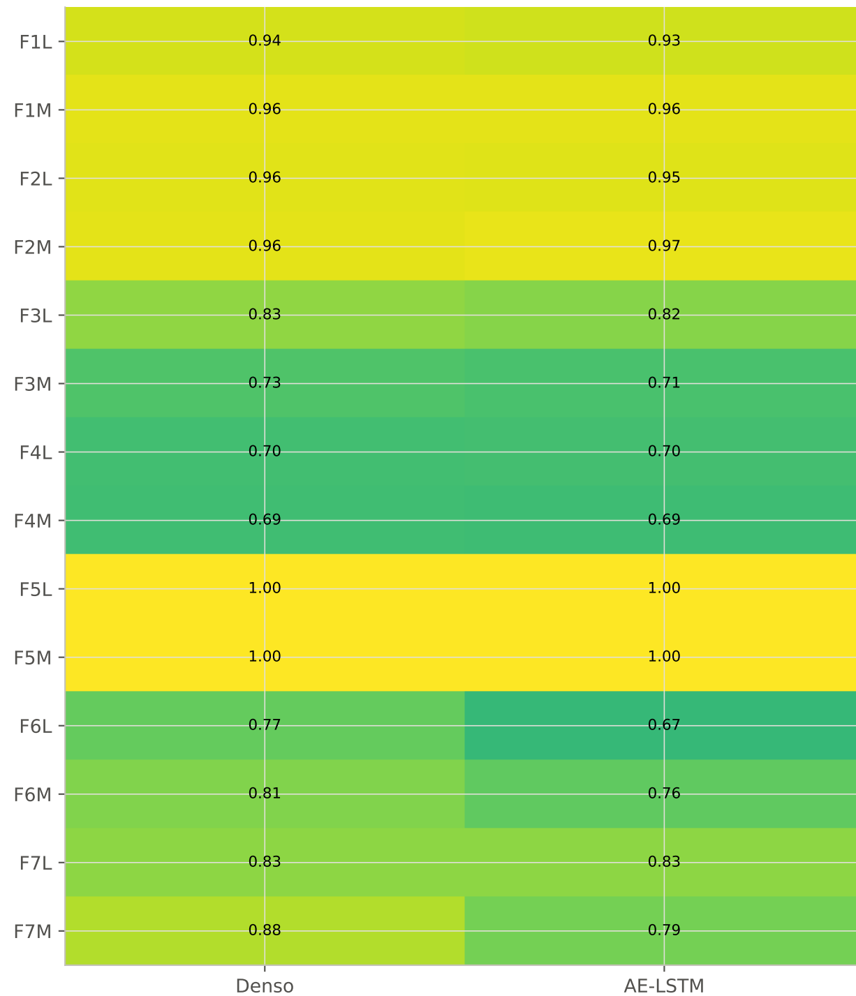
AUC-PR por ensaio
