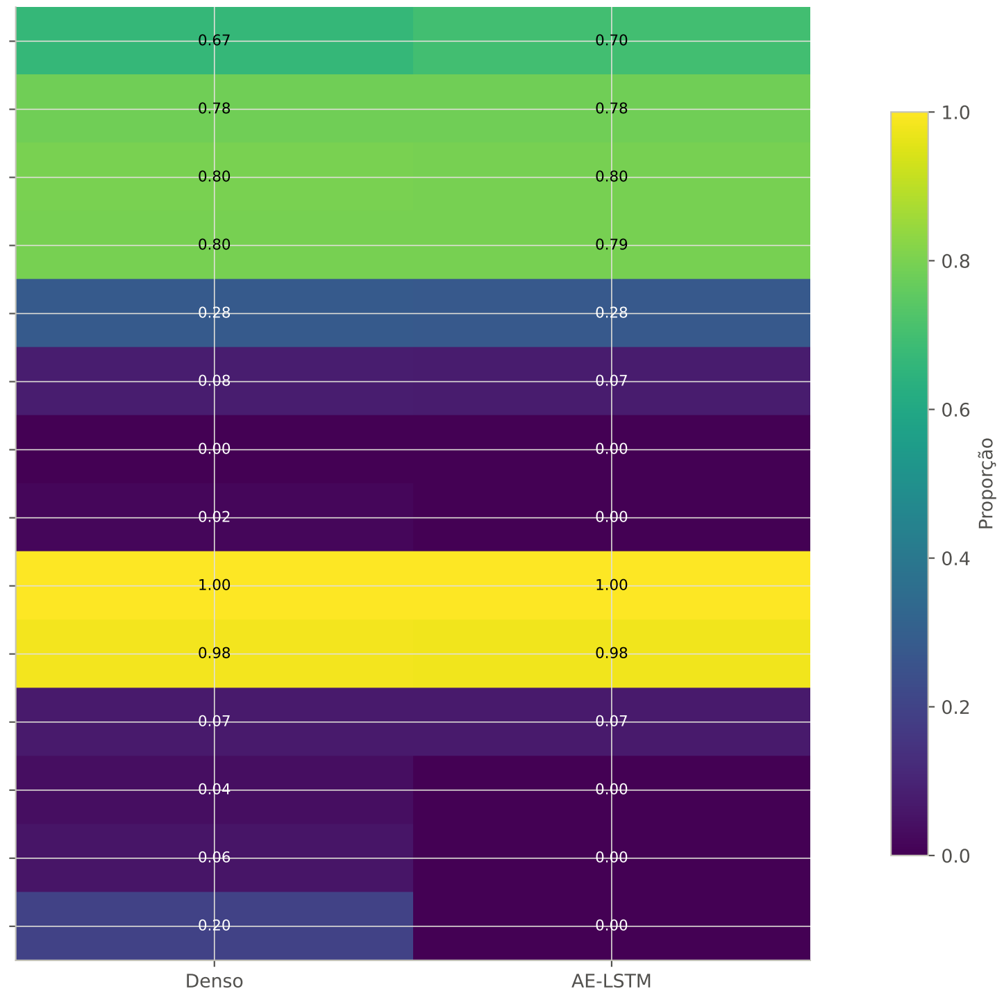
Sensibilidade no limiar p99
