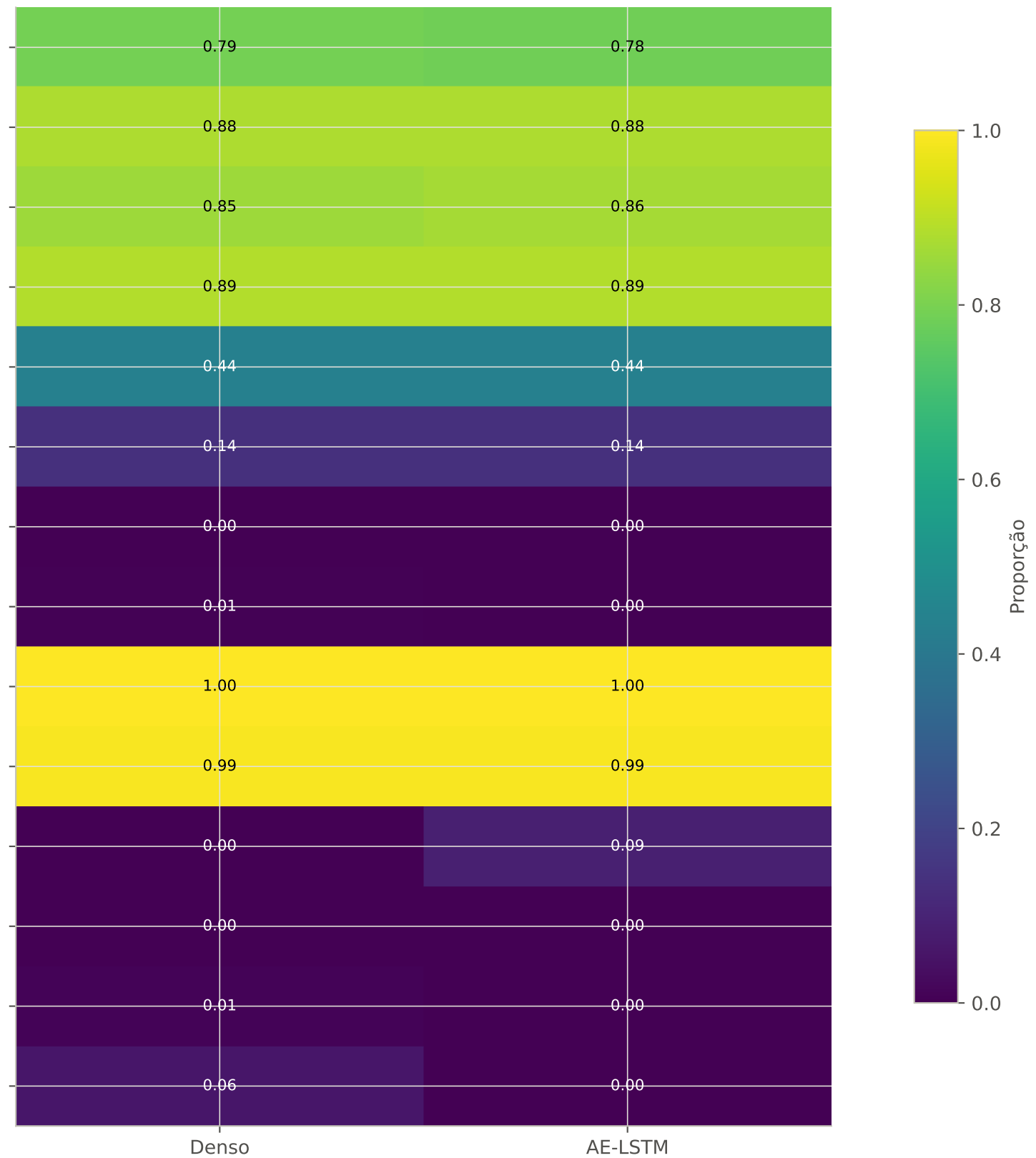
F1 por ensaio no limiar calibrado
