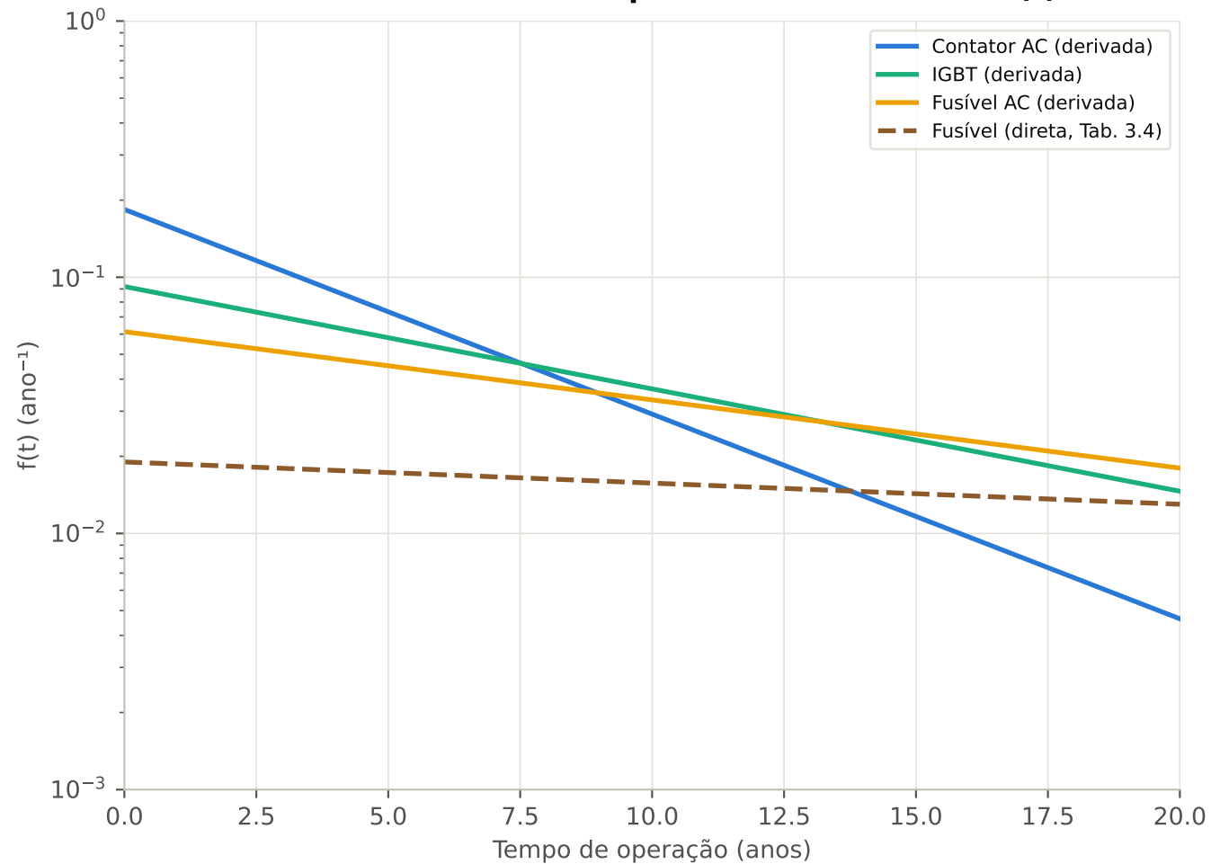
Curva da densidade de probabilidade de falha f(t)
