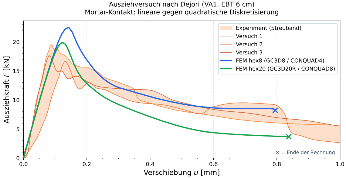
Abbildung 1: Ausziehversuch nach Dejori: Kraft-Weg-Kurven der linearen (hex8) und der quadratischen (hex20) Diskretisierung gegen das Streuband der drei Laborversuche. Beide Rechnungen verwenden dieselbe Gesamt-Auflagerbettung (Abschnitt 15.2). Das Kreuz markiert jeweils das Ende der Rechnung. Erzeugt mit POT_Dejori/plot_comparison.py .
