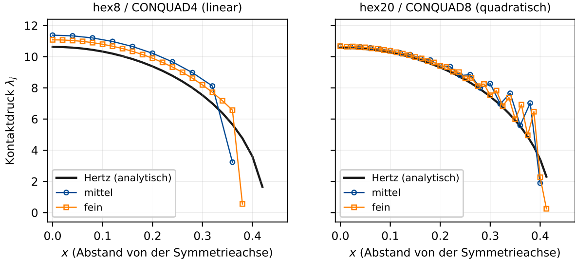
Abbildung 7: Kontaktdruck \lambda_j an den Slave-Knoten gegen die Hertz'sche Halbellipse (61), je Elementtyp für zwei Netzfeinheiten. Links: lineare Elemente liefern ein glattes Profil, dessen Maximum aber systematisch zu hoch liegt und mit Verfeinerung sinkt. Rechts: quadratische Elemente treffen das Maximum auf \sim 1\% , zeigen dafür die Knoten-zu-Knoten-Oszillation quadratischer Mortar-Kontaktdrucke, am stärksten am Rand der Kontaktzone. Die eingezeichnete Hertz-Kurve gehört jeweils zur feinen Variante; p_0 hängt über P' schwach vom Netz ab. Erzeugt aus Control_Tests/08_hertz/hertz_profile_*.csv .
