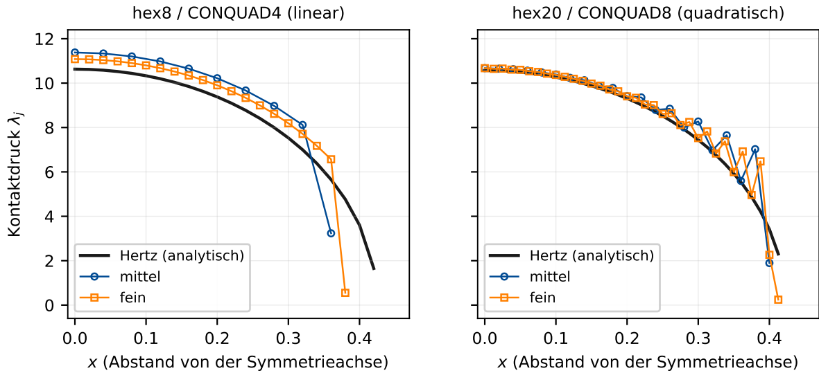
Abbildung 7: Kontaktdruck \lambda_j an den Slave-Knoten gegen die Hertz'sche Halbellipse (66), je Elementtyp für zwei Netzfeinheiten. Links: lineare Elemente liefern ein glattes Profil, dessen Maximum aber systematisch zu hoch liegt und mit Verfeinerung sinkt. Rechts: quadratische Elemente treffen das Maximum auf \sim 1\% , zeigen dafür die Knoten-zu-Knoten-Oszillation quadratischer Mortar-Kontaktdrucke, am stärksten am Rand der Kontaktzone. Die eingezeichnete Hertz-Kurve gehört jeweils zur feinen Variante; p_0 hängt über P' schwach vom Netz ab. Erzeugt aus Control_Tests/08_hertz/hertz_profile_*.csv .
