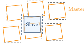
Abbildung 3: Nachbarsuche. Jede Master-Facette erhält eine achsparallele Hüllbox (grau gestrichelt), die in einem binären Baum organisiert wird. Die Abfragebox der Slave-Facette (blau gestrichelt) liefert die Kandidaten; nur für diese wird anschließend die exakte Verschneidung durchgeführt.
