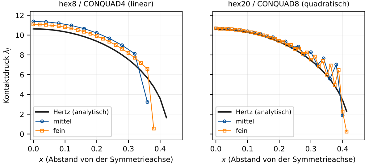
Abbildung 7: Kontaktdruck \lambda_j an den Slave-Knoten gegen die Hertz'sche Halbellipse (59), je Elementtyp für zwei Netzfeinheiten. Links : lineare Elemente liefern ein glattes Profil, dessen Maximum aber systematisch zu hoch liegt und mit Verfeinerung sinkt. Rechts : quadratische Elemente treffen das Maximum auf \sim 1\% , zeigen dafür die Knoten-zu-Knoten-Oszillation quadratischer Mortar-Kontaktdrücke, am stärksten am Rand der Kontaktzone. Die eingezeichnete Hertz-Kurve gehört jeweils zur feinen Variante; p_0 hängt über P' schwach vom Netz ab. Erzeugt aus Control_Tests/08_hertz/hertz_profile_*.csv .
