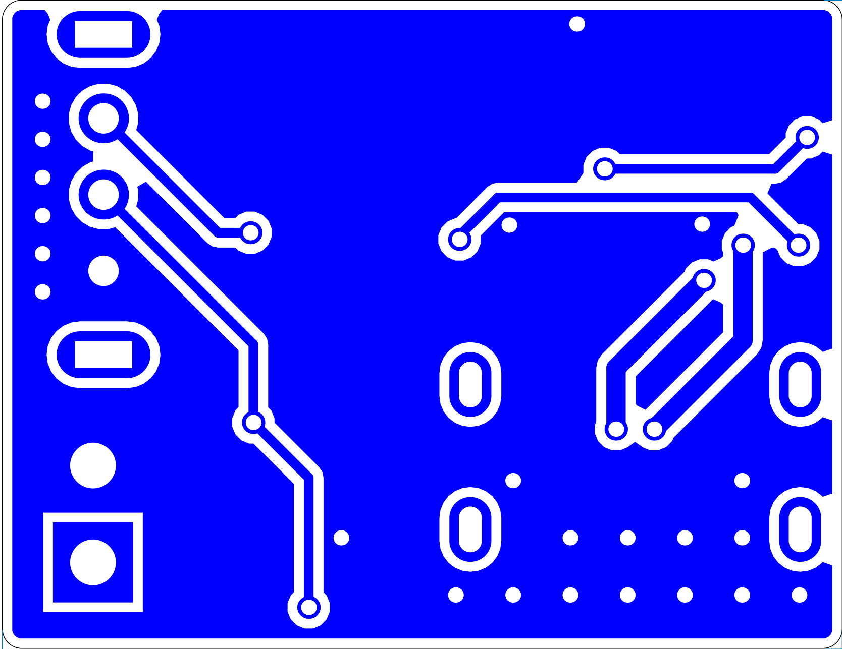
Bottom Layer (Scale 10:1)
