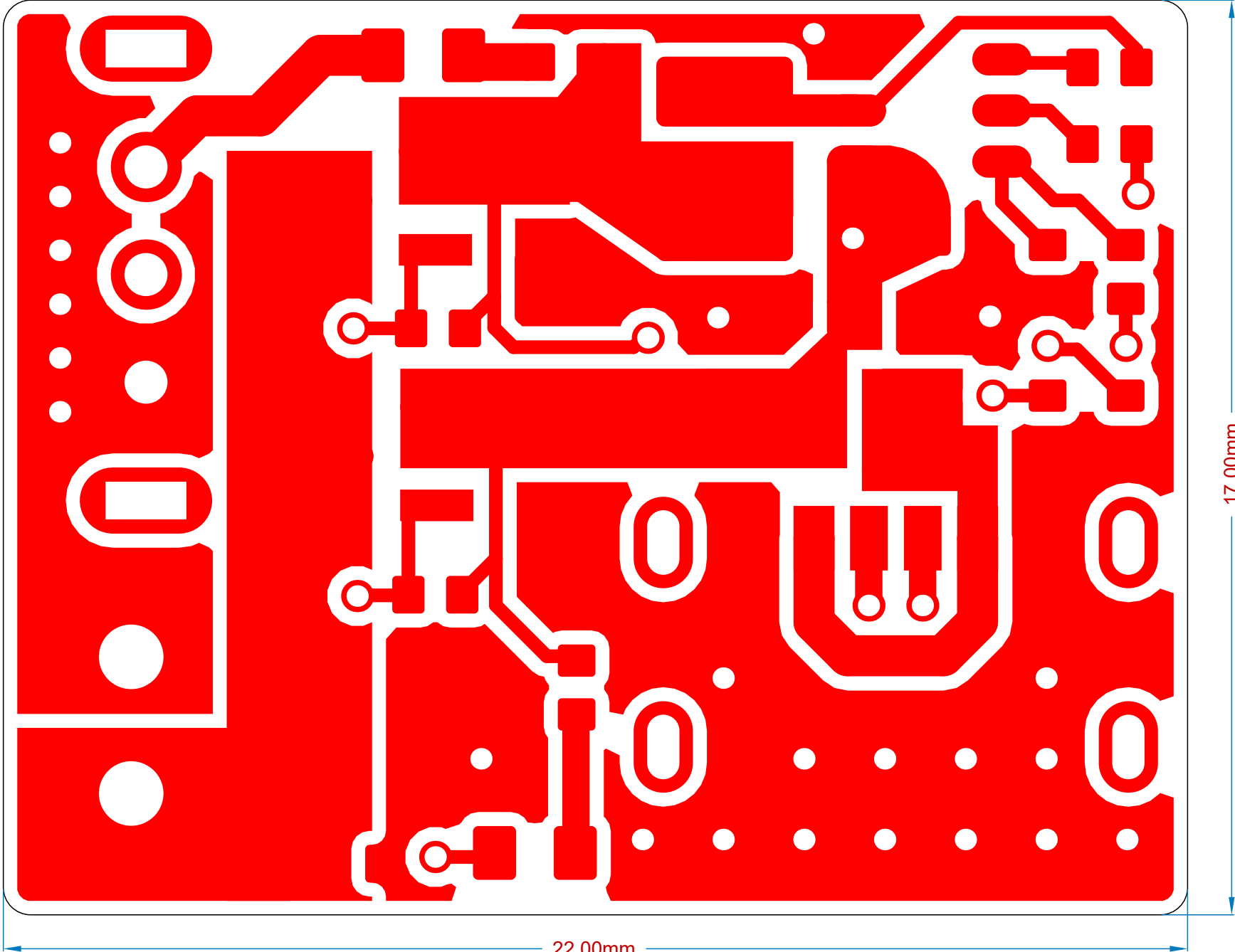
Top Layer (Scale 10:1)
