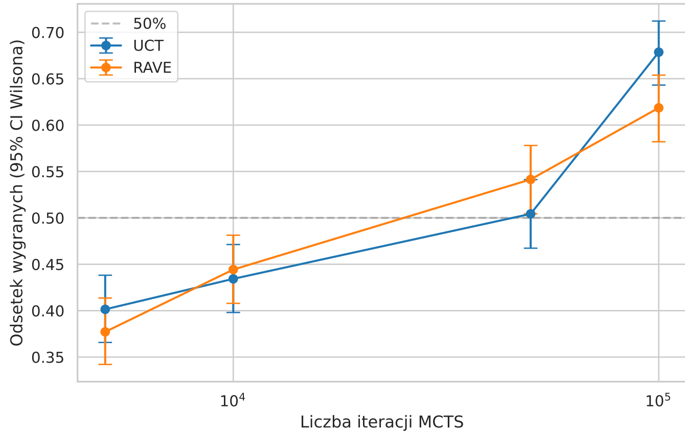
H1: RAVE vs UCT — skalowanie z budżetem iteracji
