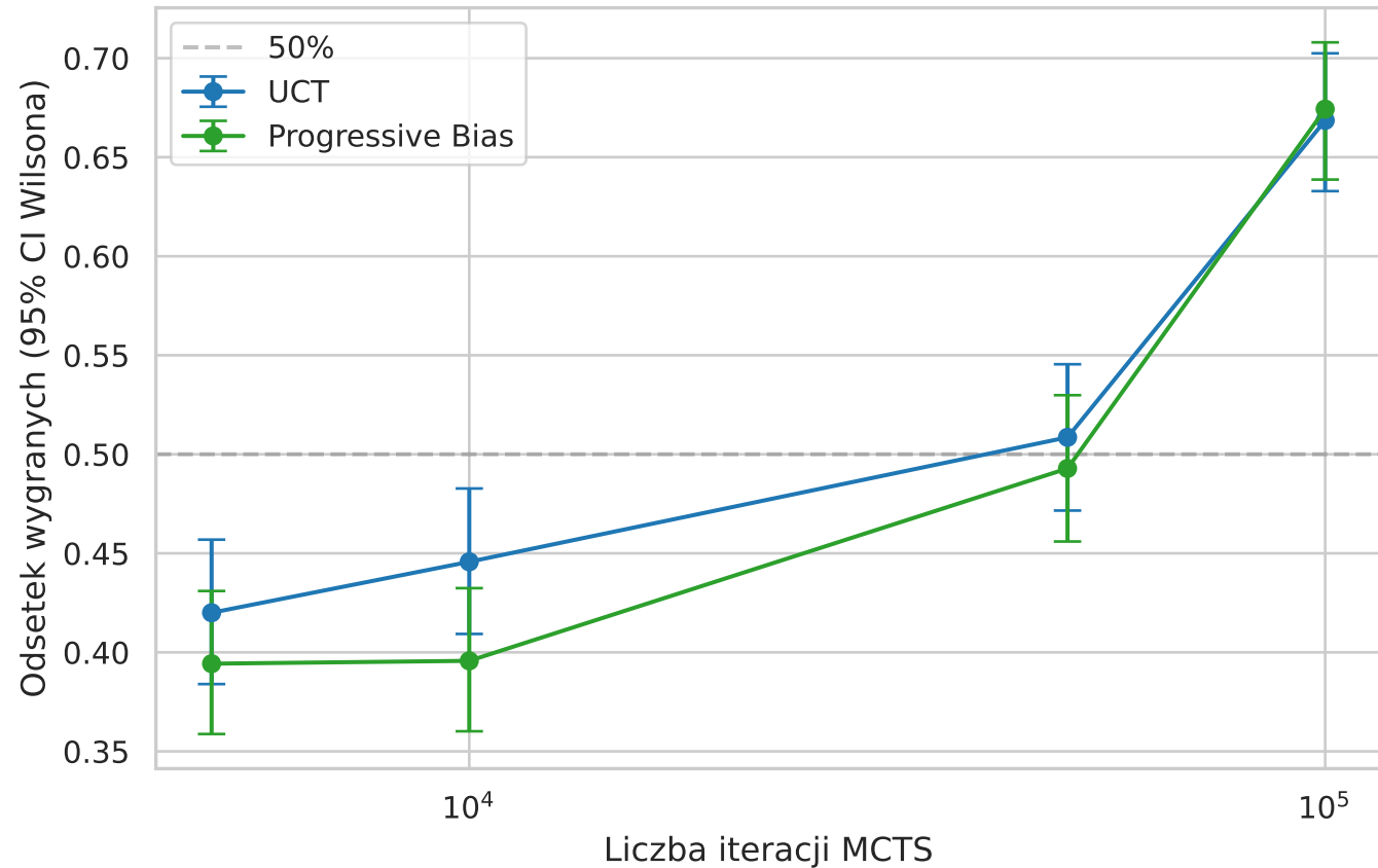
H2: Progressive Bias vs UCT — skalowanie z budżetem iteracji
