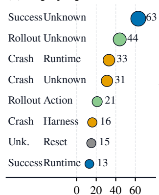
(d) Top symptom-factor links
