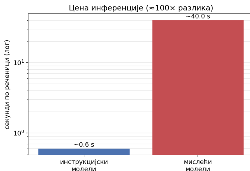
Слика 16: Просечна цена инференције по реченици
