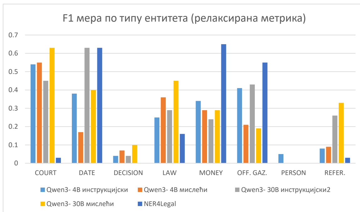
Слика 20: Графички приказ F1 мере по типу ентитета (релаксирана метрика)
