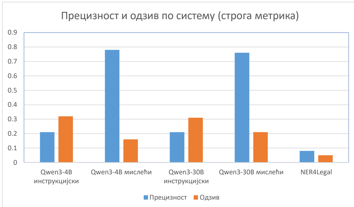
Слика 19: Графички приказ прецизности и одзива по систему (строга метрика)
