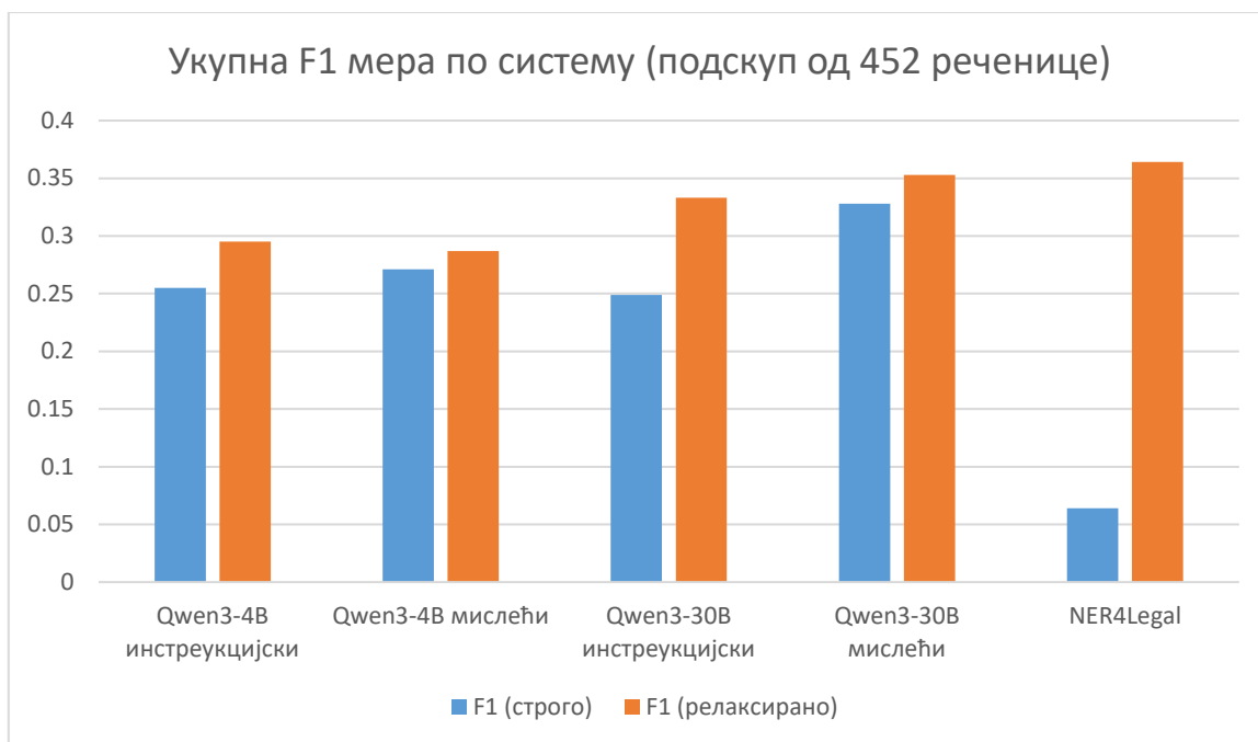
Слика 18: Графички приказ F1 мера по систему
