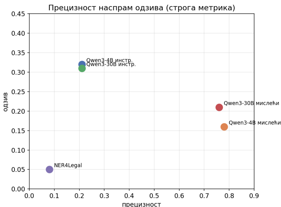
Слика 21. Однос прецизности и одзива по систему
