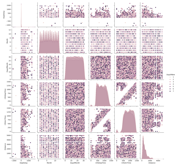
Figura 1.1: Pair plot para visualizar la mayoría de los datos comparados entre sí. No se graficaron los 10 millones de puntos por el tiempo de computo requerido, sólo se graficaron un millón. Se añadió también que, para cada punto, se etiquetara por su el día de la semana ( DayOfWeek ) para intentar de visualizar alguna zona de interes así como la distribución de los mismos.
