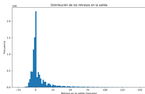
Figura 1.3: Histograma con retrasos en los vuelos. NOTA: La escala de este histograma se ha recordado de -25 a 150. Esto debido a que los outliers (tanto positivos como negativos) son tan grandes y muy pocos que reducen mucho la visibilidad de la gran mayoría de los datos.
